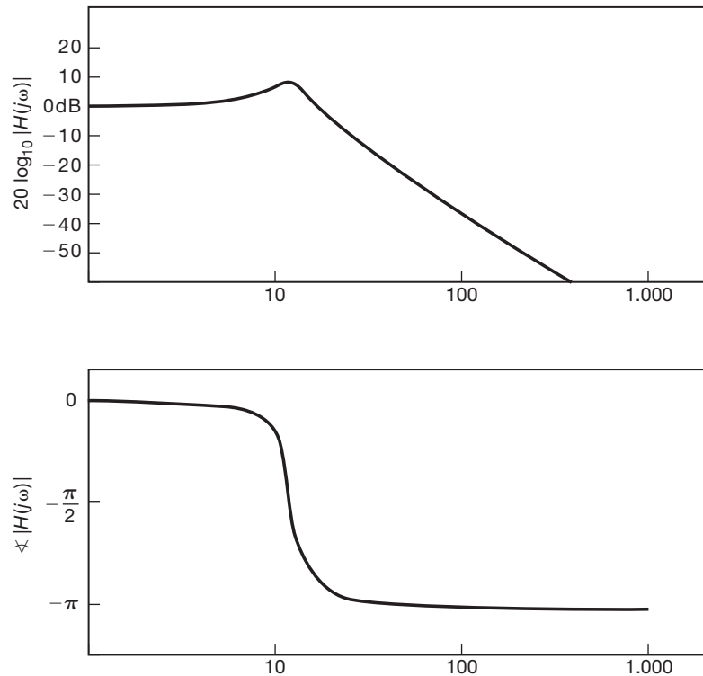
Figura 6.8 Um diagrama de Bode típico. (Observe que \omega é apresentado graficamente usando-se uma escala logarítmica.)
