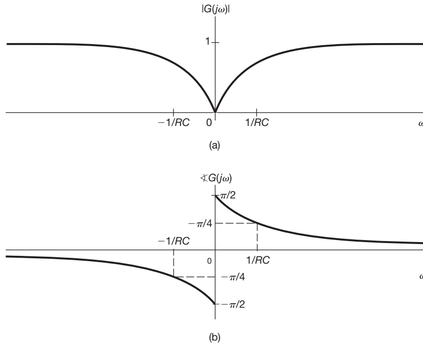
Figura 3.32 Gráficos de (a) magnitude e (b) fase da resposta em frequência do circuito RC da Figura 3.29 com saída v_f(t) .
