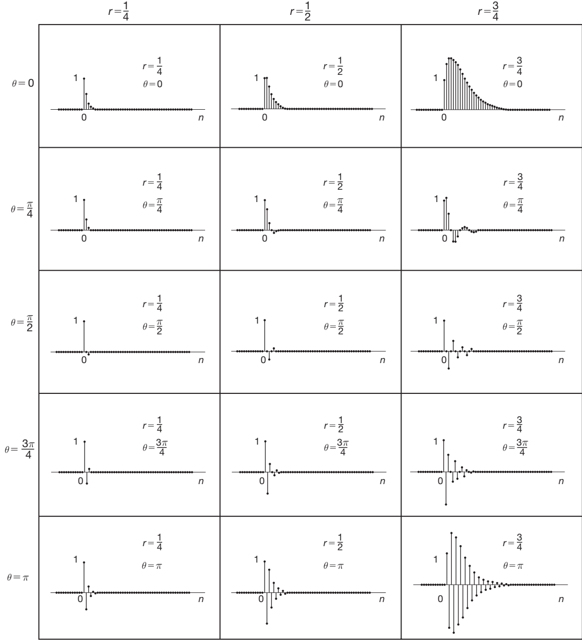
Figura 6.29 Resposta ao impulso do sistema de segunda ordem da Equação 6.57 para diferentes valores de r e \theta .
