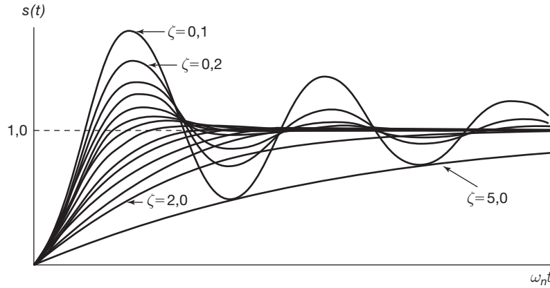
Figura 6.34 Resposta ao degrau do sistema de suspensão de automóvel para diversos valores do fator de amortecimento ( \zeta = 0,1; 0,2; 0,3; 0,4; 0,5; 0,6; 0,7; 0,8; 0,9; 1,0; 1,2; 1,5; 2,0; 5,0 ).
