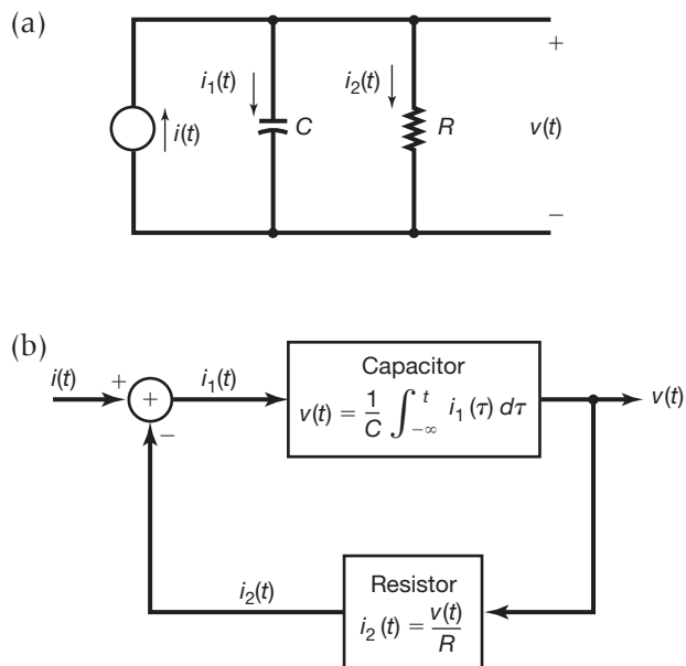
Figura 1.44 (a) Circuito elétrico simples; (b) diagrama de blocos no qual o circuito é representado como a interconexão com realimentação dos dois elementos do circuito.
