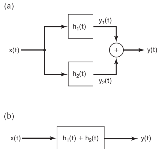
Figura 2.23 Interpretação da propriedade distributiva da convolução para uma interconexão paralela de sistemas LIT.
