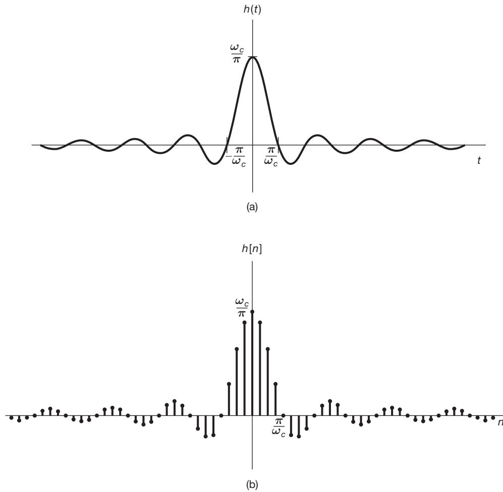
Figura 6.12 (a) A resposta ao impulso do filtro passa-baixas ideal de tempo contínuo da Figura 6.10(a); (b) a resposta ao impulso do filtro passa-baixas ideal de tempo discreto da Figura 6.10(b) com \omega_c = \pi/4 .
