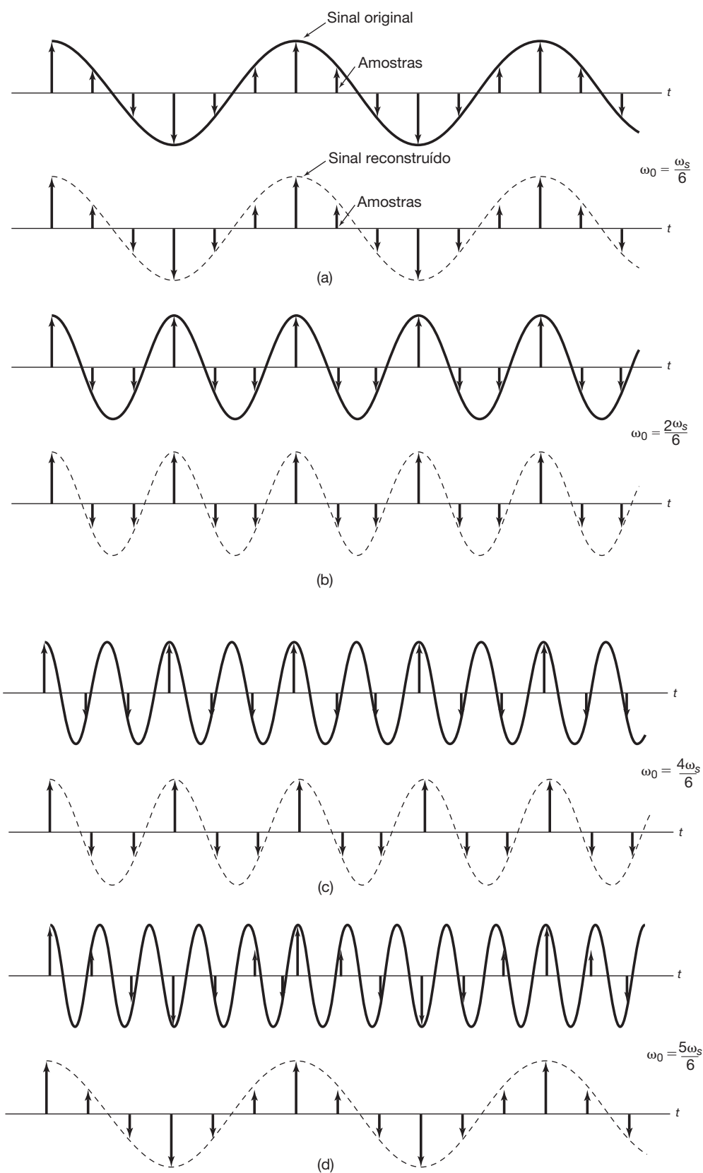
Figura 7.16 Efeito do aliasing sobre um sinal senoidal. Para cada um dos quatro valores de \omega_0 , são ilustrados: o sinal senoidal original (curva sólida), suas amostras e o sinal reconstruído (curva tracejada). (a) \omega_0 = \omega_s/6 ; (b) \omega_0 = 2\omega_s/6 ; (c) \omega_0 = 4\omega_s/6 ; (d) \omega_0 = 5\omega_s/6 . Em (a) e (b) não ocorre aliasing , enquanto em (c) e (d) existe aliasing .
