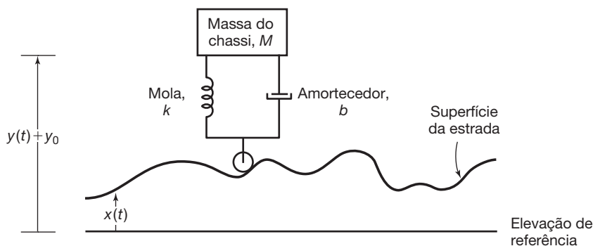
Figura 6.32 Representação diagramática de um sistema de suspensão de automóvel. Aqui, y_0 representa a distância entre o chassi e a superfície da estrada quando o automóvel está em repouso, y(t) + y_0 indica a posição do chassi acima da elevação de referência, e x(t) mostra a elevação da estrada acima da elevação de referência.
