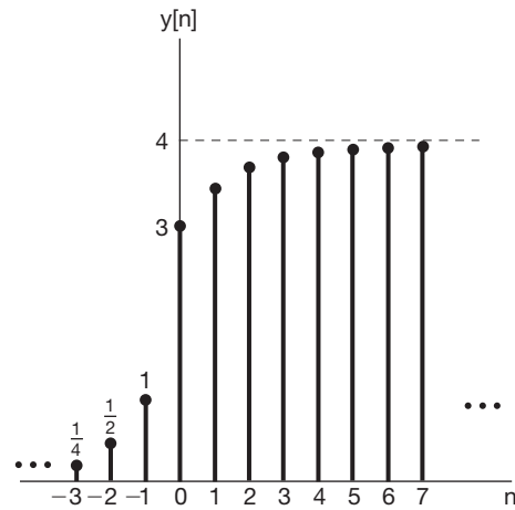
Figura 2.24 Sinal y[n] = x[n] * h[n] para o Exemplo 2.10.
