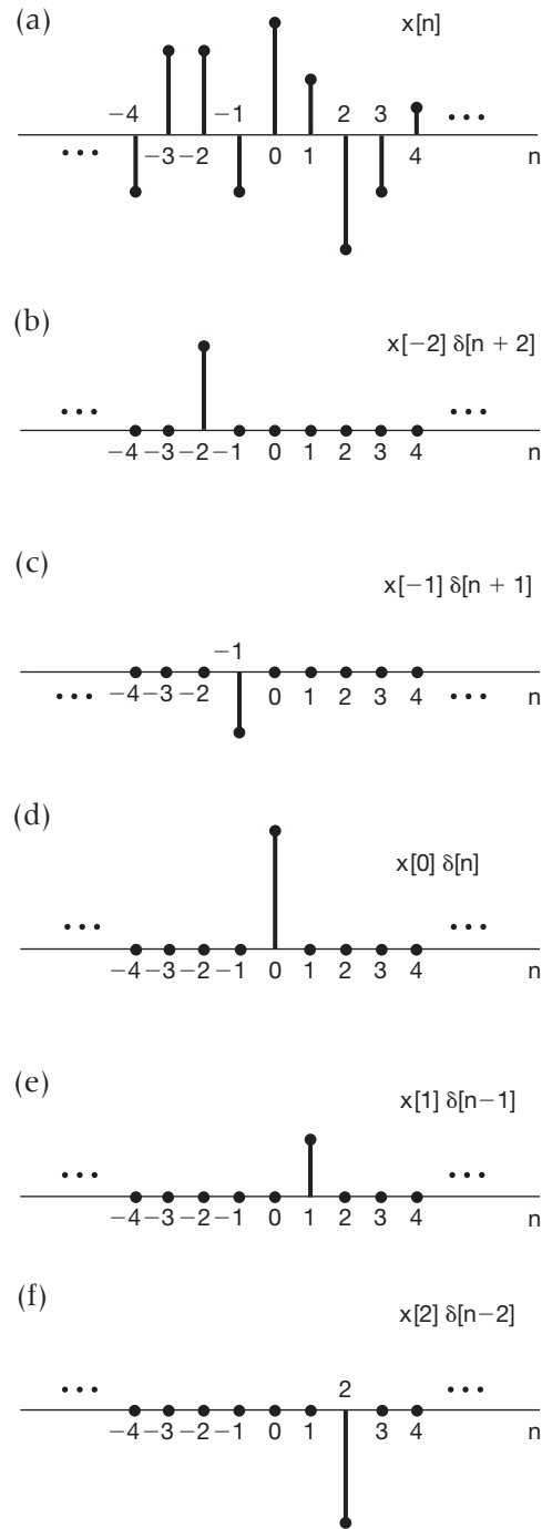
Figura 2.1 Decomposição de um sinal de tempo discreto em uma soma de impulsos ponderados e deslocados.
