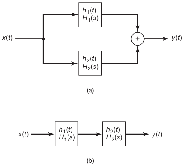
Figura 9.30 a) Interconexão paralela de dois sistemas LIT. (b) Combinação em série de dois sistemas LIT.
