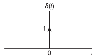
Figura 1.35 Impulso unitário de tempo contínuo.
