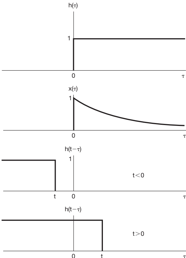
Figura 2.17 Cálculo da integral de convolução do Exemplo 2.6.
