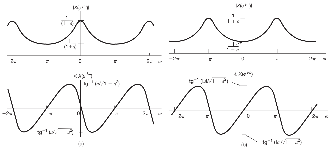
Figura 5.4 Magnitude e fase da transformada de Fourier do Exemplo 5.1 para (a) a > 0 e (b) a < 0 .
