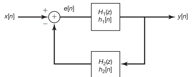
Figura 10.17 Interconexão de realimentação de dois sistemas.
