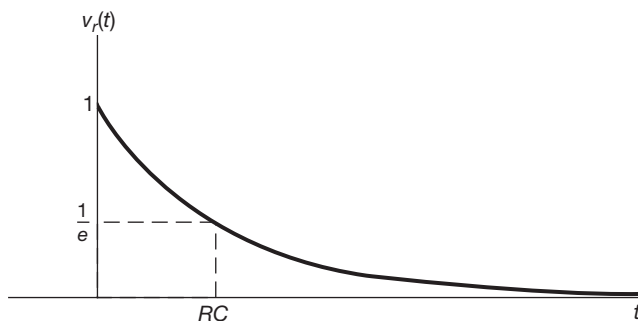
Figura 3.33 Resposta ao degrau do filtro passa-altas RC de primeira ordem com \tau = RC .
