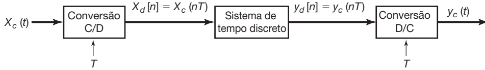
Figura 7.20 Notação para conversão de tempo contínuo para tempo discreto e conversão de tempo discreto para tempo contínuo. T representa o período de amostragem.
