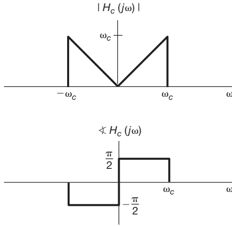
Figura 7.27 Resposta em frequência de um diferenciador de banda limitada ideal de tempo contínuo H_c(j\omega) = j\omega ; |\omega| < \omega_c .
