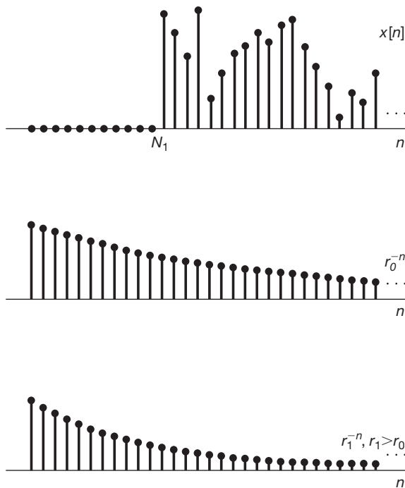
Figura 10.7 Com r_1 > r_0 , x[n]r_1^{-n} decai mais rapidamente com o aumento de n do que x[n]r_0^{-n} . Como x[n] = 0 , n < N_1 , isso implica que se x[n]r_0^{-n} é absolutamente somável, então x[n]r_1^{-n} também o será.
