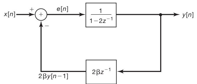
Figura 11.5 Diagrama de blocos de um modelo simples da dinâmica da população com realimentação.
