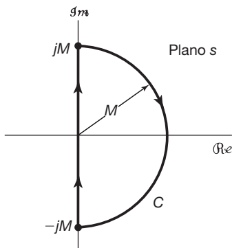
Figura 11.19 Contorno fechado contendo uma parte do semiplano direito; à medida que M \rightarrow \infty , o contorno delimita o semiplano direito inteiro.
