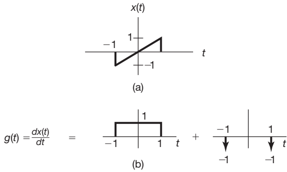
Figura 4.16 (a) Um sinal x(t) para o qual a transformada de Fourier deve ser calculada. (b) Representação da derivada de x(t) como a soma de dois componentes.
