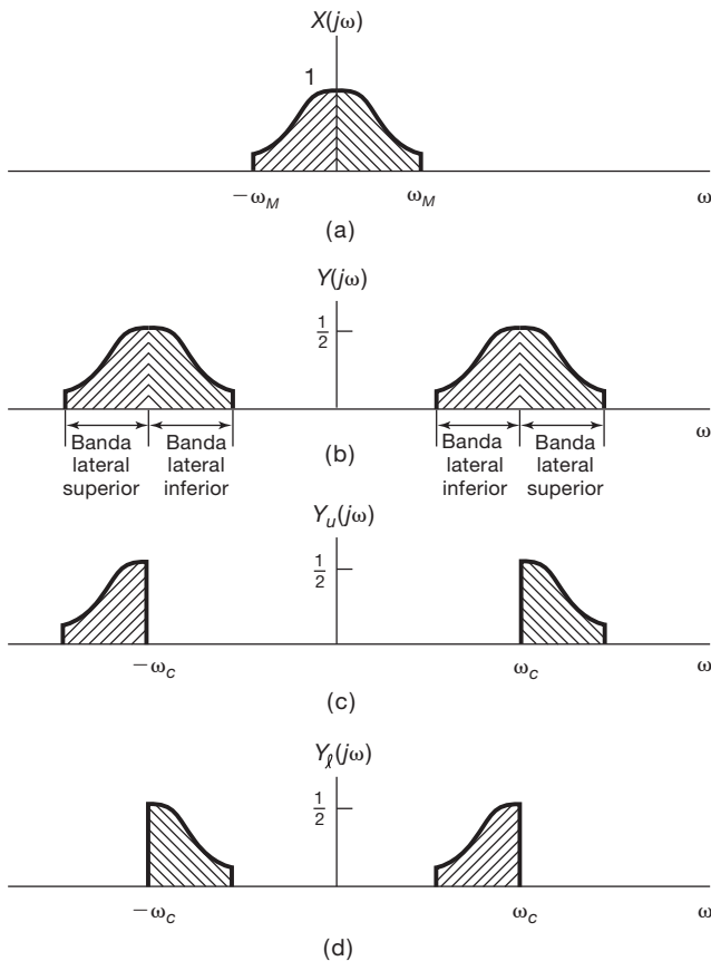
Figura 8.19 Modulação de banda lateral dupla e simples: (a) espectro do sinal modulante; (b) espectro após modulação com portadora senoidal; (c) espectro apenas com bandas laterais superiores; (d) espectro apenas com bandas laterais inferiores.
