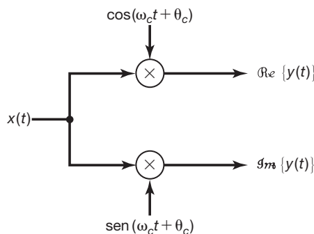
Figura 8.2 Implementação da modulação em amplitude com uma portadora exponencial complexa: c(t) = e^{j(\omega_c t + \theta_c)} .
