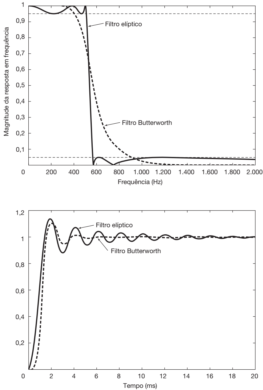
Figura 6.18 Exemplo de um filtro Butterworth de ordem 5 e um filtro elíptico de ordem 5, projetados para terem a mesma ondulação na banda de passagem e banda de rejeição e a mesma frequência de corte (conforme Exemplo 6.3); (a) magnitudes da resposta em frequência em função da frequência medida em hertz; (b) respostas ao degrau.
