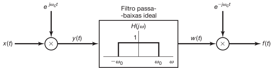
Figura 4.26 Implementação de um filtro passa-faixa usando modulação em amplitude com uma portadora exponencial complexa.
