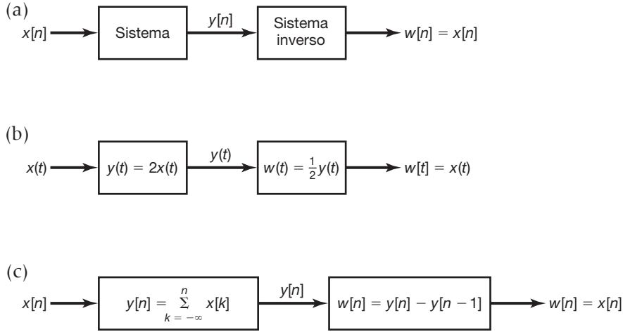
Figura 1.45 Conceito de um sistema inverso para: (a) um sistema invertível geral; (b) sistema invertível descrito pela Equação 1.97; (c) sistema invertível definido na Equação 1.92.
