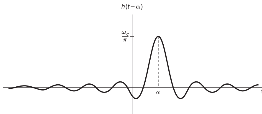
Figura 6.13 Resposta ao impulso de um filtro passa-baixas ideal com magnitude e fase mostradas na Figura 6.11.
