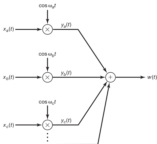
Figura 8.15 Multiplexação por divisão de frequência usando modulação em amplitude senoidal.
