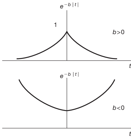
Figura 9.11 Sinal x(t) = e^{-b|t|} para b > 0 e b < 0 .
