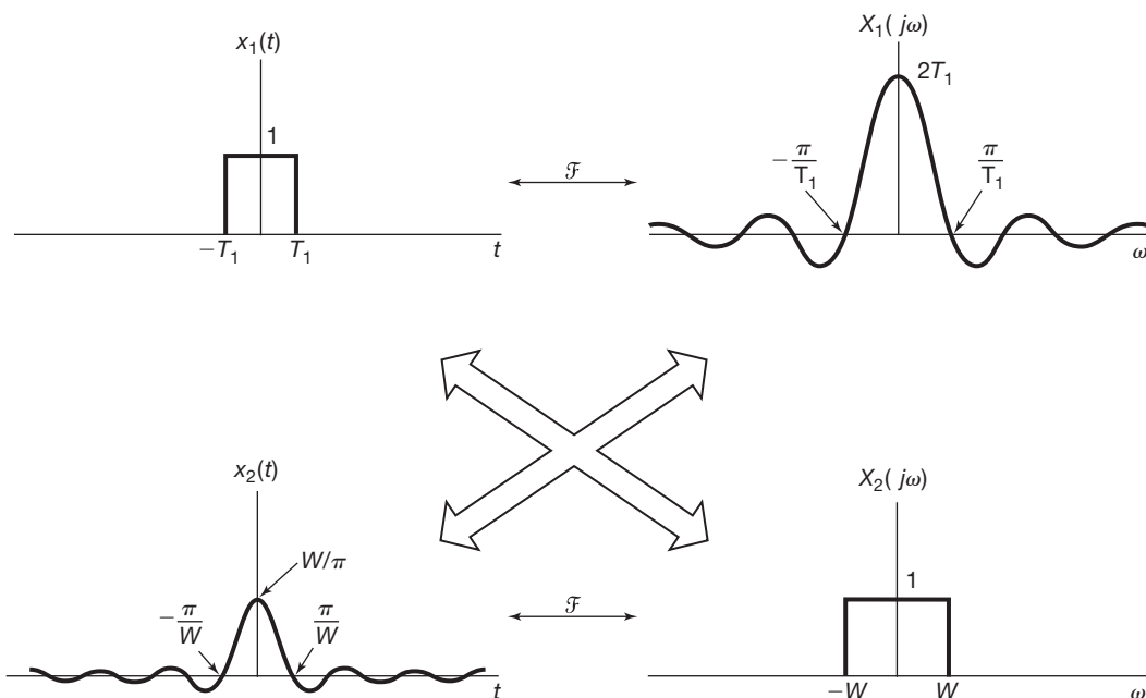
Figura 4.17 Relação entre os pares transformados de Fourier das equações 4.36 e 4.37.
