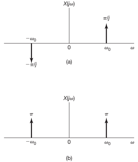
Figura 4.13 Transformadas de Fourier de (a) x(t) = \sin \omega_0 t , (b) x(t) = \cos \omega_0 t , do Exemplo 4.7.
