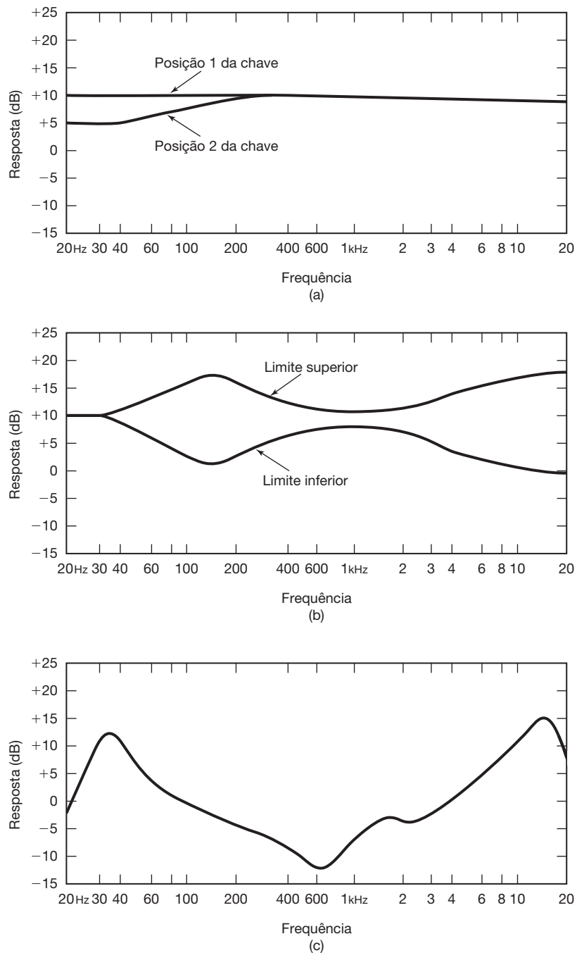
Figura 3.22 Magnitudes das respostas em frequência dos circuitos equalizadores para uma série particular de alto-falantes de áudio, mostradas em uma escala de 20 \log_{10} |H(j\omega)| , que é conhecida como uma escala em decibéis (ou dB). (a) Filtro de baixas frequências controlado por uma chave de duas posições; (b) limites de frequência superior e inferior em um filtro conformador de ajuste contínuo; (c) resposta em frequência fixa do estágio equalizador.
