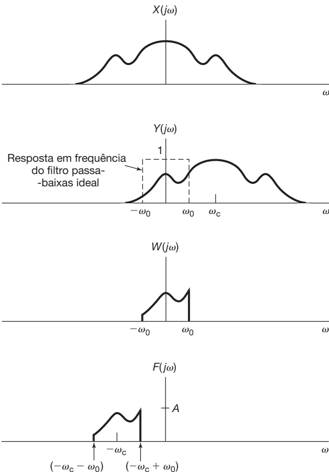
Figura 4.27 Espectros dos sinais do sistema da Figura 4.26.
