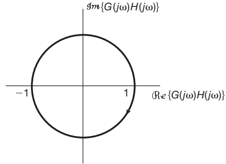
Figura 11.23 Diagrama de Nyquist para o Exemplo 11.7.
