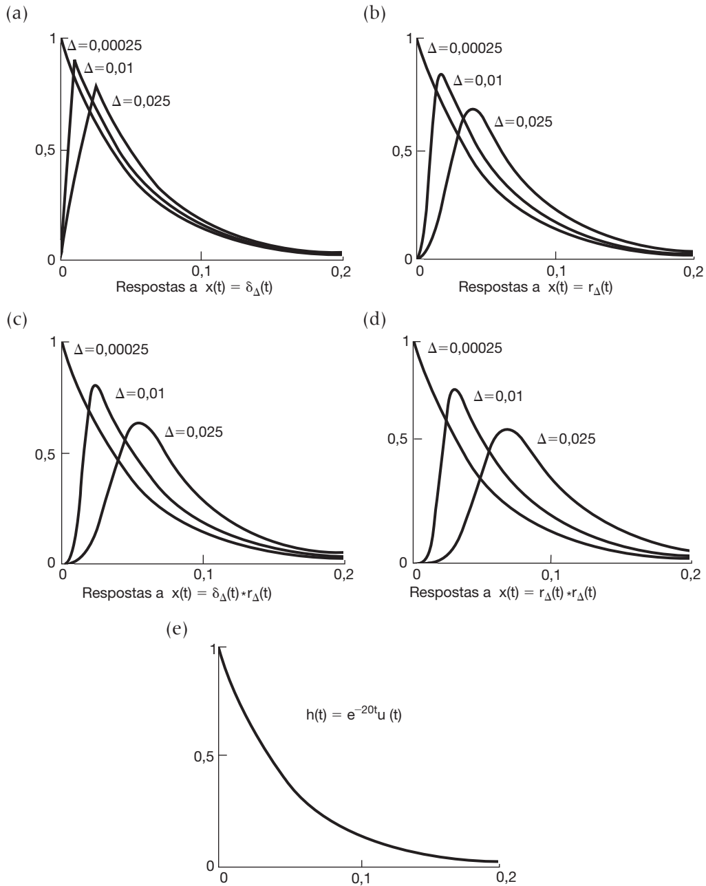
Figura 2.35 Encontrar um valor de \Delta que seja “suficientemente pequeno” depende do sistema no qual estamos aplicando as entradas: (a) respostas do sistema LIT causal descrito pela Equação 2.137 à entrada \delta_\Delta(t) para \Delta = 0,025, 0,01 e 0,00025 ; (b) respostas a r_\Delta(t) ; (c) respostas a \delta_\Delta(t) * r_\Delta(t) ; (d) respostas a r_\Delta(t) * r_\Delta(t) ; (e) resposta ao impulso h(t) = e^{-20t}u(t) para o sistema. Comparando essas respostas às da Figura 2.34, percebemos que é preciso usar um valor menor de \Delta nesse caso antes que a duração e a forma do pulso não tenham consequência.
