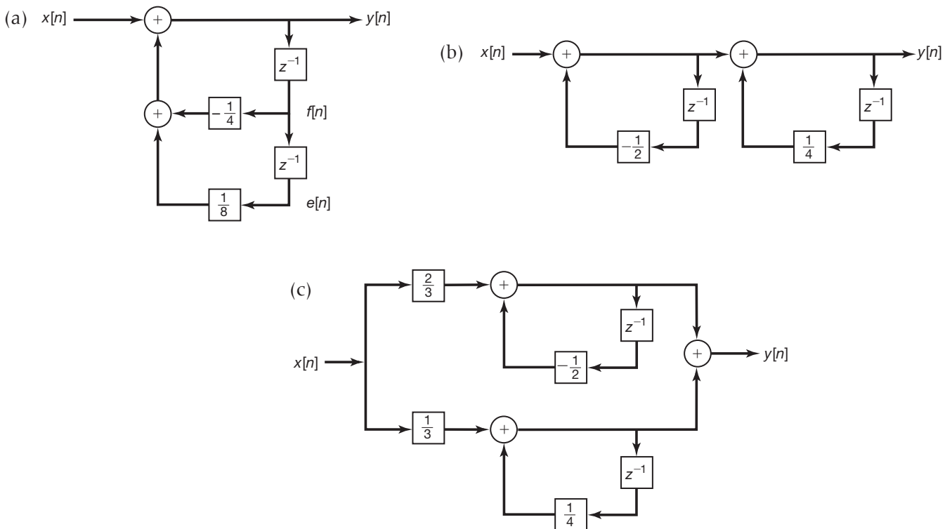
Figura 10.20 Representações por diagrama de blocos para o sistema do Exemplo 10.30: (a) forma direta; (b) forma em cascata; (c) forma paralela.
