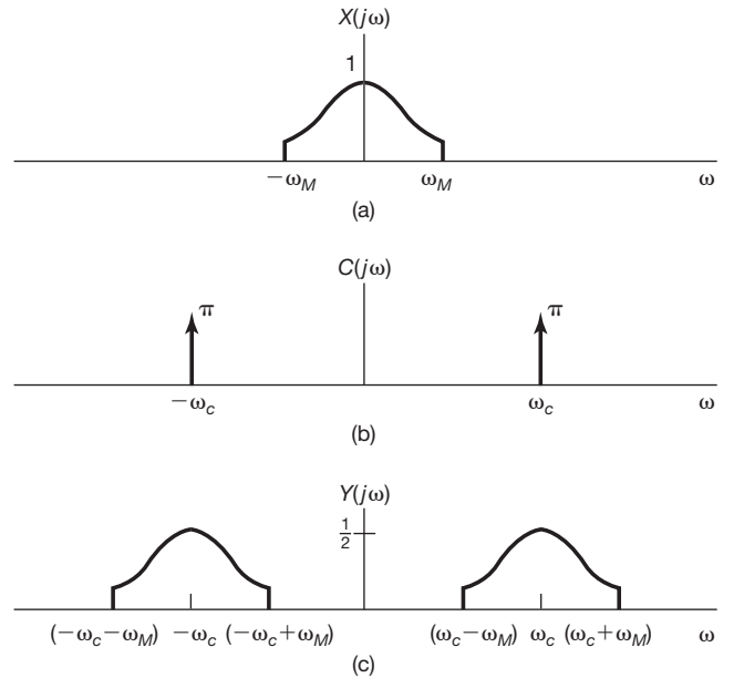
Figura 8.4 Efeito no domínio de frequência da modulação em amplitude com portadora senoidal: (a) espectro do sinal modulante x(t) ; (b) espectro da portadora c(t) = \cos \omega_c t ; (c) espectro do sinal modulado em amplitude.
