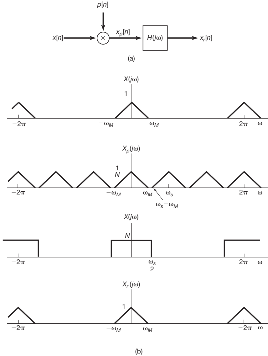
Figura 7.33 Recuperação exata de um sinal de tempo discreto a partir de suas amostras usando um filtro passa-baixas ideal: (a) diagrama de blocos para amostragem e reconstrução de um sinal de banda limitada a partir de suas amostras; (b) espectro do sinal x[n] ; (c) espectro de x_p[n] ; (d) resposta em frequência de um filtro passa-baixas ideal com frequência de corte \omega_s/2 ; (e) espectro do sinal reconstruído x_r[n] . Para o exemplo representado aqui, \omega_s > 2\omega_M de modo que nenhum aliasing ocorra e, por conseguinte, x_r[n] = x[n] .
