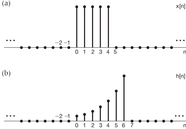
Figura 2.8 Sinais a serem convoluídos no Exemplo 2.4.
