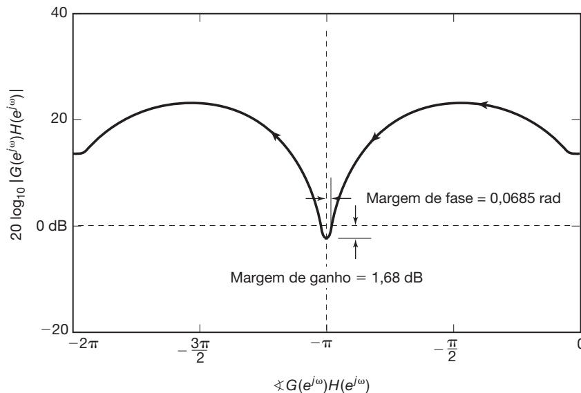
Figura 11.34 Gráfico logarítmico de magnitude-fase para o sistema com realimentação de tempo discreto do Exemplo 11.13.
