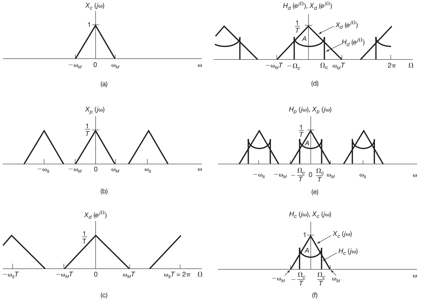
Figura 7.25 Ilustração no domínio de frequência do sistema da Figura 7.24: (a) espectro de tempo contínuo X_c(j\omega) ; (b) espectro após amostragem com trem de impulsos; (c) espectro da sequência de tempo discreto x_d[n] ; (d) H_d(e^{j\Omega}) e X_d(e^{j\Omega}) que são multiplicados para formar Y_d(e^{j\Omega}) ; (e) espectros que são multiplicados para formar Y_p(j\omega) ; (f) espectros que são multiplicados para formar Y_c(j\omega) .
