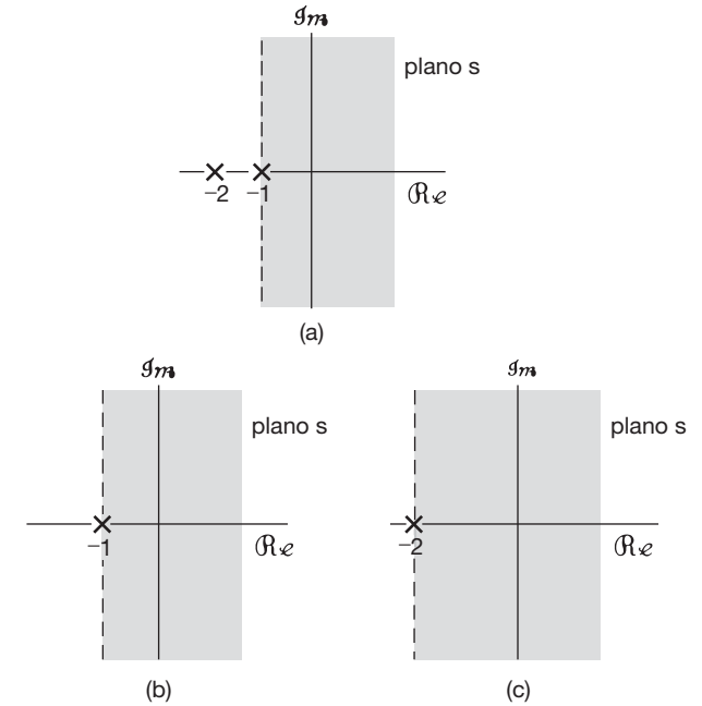
Figura 9.14 Construção das RDCs para os termos individuais na expansão em frações parciais de X(s) do Exemplo 9.8: (a) diagrama de polos e zeros e RDC para X(s) ; (b) polo em s = -1 e sua RDC; (c) polo em s = -2 e sua RDC.
