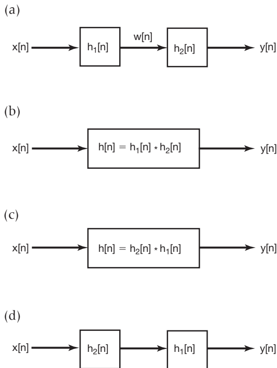
Figura 2.25 Propriedade associativa da convolução, sua implicação e a propriedade comutativa para a interconexão em séries dos sistemas LIT.
