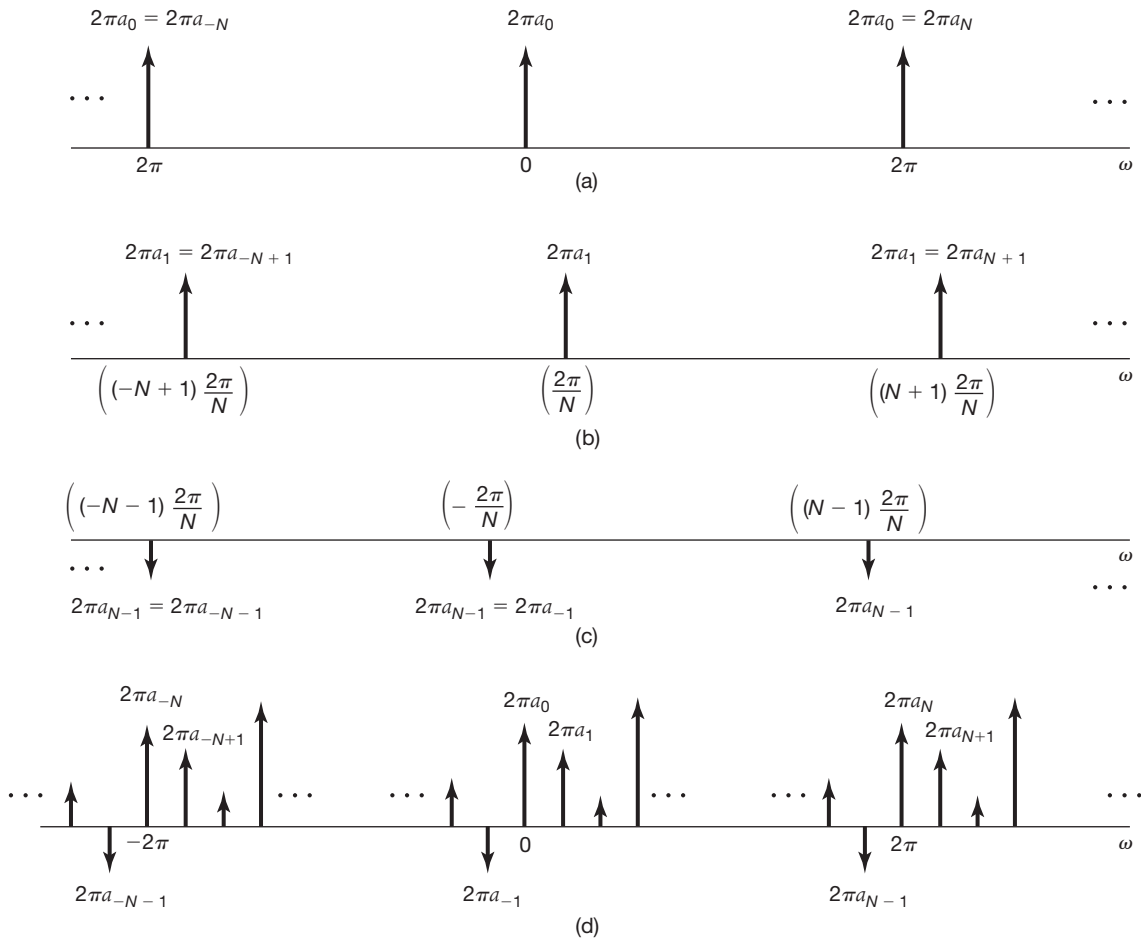
Figura 5.9 Transformada de Fourier de um sinal periódico de tempo discreto: (a) transformada de Fourier da primeira parcela no membro direito da Equação 5.21; (b) transformada de Fourier da segunda parcela na Equação 5.21; (c) transformada de Fourier da última parcela na Equação 5.21; (d) transformada de Fourier de x[n] na Equação 5.21.
