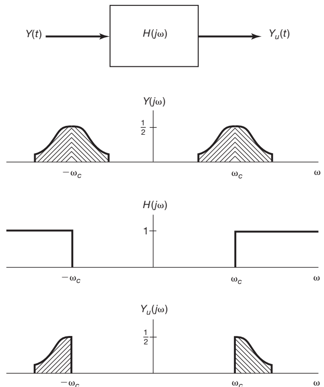
Figura 8.20 Sistema que retém as bandas laterais superiores usando o filtragem passa-altas ideal.
