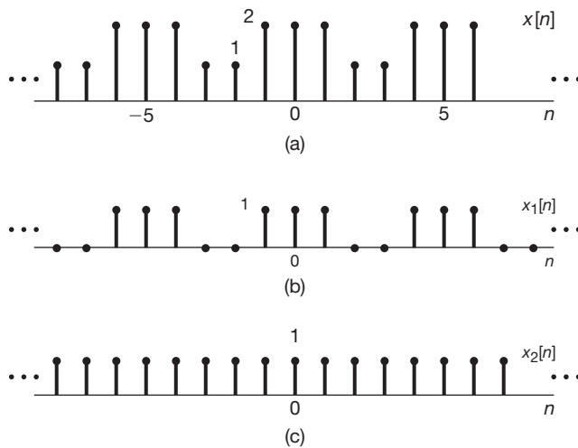
Figura 3.19 (a) Sequência periódica x[n] para o Exemplo 3.13 e sua representação como uma soma de (b) a onda quadrada x_1[n] e (c) a sequência dc x_2[n] .
