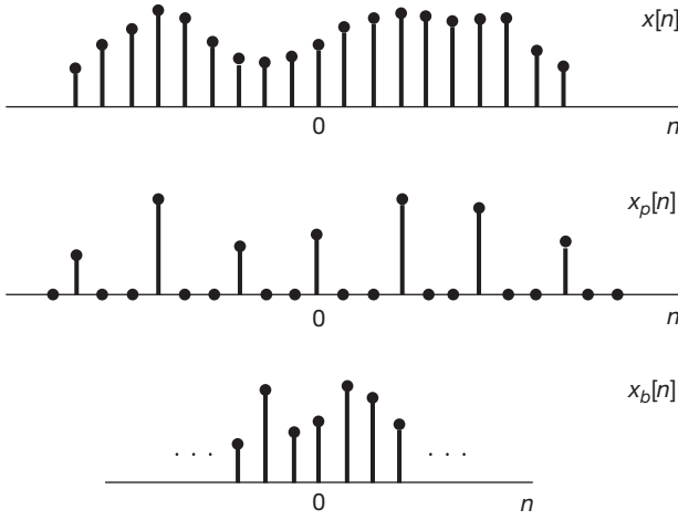
Figura 7.34 Relação entre x_p[n] correspondente à amostragem e x_b[n] correspondente à dizimação.
