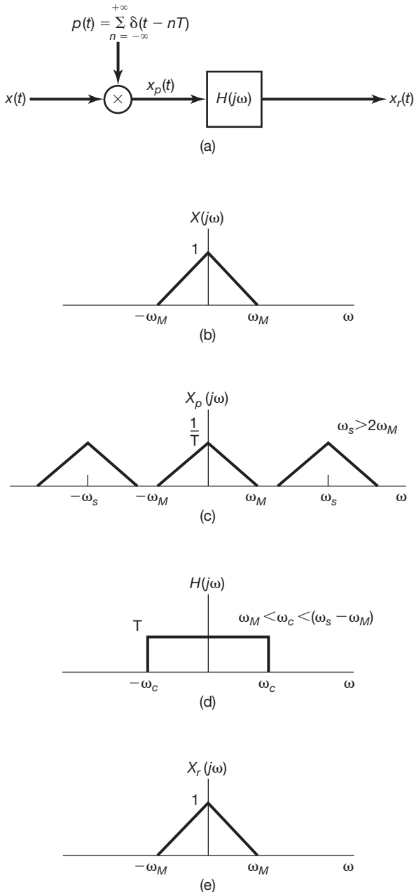
Figura 7.4 Recuperação exata de um sinal de tempo contínuo a partir de suas amostras usando um filtro passa-baixas ideal. (a) Sistema para amostragem e reconstrução. (b) Espectro representativo para x(t) . (c) Espectro correspondente para x_p(t) . (d) Filtro passa-baixas ideal para recuperar X(j\omega) a partir de X_p(j\omega) . (e) Espectro de x_r(t) .
