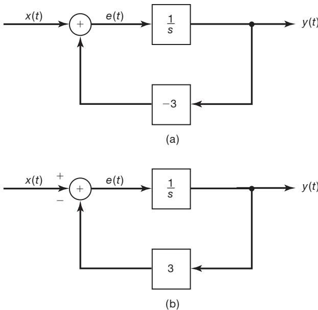
Figura 9.32 (a) Representação em diagrama de blocos do sistema LIT causal no Exemplo 9.28. (b) Representação em diagrama de blocos equivalente.
