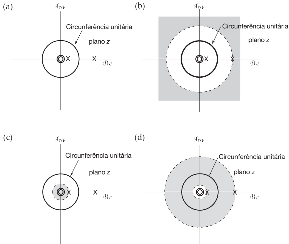
Figura 10.12 As três RDCs possíveis que podem ser associadas à expressão da transformada z no Exemplo 10.8: (a) diagrama de polos e zeros para X(z) ; (b) diagrama de polos e zeros e RDC se x[n] for lateral direita; (c) diagrama de polos e zeros e RDC se x[n] for lateral esquerda; (d) diagrama de polos e zeros e RDC se x[n] for bilateral. Em cada caso, o zero na origem é um zero de segunda ordem.
