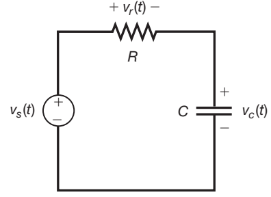
Figura 3.29 Filtro RC de primeira ordem.
