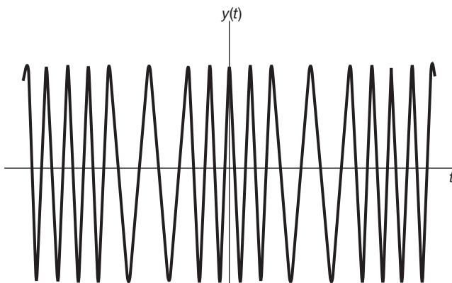
Figura 8.37 Modulação em frequência com um sinal modulante de onda quadrada periódica.
