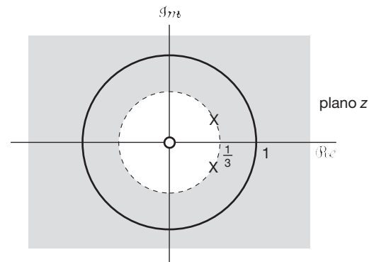
Figura 10.5 Diagrama de polos e zeros e RDC para a transformada z do Exemplo 10.4.
