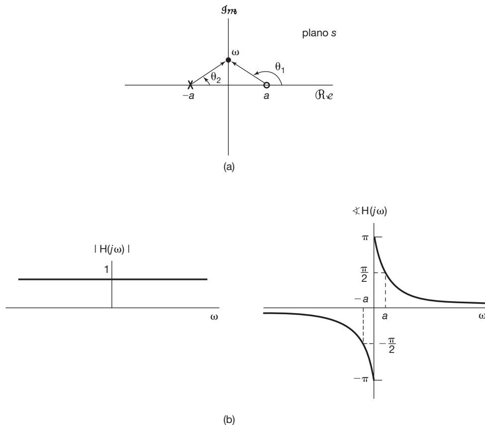
Figura 9.21 (a) Diagrama de polos e zeros para um sistema passa-tudo. (b) Magnitude e fase de uma resposta em frequência passa-tudo.
