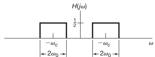
Figura 4.30 Filtro passa-faixa equivalente para \Re\{f(t)\} da Figura 4.29.
