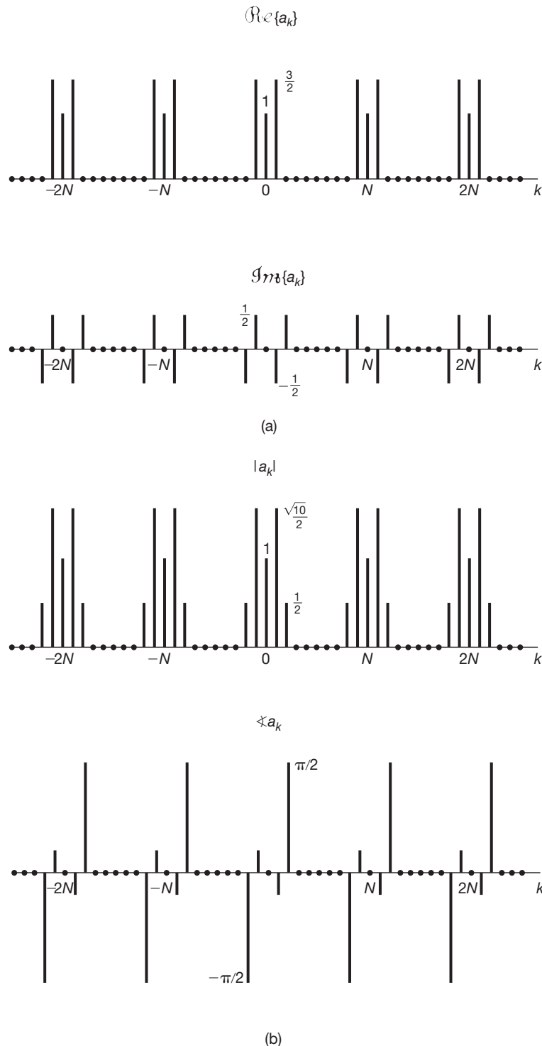
Figura 3.15 (a) Partes real e imaginária dos coeficientes da série de Fourier no Exemplo 3.11; (b) magnitude e fase dos mesmos coeficientes.
