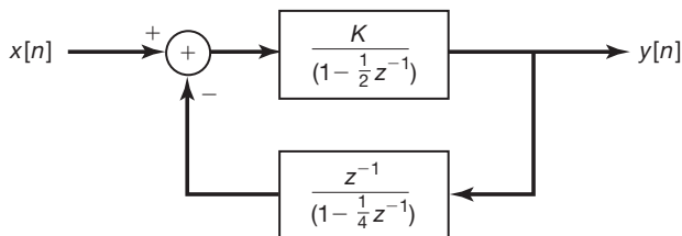
Figura 11.15 Sistema com realimentação de tempo discreto do Exemplo 11.3.
