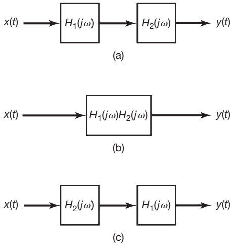
Figura 4.19 Três sistemas LIT equivalentes. Aqui, cada bloco representa um sistema LIT com a resposta em frequência indicada.
