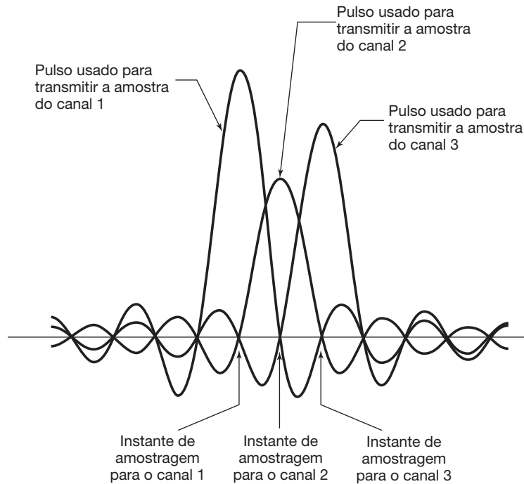
Figura 8.30 Ausência de interferência intersimbólica quando são usados pulsos sinc com cruzamentos de zero corretamente escolhidos.
