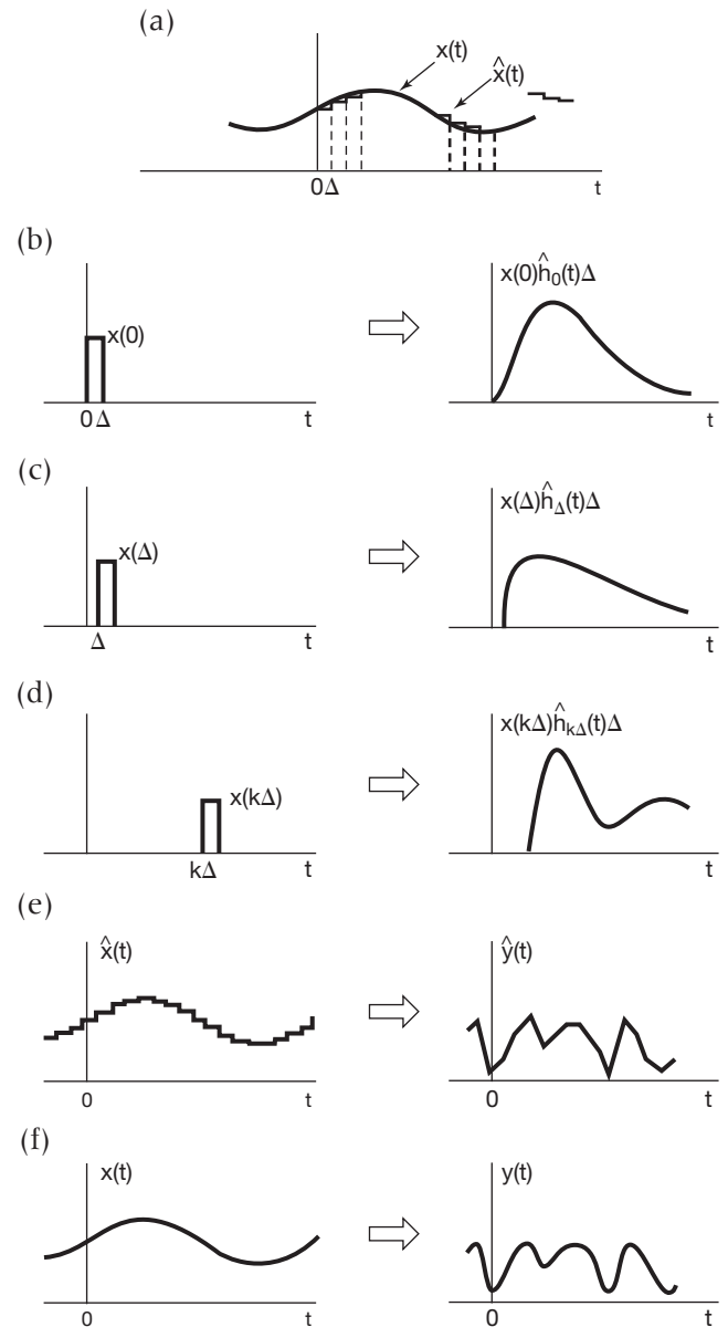
Figura 2.15 Interpretação gráfica da resposta de um sistema linear de tempo contínuo conforme expresso nas equações 2.29 e 2.30.
