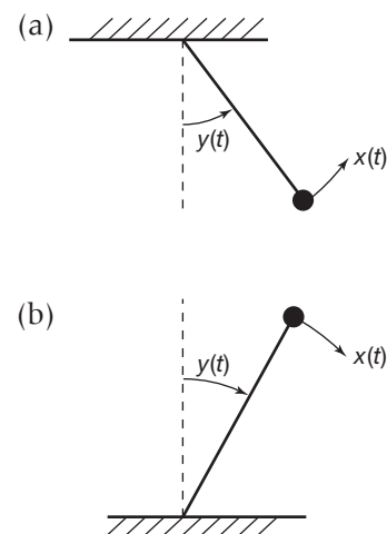
Figura 1.46 (a) Pêndulo estável; (b) pêndulo invertido instável.
