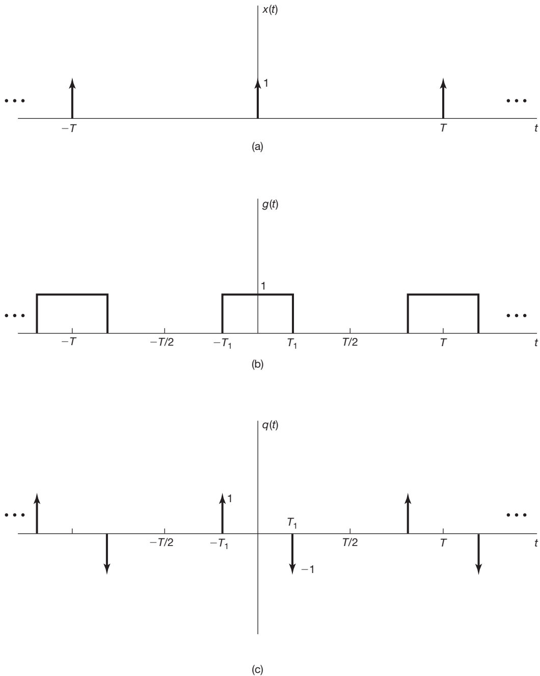
Figura 3.12 (a) Trem de impulso periódico; (b) onda quadrada periódica; (c) derivada da onda quadrada periódica em (b).
