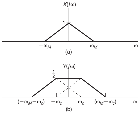
Figura 8.5 Modulação em amplitude senoidal com portadora \cos \omega_c t com \omega_c = \omega_M/2 : (a) espectro do sinal modulante; (b) espectro do sinal modulado.
