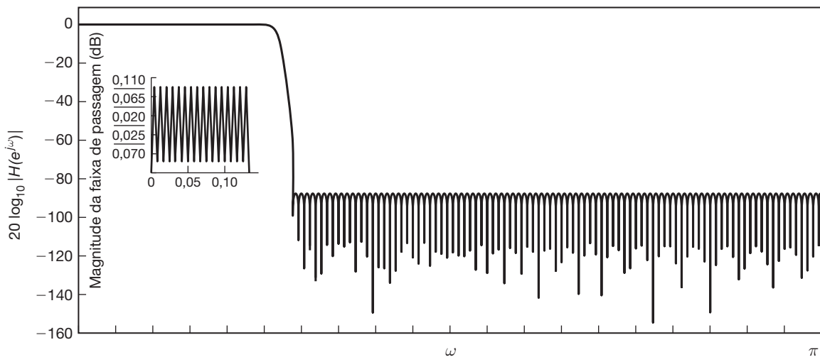
Figura 6.39 Filtro não recursivo passa-baixas com 251 coeficientes projetados para obter o corte mais abrupto possível.
