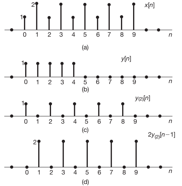
Figura 5.15 (a) O sinal x[n] no Exemplo 5.9; (b) o sinal y[n] ; (c) o sinal y_{(2)}[n] obtido inserindo-se um zero entre valores sucessivos de y[n] ; (d) o sinal 2y_{(2)}[n-1] .
