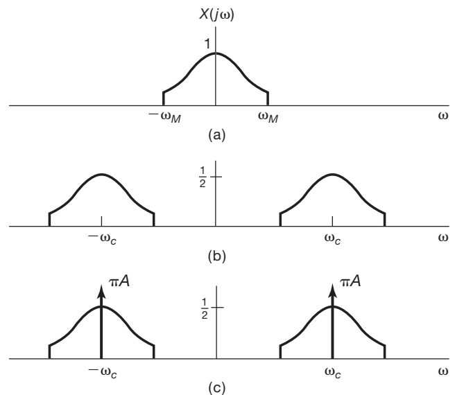
Figura 8.14 Comparação de espectros para sistemas de modulação em amplitude senoidais síncronos e assíncronos: (a) espectro de sinal modulante; (b) espectro de x(t) \cos \omega_c t representando sinal modulado em um sistema síncrono; (c) espectro de [x(t) + A] \cos \omega_c t representando sinal modulado em um sistema assíncrono.
