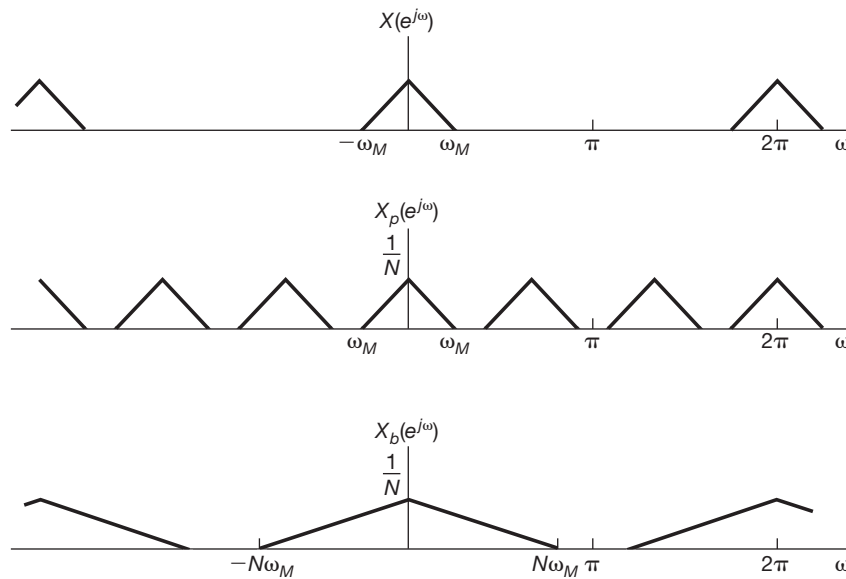
Figura 7.35 Ilustração no domínio de frequência da relação entre amostragem e dizimação.
