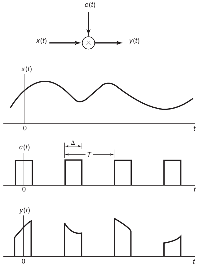
Figura 8.23 Modulação em amplitude de um trem de pulsos.
