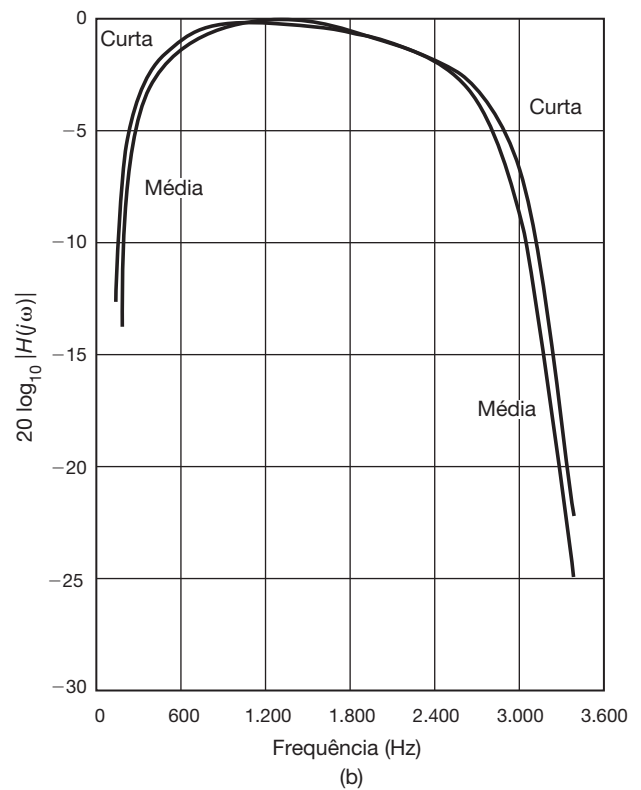
Figura 6.6 (a) Parcela não constante do atraso de grupo; e (b) magnitude da resposta em frequência como funções da frequência para ligações de curta e média distâncias nas redes de telecomunicações comutadas [por Duffy e Thatcher]. Cada uma dessas quantidades é representada em função da frequência medida em hertz. Além disso, como comumente é feito na prática, as magnitudes das respostas em frequência são esboçadas usando-se uma escala logarítmica em unidades de decibéis . Ou seja, o que é esboçado em (b) é 20 \log_{10} |H(j\omega)| para as respostas em frequência correspondentes a ligações de curta e média distâncias. O uso dessa escala logarítmica para as magnitudes de resposta a frequência é discutido com detalhes na Seção 6.2.3.
