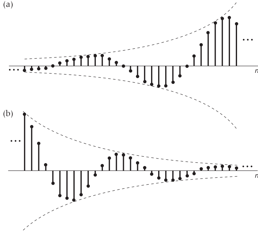
Figura 1.26 (a) Sinais senoidais crescentes de tempo discreto; (b) senoide decrescente de tempo discreto.
