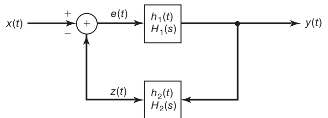
Figura 9.31 Interconexão com realimentação de dois sistemas LIT.
