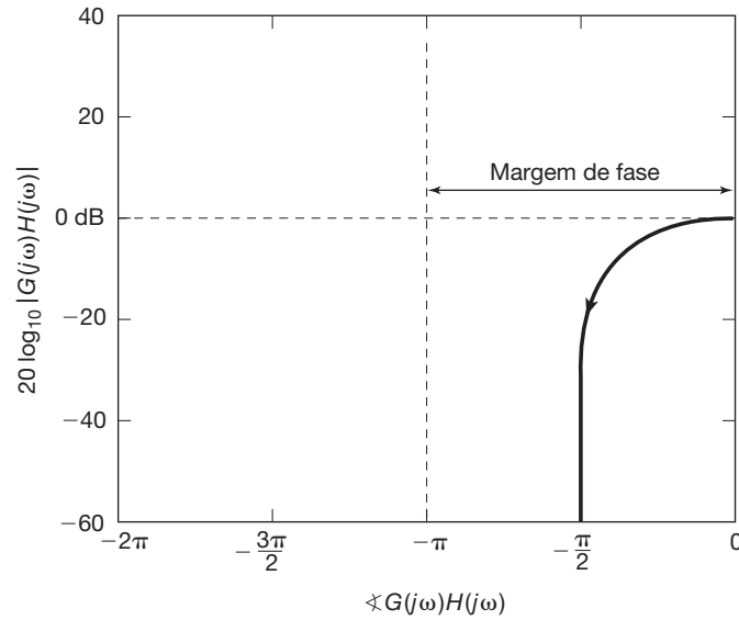
Figura 11.29 Gráfico logarítmico de magnitude-fase para o sistema de primeira ordem do Exemplo 11.10.
