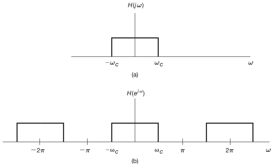
Figura 6.10 (a) A resposta em frequência de um filtro passa-baixas ideal de tempo contínuo; (b) a resposta em frequência de um filtro passa-baixas ideal de tempo discreto.
