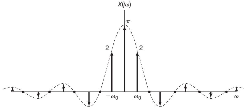
Figura 4.12 Transformada de Fourier de uma onda quadrada periódica simétrica.
