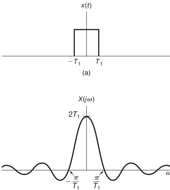
Figura 4.8 (a) O sinal pulso retangular do Exemplo 4.4 e (b) sua transformada de Fourier.
