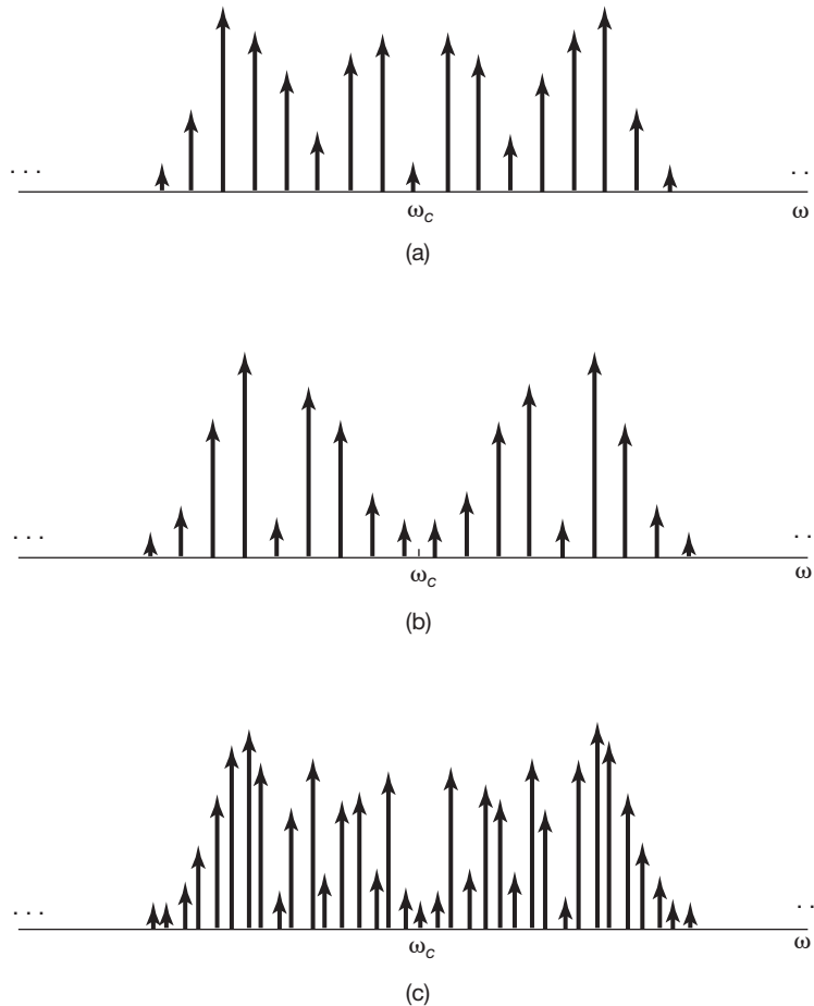
Figura 8.35 Magnitude do espectro da modulação em frequência de banda larga com m = 12 : (a) magnitude do espectro de \cos \omega_c t \cos[m \sin \omega_m t] ; (b) magnitude de espectro de \sin \omega_c t \sin[m \sin \omega_m t] ; (c) magnitude espectral combinada de \cos[\omega_c t + m \sin \omega_m t] .
