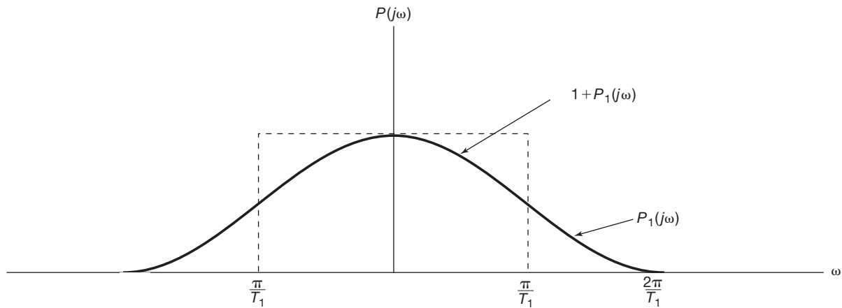
Figura 8.31 Simetria ímpar em torno de \pi/T_1 , conforme definido na Equação 8.29.
