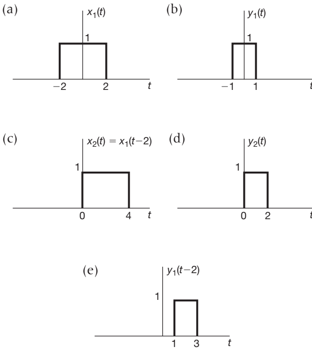
Figura 1.47 (a) Entrada x_1(t) para o sistema do Exemplo 1.16; (b) saída y_1(t) correspondente a x_1(t) ; (c) entrada deslocada x_2(t) = x_1(t - 2) ; (d) saída y_2(t) correspondente a x_2(t) ; (e) sinal deslocado y_1(t - 2) . Note-se que y_2(t) \neq y_1(t - 2) , mostrando que o sistema não é invariante no tempo.
