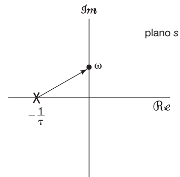
Figura 9.17 Diagrama de polos e zeros para o sistema de primeira ordem da Equação 9.76.
