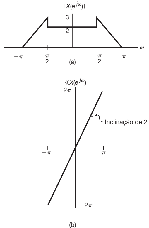
Figura 5.16 Magnitude e fase da transformada de Fourier para o Exemplo 5.10.
