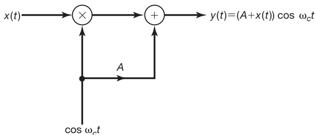
Figura 8.12 Modulador para um sistema de modulação-demodulação assíncrono.
