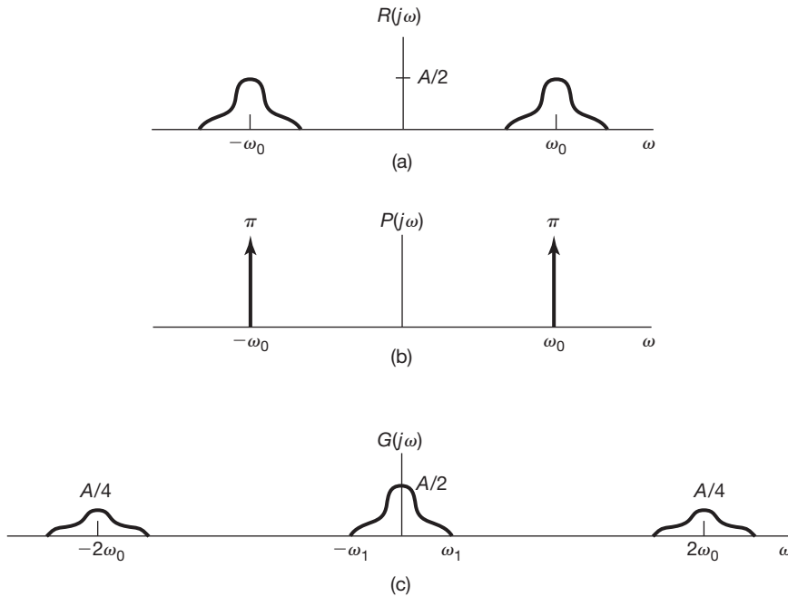
Figura 4.24 Espectros dos sinais considerados no Exemplo 4.22: (a) R(j\omega) ; (b) P(j\omega) ; (c) G(j\omega) .
