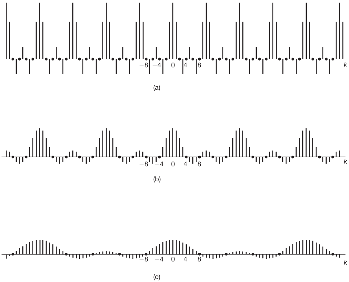
Figura 3.17 Coeficientes da série de Fourier para a onda quadrada periódica do Exemplo 3.12; gráficos de Na_k para 2N_1 + 1 = 5 e (a) N = 10 ; (b) N = 20 ; (c) N = 40 .
