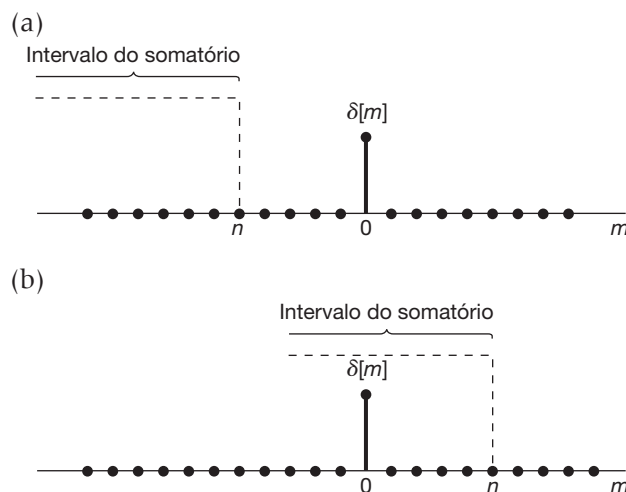
Figura 1.30 Soma cumulativa da Equação 1.66: (a) n < 0 ; (b) n > 0 .
