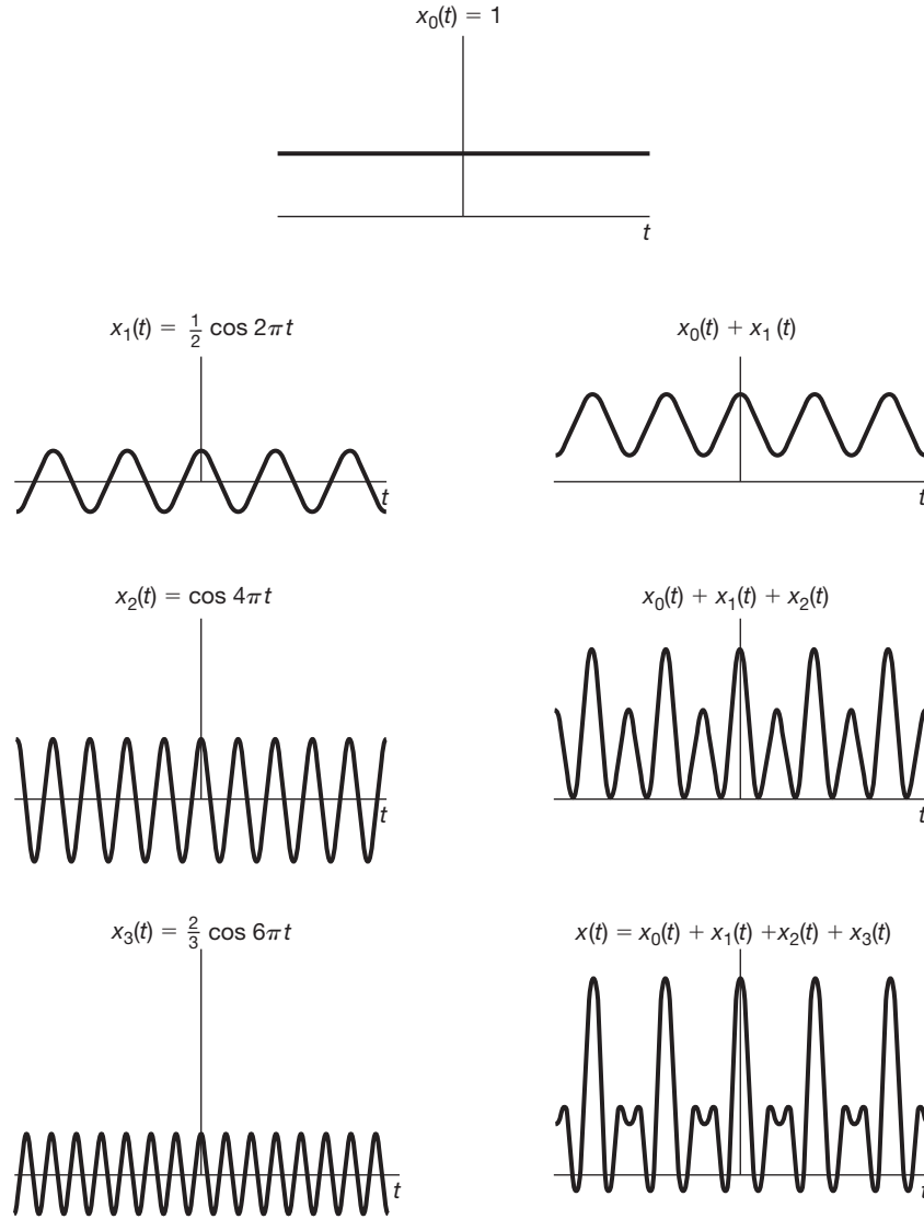
Figura 3.4 Construção do sinal x(t) do Exemplo 3.2 como uma combinação linear de sinais senoidais harmonicamente relacionados.
