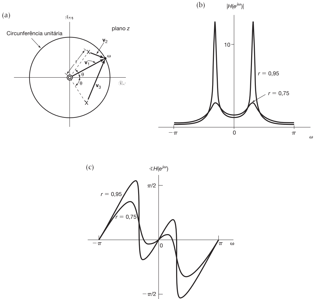
Figura 10.14 (a) Vetor de zeros \mathbf{v}_1 e vetores de polos \mathbf{v}_2 e \mathbf{v}_3 , usados no cálculo das respostas em frequência para um sistema de segunda ordem; (b) magnitude da resposta em frequência correspondente ao inverso do produto dos comprimentos dos vetores dos polos para r = 0,95 e r = 0,75 ; (c) fase da resposta em frequência para r = 0,95 e r = 0,75 .
