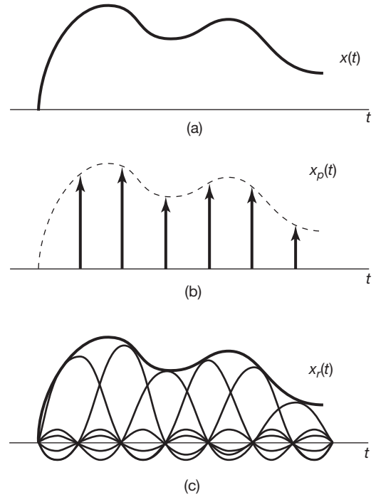
Figura 7.10 Interpolação ideal de banda limitada usando a função sinc. (a) Sinal de banda limitada x(t) . (b) Trem de impulsos de amostras de x(t) . (c) Interpolação ideal de banda limitada em que o trem de impulsos é substituído por uma superposição de funções sinc (Equação 7.11).
