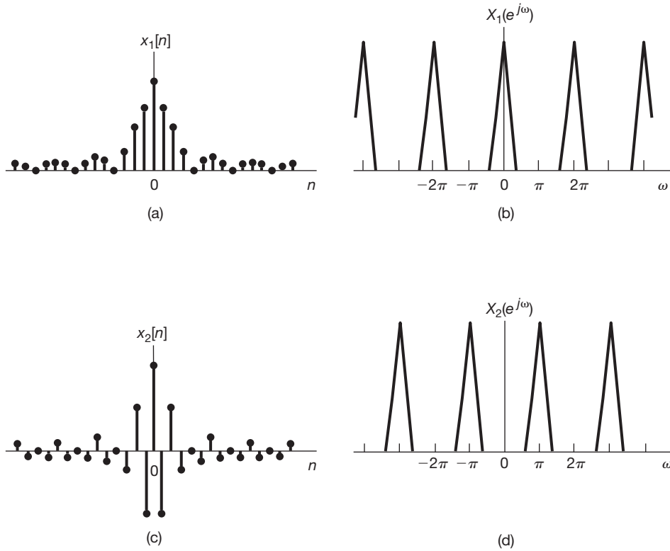
Figura 5.3 (a) Sinal de tempo discreto x_1[n] . (b) Transformada de Fourier de x_1[n] . Observe que X_1(e^{j\omega}) está concentrado perto de \omega = 0, \pm 2\pi, \pm 4\pi, \dots (c) Sinal de tempo discreto x_2[n] . (d) Transformada de Fourier de x_2[n] . Observe que X_2(e^{j\omega}) está concentrado perto de \omega = \pm\pi, \pm 3\pi, \dots
