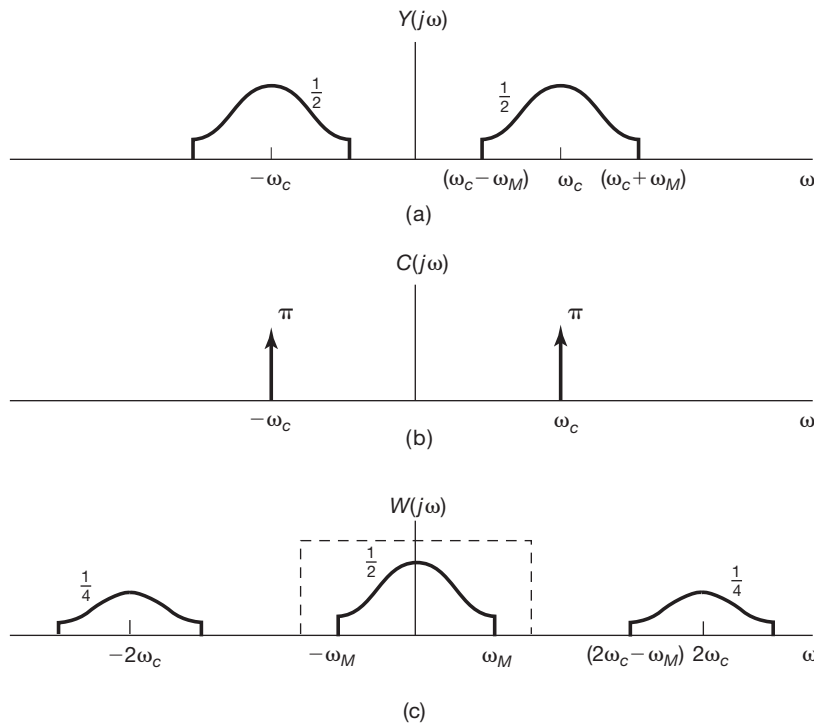
Figura 8.6 Demodulação de um sinal modulado em amplitude com uma portadora senoidal: (a) espectro do sinal modulado; (b) espectro do sinal da portadora; (c) espectro de sinal modulado multiplicado pela portadora. A linha tracejada indica a resposta em frequência de um filtro passa-baixas para extrair o sinal demodulado.
