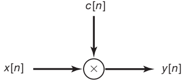
Figura 8.40 Modulação em amplitude de tempo discreto.
