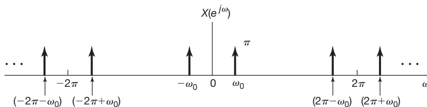
Figura 5.10 Transformada de Fourier de tempo discreto de x[n] = \cos \omega_0 n .
