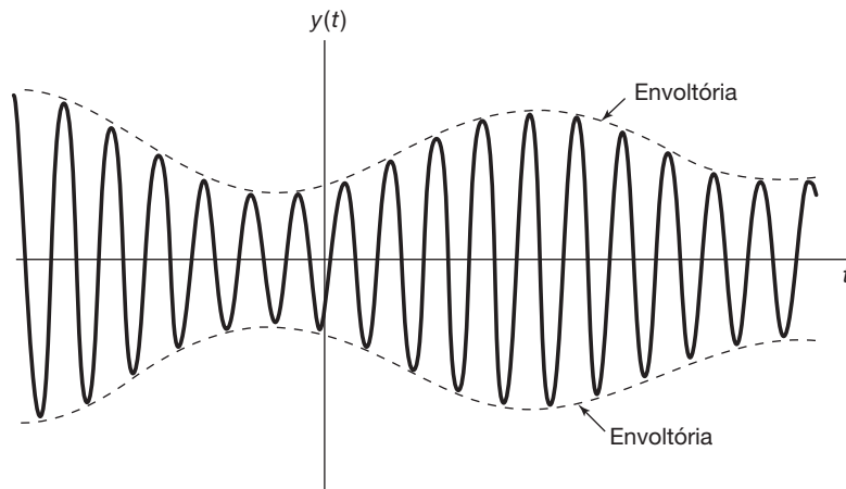
Figura 8.10 Sinal modulado em amplitude para o qual o sinal modulante é positivo. A curva tracejada representa a envoltória do sinal modulado.
