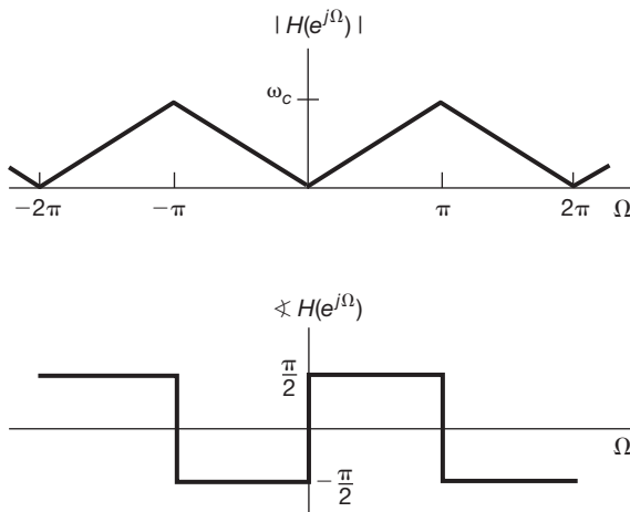
Figura 7.28 Resposta em frequência do filtro de tempo discreto usado para implementar um diferenciador de banda limitada de tempo contínuo.
