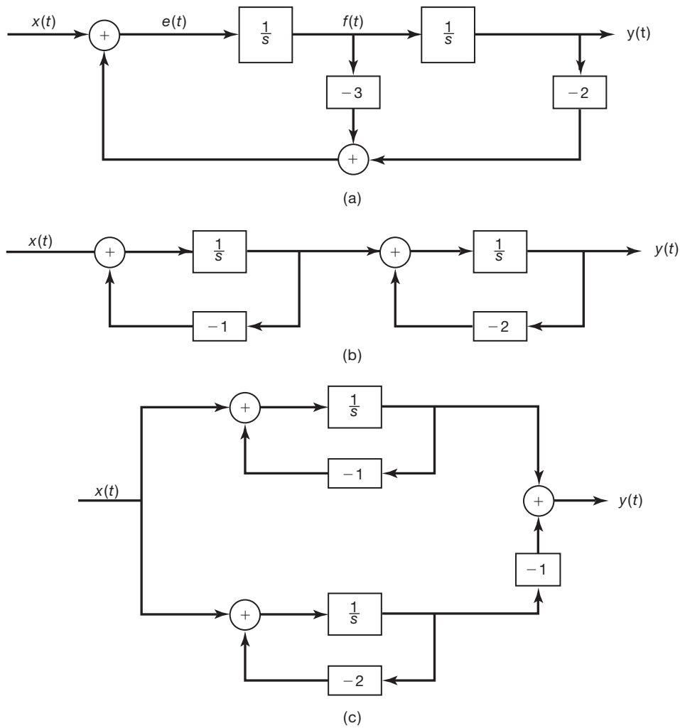
Figura 9.34 Representações em diagrama de blocos para o sistema do Exemplo 9.30: (a) forma direta; (b) forma em cascata; (c) forma paralela.
