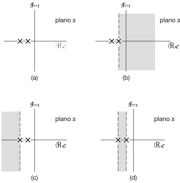
Figura 9.13 (a) Diagrama de polos e zeros do Exemplo 9.8. (b) RDC correspondente a uma sequência lateral direita. (c) RDC correspondente a uma sequência lateral esquerda. (d) RDC correspondente a uma sequência bilateral.
