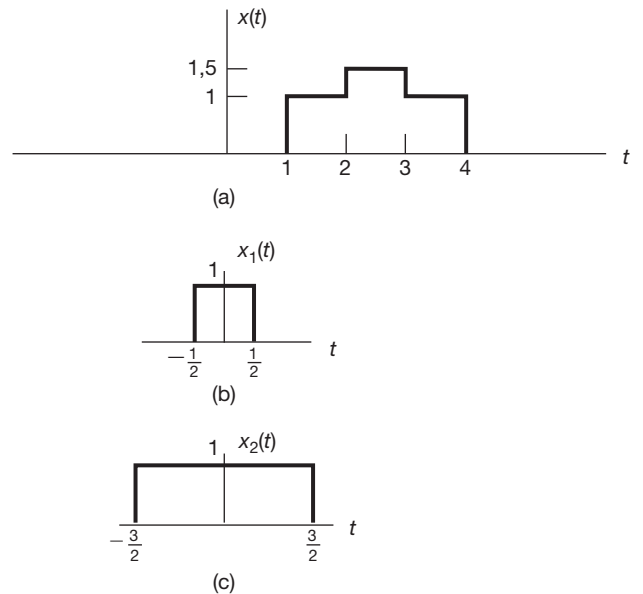
Figura 4.15 Decomposição de um sinal em uma combinação linear de dois sinais mais simples. (a) O sinal x(t) para o Exemplo 4.9; (b) e (c) os dois componentes dos sinais usados para representar x(t) .
