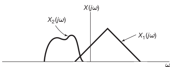
Figura 6.15 Dois espectros que são um pouco sobrepostos.
