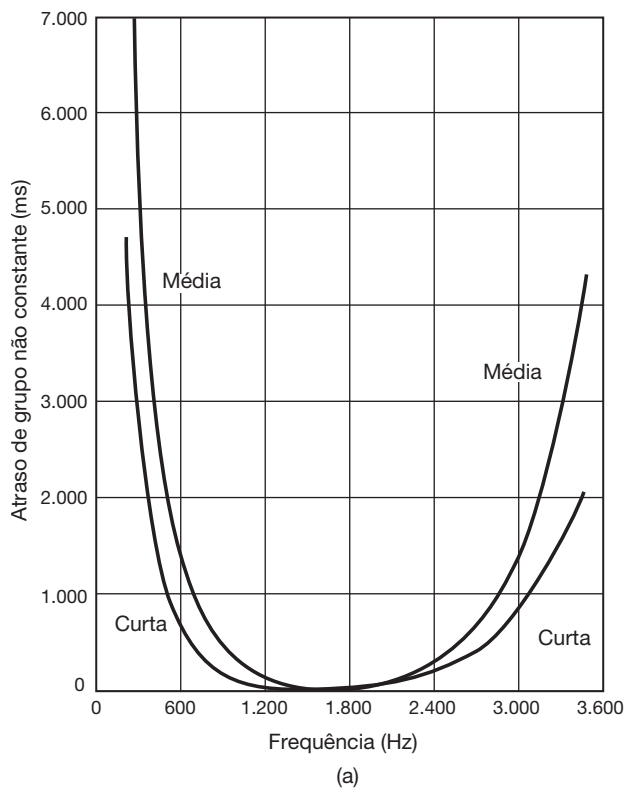
Figura 6.6 (a) Parcela não constante do atraso de grupo; e (b) magnitude da resposta em frequência como funções da frequência para ligações de curta e média distâncias nas redes de telecomunicações comutadas [por Duffy e Thatcher]. Cada uma dessas quantidades é representada em função da frequência medida em hertz. Além disso, como comumente é feito na prática, as magnitudes das respostas em frequência são esboçadas usando-se uma escala logarítmica em unidades de decibéis . Ou seja, o que é esboçado em (b) é 20 \log_{10} |H(j\omega)| para as respostas em frequência correspondentes a ligações de curta e média distâncias. O uso dessa escala logarítmica para as magnitudes de resposta a frequência é discutido com detalhes na Seção 6.2.3.
