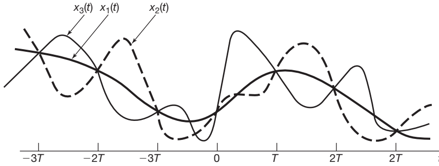
Figura 7.1 Três sinais de tempo contínuo com valores idênticos em múltiplos inteiros de T .
