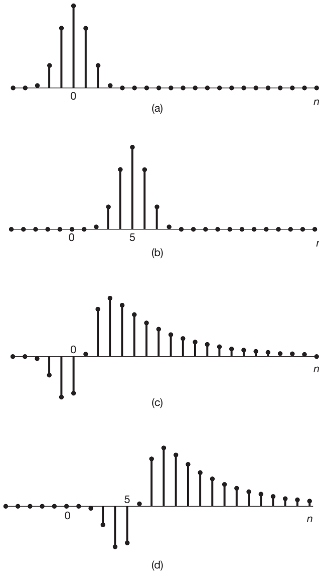
Figura 6.4 (a) Sinal de tempo discreto que é aplicado como entrada para diversos sistemas para os quais a resposta em frequência tem magnitude unitária; (b) resposta para um sistema com fase linear com inclinação de -5 ; (c) resposta para um sistema com fase não linear; (d) resposta para um sistema cuja característica de fase é aquela do item (c) mais um termo de fase linear com inclinação inteira.
