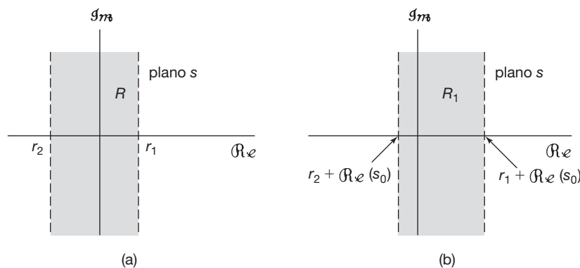
Figura 9.23 Efeito sobre a RDC do deslocamento no domínio s : (a) a RDC de X(s) ; (b) a RDC de X(s - s_0) .
