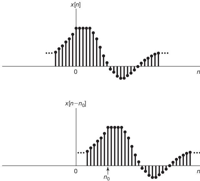
Figura 1.8 Sinais de tempo discreto relacionados por um deslocamento no tempo. Nesta figura, n_0 > 0 , de modo que x[n - n_0] é uma versão atrasada de x[n] (isto é, cada ponto em x[n] aparece atrasado em x[n - n_0] ).
