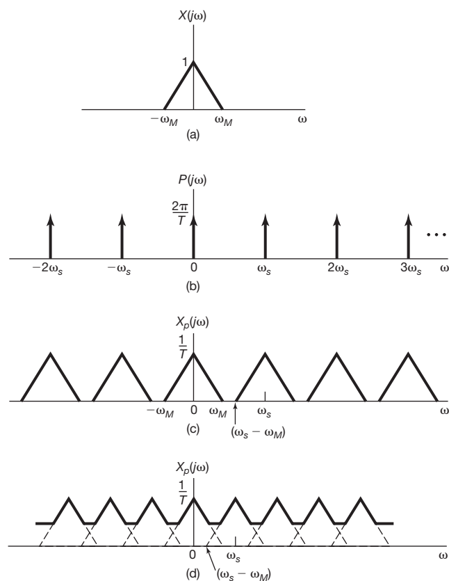
Figura 7.3 Efeito no domínio da frequência da amostragem no domínio do tempo: (a) espectro do sinal original; (b) espectro da função de amostragem; (c) espectro do sinal amostrado com \omega_s > 2\omega_M ; (d) espectro do sinal amostrado com \omega_s < 2\omega_M .
