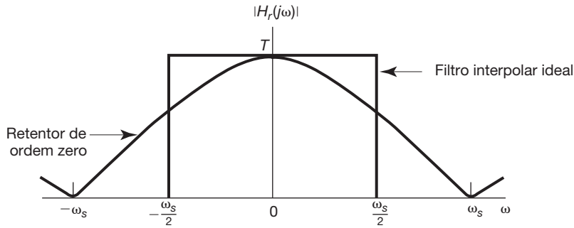
Figura 7.11 Função de transferência para o retentor de ordem zero e para o filtro interpolador ideal.
