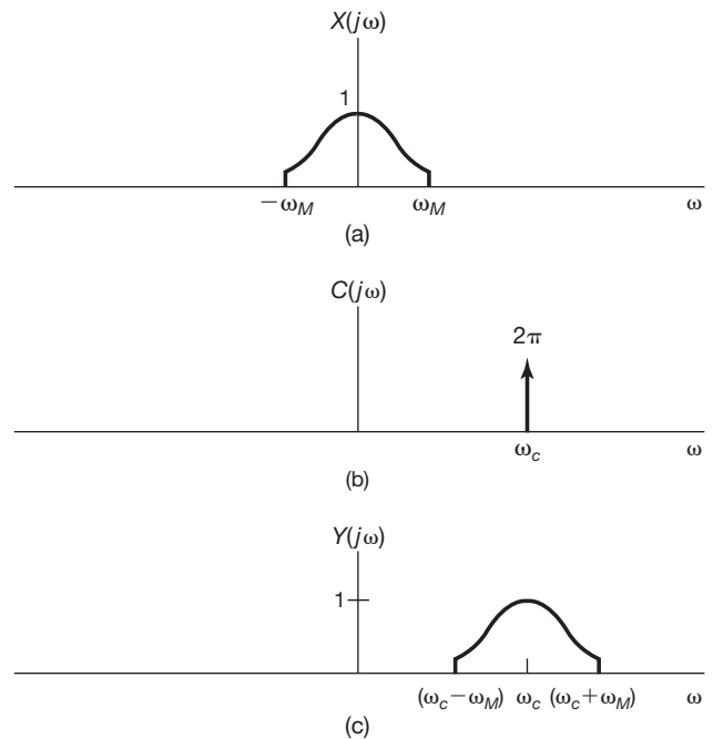
Figura 8.1 Efeito no domínio de frequência da modulação de amplitude com uma portadora complexa: (a) espectro do sinal modulante x(t) ; (b) espectro da portadora c(t) = e^{j\omega_c t} ; (c) espectro de sinal modulado em amplitude y(t) = x(t)e^{j\omega_c t} .
