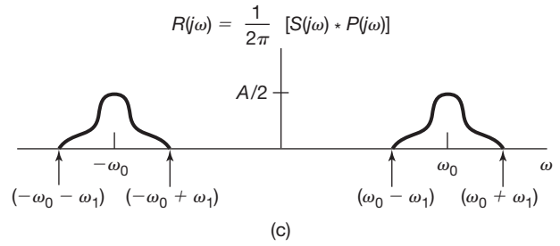
Figura 4.23 Uso da propriedade de multiplicação do Exemplo 4.21: (a) A transformada de Fourier de um sinal s(t) ; (b) a transformada de Fourier de p(t) = \cos \omega_0 t ; (c) a transformada de Fourier de r(t) = s(t)p(t) .
