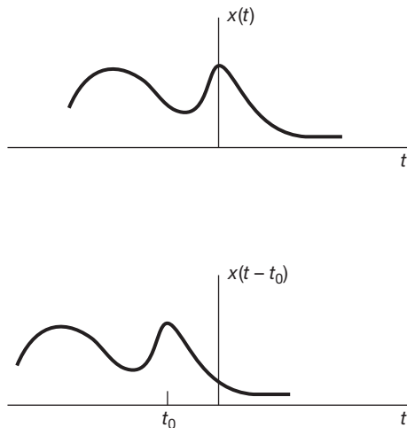
Figura 1.9 Sinais de tempo contínuo relacionados por um deslocamento no tempo. Nesta figura, t_0 < 0 , de modo que x(t - t_0) é uma versão adiantada de x(t) (isto é, cada ponto em x(t) aparece antes em x(t - t_0) ).
