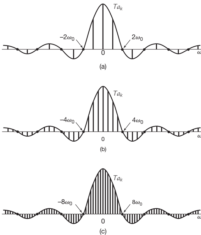
Figura 4.2 Os coeficientes da série de Fourier e sua envoltória para a onda quadrada periódica na Figura 4.1, para diferentes valores de T (com T_1 fixo): (a) T = 4T_1 ; (b) T = 8T_1 ; (c) T = 16T_1 .
