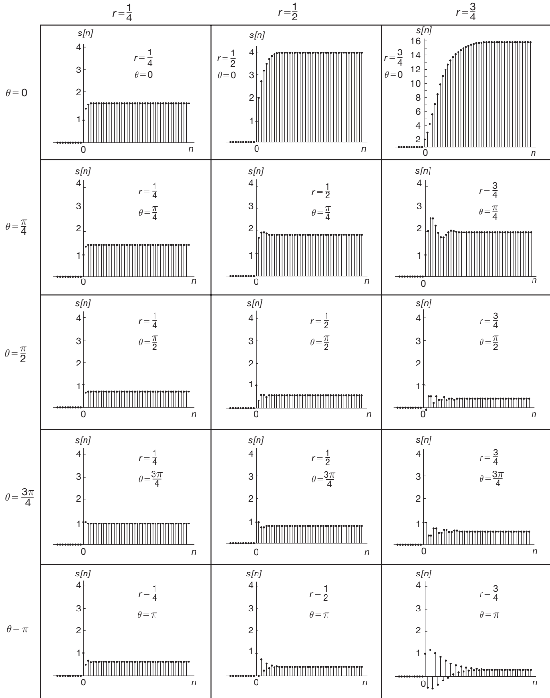
Figura 6.30 Resposta ao degrau do sistema de segunda ordem da Equação 6.57 para diferentes de valores de r e \theta .
