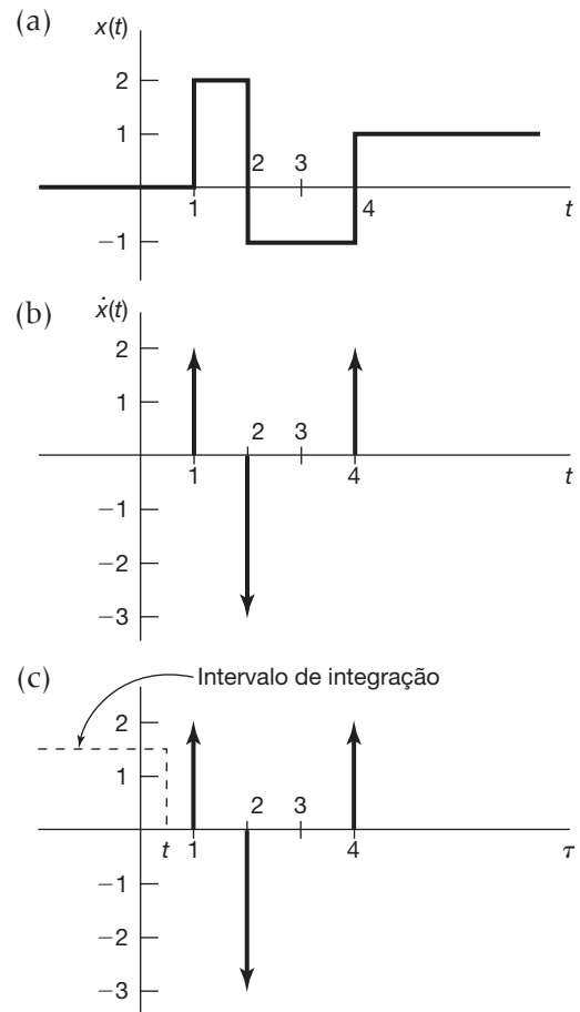
Figura 1.40 (a) Sinal descontínuo x(t) analisado no Exemplo 1.7; (b) sua derivada \dot{x}(t) ; (c) representação da reconstrução de x(t) como integral de \dot{x}(t) , ilustrada para um valor de t entre 0 e 1.
