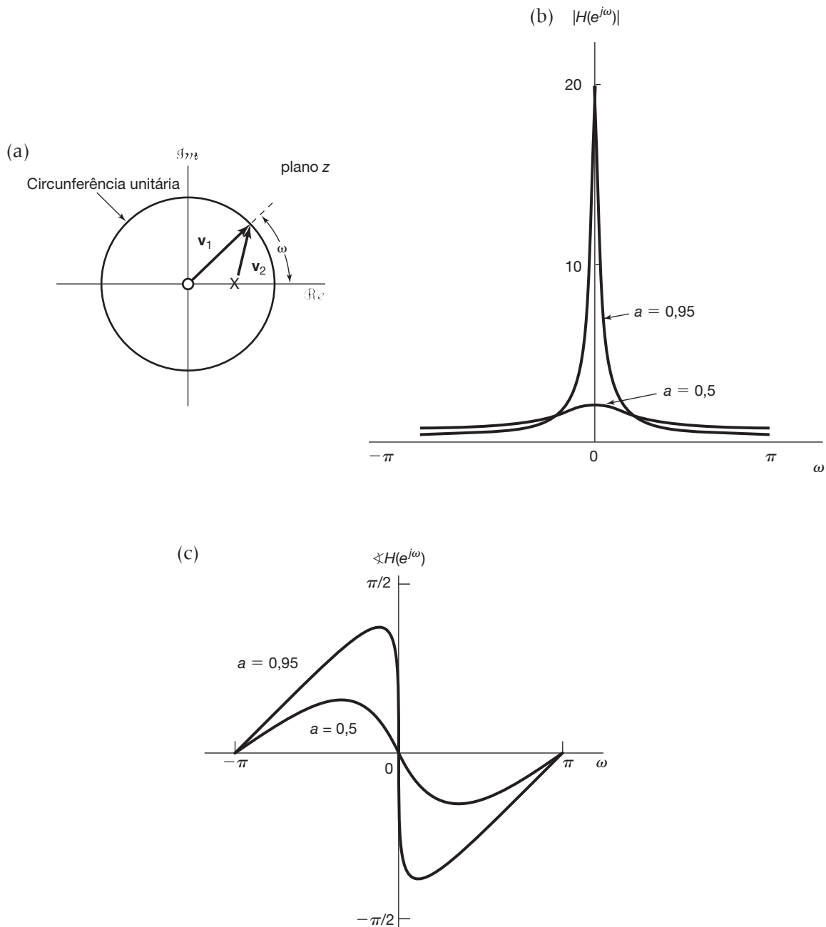
Figura 10.13 (a) Vetores de polos e zeros para a determinação da resposta em frequência para um sistema de primeira ordem com um valor de a entre 0 e 1; (b) magnitude da resposta em frequência para a = 0,95 e a = 0,5 , (c) fase da resposta em frequência para a = 0,95 e a = 0,5 .
