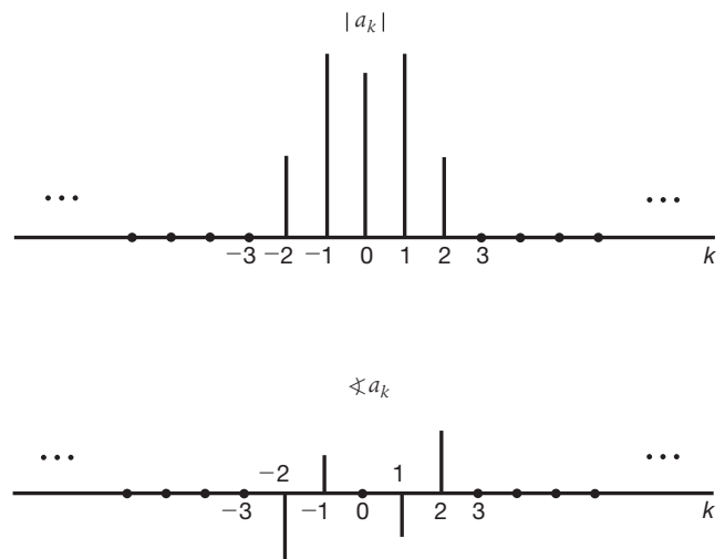
Figura 3.5 Gráficos da magnitude e fase dos coeficientes de Fourier do sinal considerado no Exemplo 3.4.
