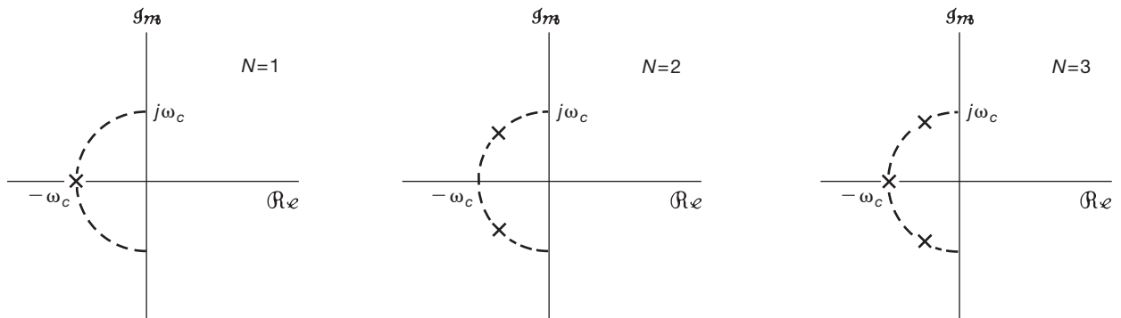
Figura 9.29 Localização dos polos de B(s) para N=1, 2 e 3 .
