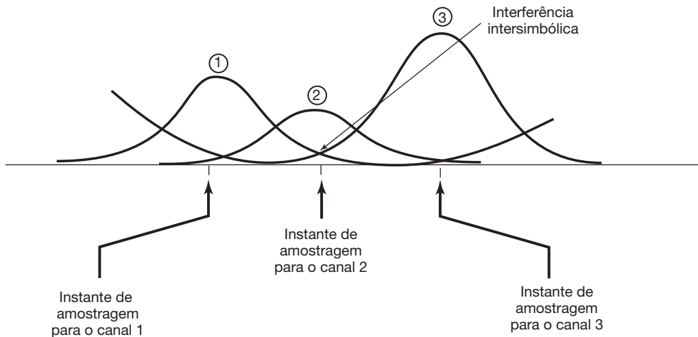
Figura 8.28 Interferência intersimbólica.
