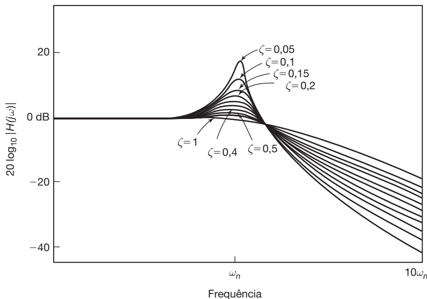
Figura 6.33 Diagrama de Bode de magnitude da resposta em frequência do sistema de suspensão de automóvel para diferentes valores de fator de amortecimento.
