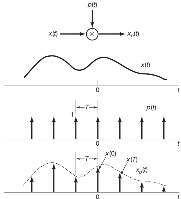
Figura 7.2 Amostragem com trem de impulsos.
