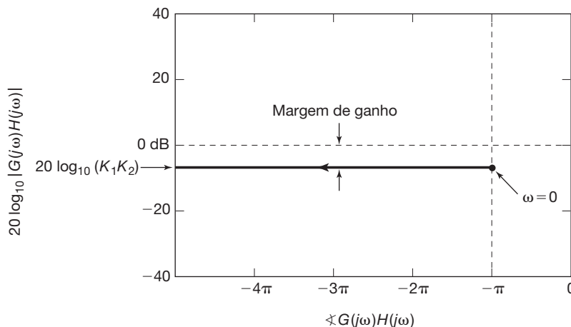
Figura 11.32 Gráfico logarítmico de magnitude-fase para o Exemplo 11.12.
