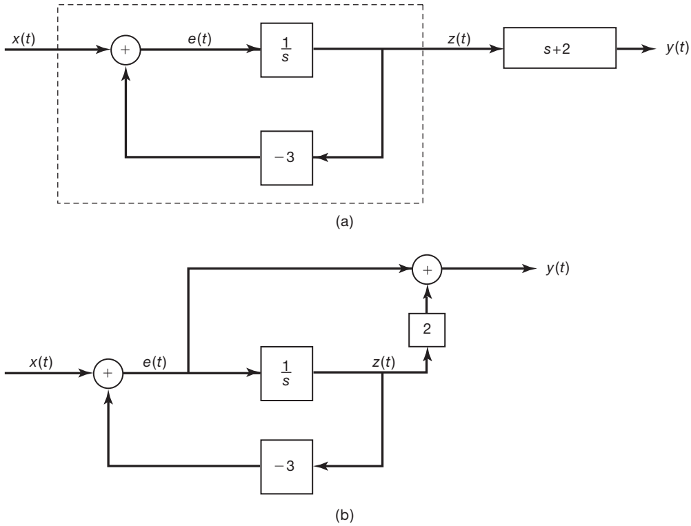
Figura 9.33 (a) Representações por diagrama de blocos para o sistema do Exemplo 9.29. (b) Representação por diagrama de blocos equivalente.
