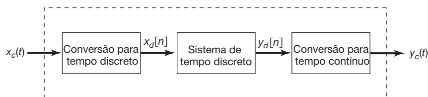
Figura 7.19 Processamento de tempo discreto de sinais de tempo contínuo.
