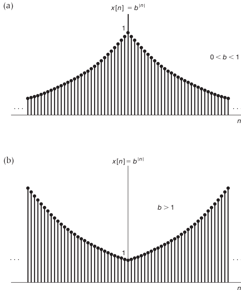
Figura 10.10 Sequência x[n] = b^{|n|} para 0 < b < 1 e para b > 1 : (a) b = 0,95 ; (b) b = 1,05 .
