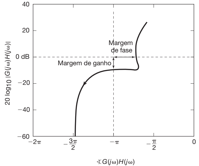
Figura 11.28 Gráfico logarítmico de magnitude-fase para o sistema do Exemplo 11.9.
