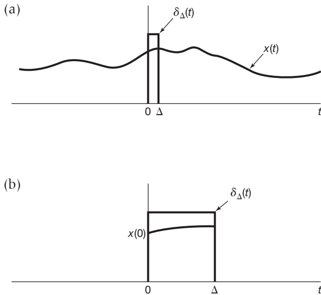
Figura 1.39 O produto x(t)\delta_\Delta(t) : (a) gráficos das duas funções; (b) visão ampliada da porção diferente de zero de seu produto.
