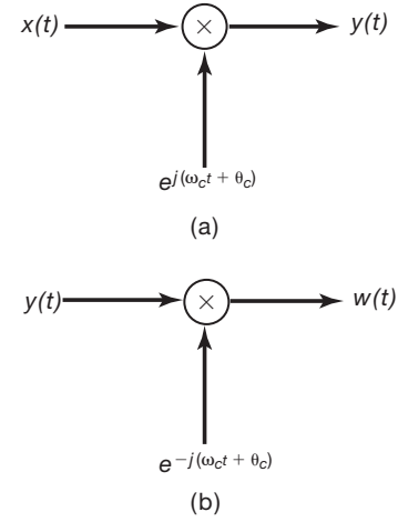
Figura 8.7 Sistema para modulação e demodulação em amplitude usando uma portadora exponencial complexa: (a) modulação; (b) demodulação.
