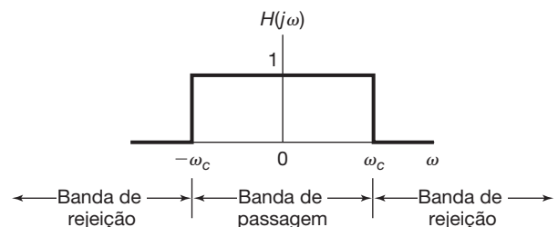
Figura 3.26 Resposta em frequência de um filtro passa-baixas ideal.
