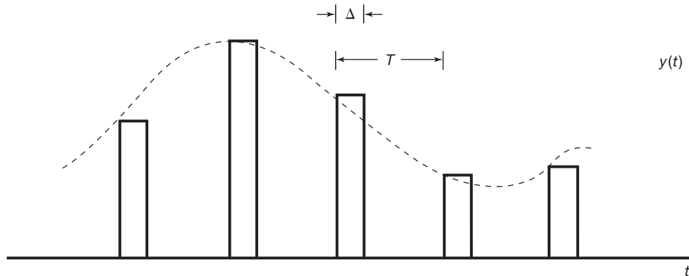
Figura 8.26 Forma de onda transmitida para um único canal PAM. A curva tracejada representa o sinal x(t) .
