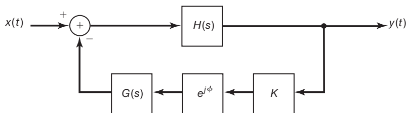
Figura 11.26 Sistema com realimentação contendo possíveis desvios de ganho e fase da descrição nominal representada na Figura 11.25.
