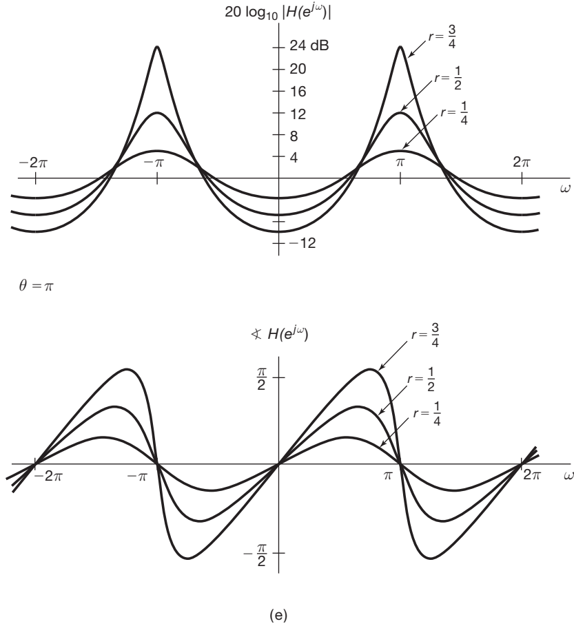
Figura 6.31 Magnitude e fase da resposta em frequência do sistema de segunda ordem da Equação 6.57: (a) \theta = 0 ; (b) \theta = \pi/4 ; (c) \theta = \pi/2 ; (d) \theta = 3\pi/4 ; (e) \theta = \pi . Cada gráfico contém curvas correspondentes a r = 1/4 , 1/2 e 3/4 .
