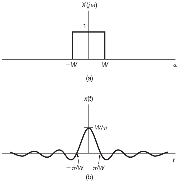
Figura 4.9 Par transformado de Fourier do Exemplo 4.5: (a) Transformada de Fourier do Exemplo 4.5. (b) A função de tempo correspondente.
