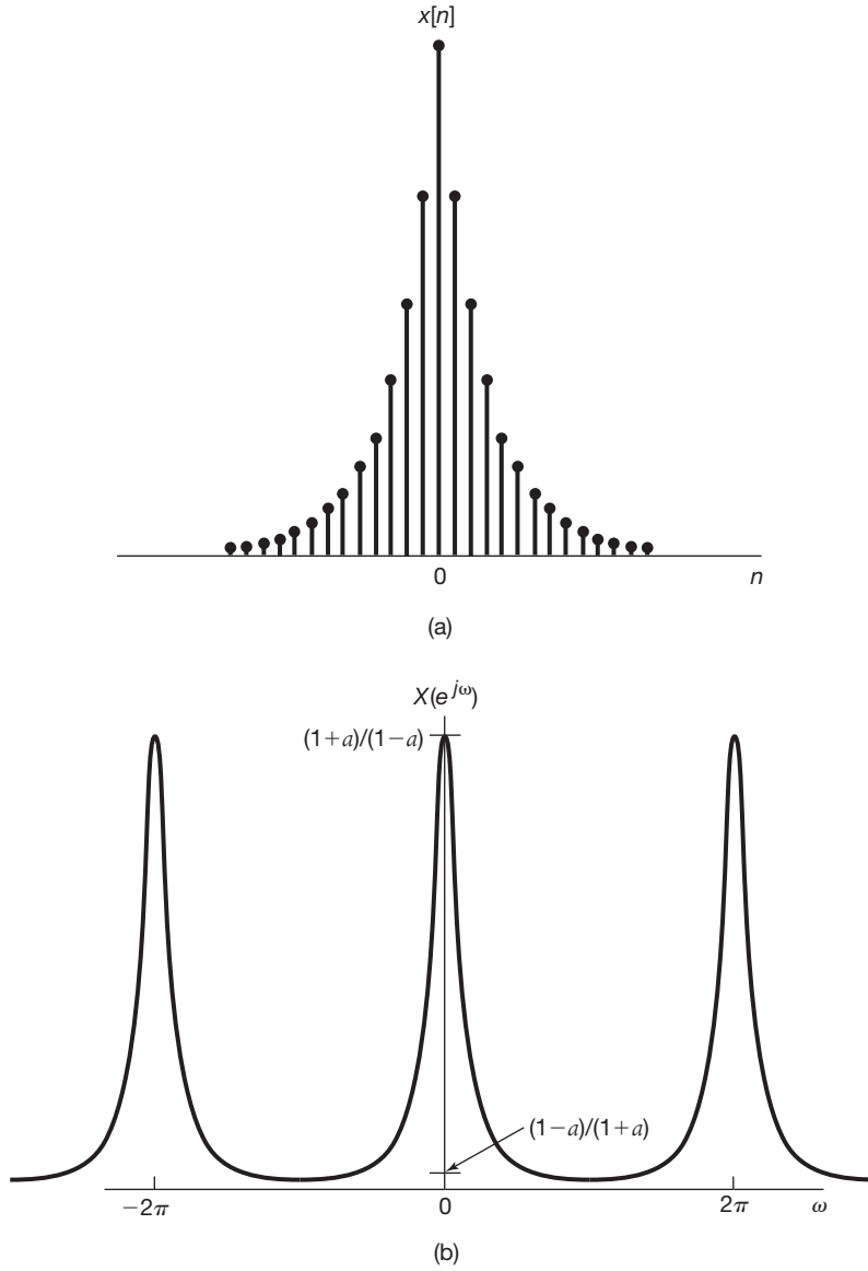
Figura 5.5 (a) Sinal x[n] = a^{|n|} do Exemplo 5.2 e (b) sua transformada de Fourier ( 0 < a < 1 ).
