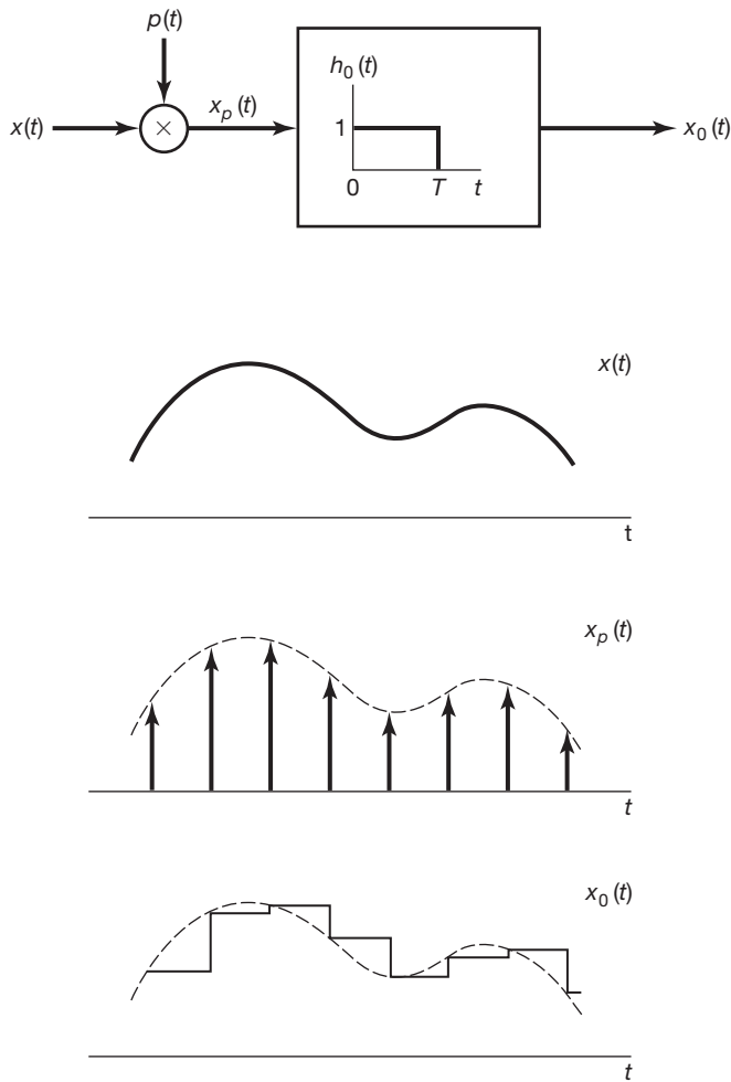
Figura 7.6 Retentor de ordem zero como amostragem por trem de impulsos seguido por um sistema LIT com um pulso retangular com a resposta impulsiva.
