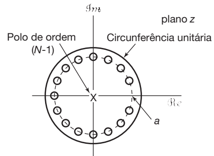
Figura 10.9 Localização dos polos e zeros para o Exemplo 10.6 com N = 16 e 0 < a < 1 . A região de convergência para esse exemplo consiste em todos os valores de z , exceto z = 0 .
