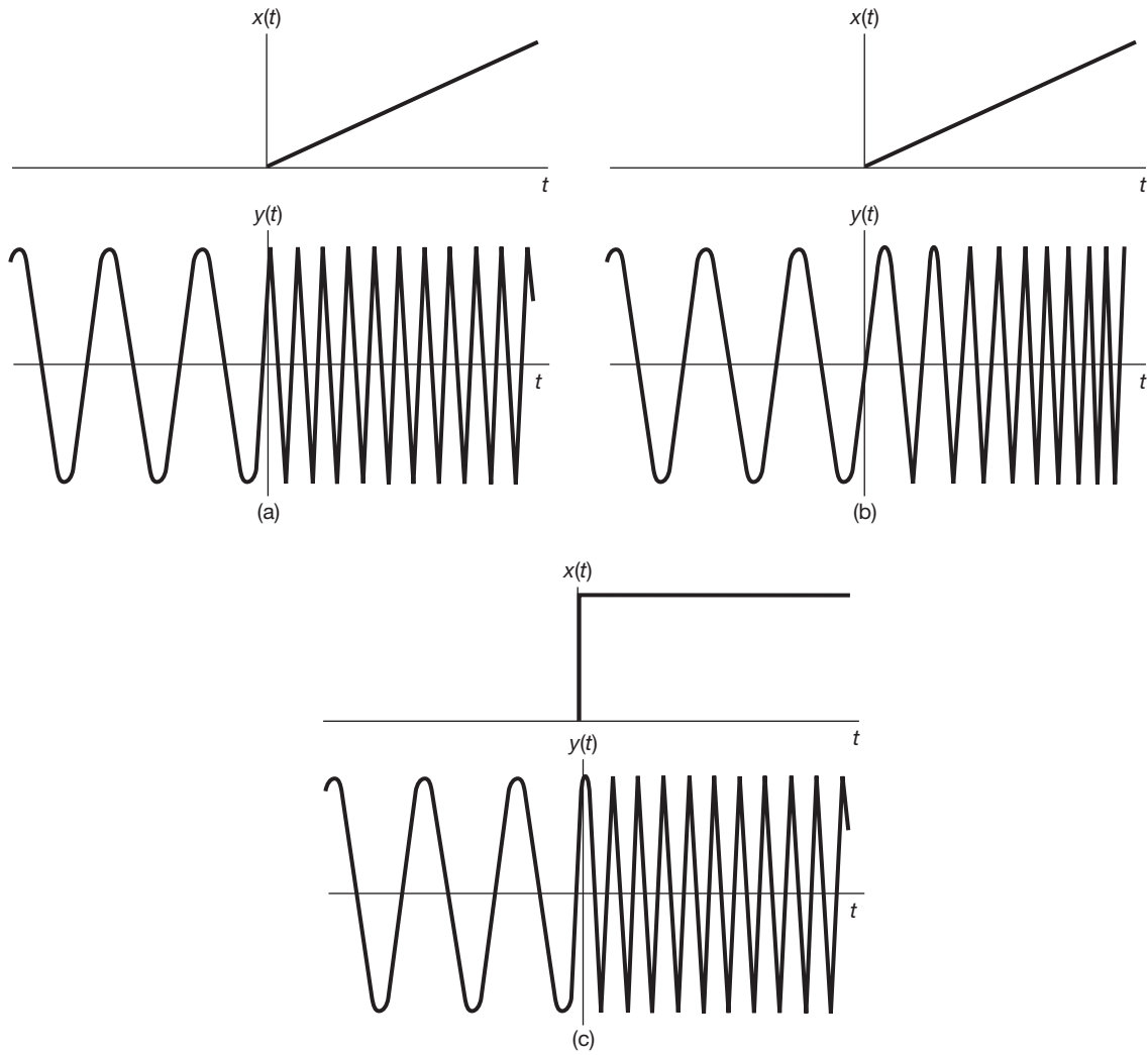
Figura 8.32 Modulação em fase, modulação em frequência e sua relação: (a) modulação em fase com uma rampa como sinal modulante; (b) modulação em frequência com uma rampa como sinal modulante; (c) modulação em frequência com um degrau (a derivada de uma rampa) como sinal modulante.
