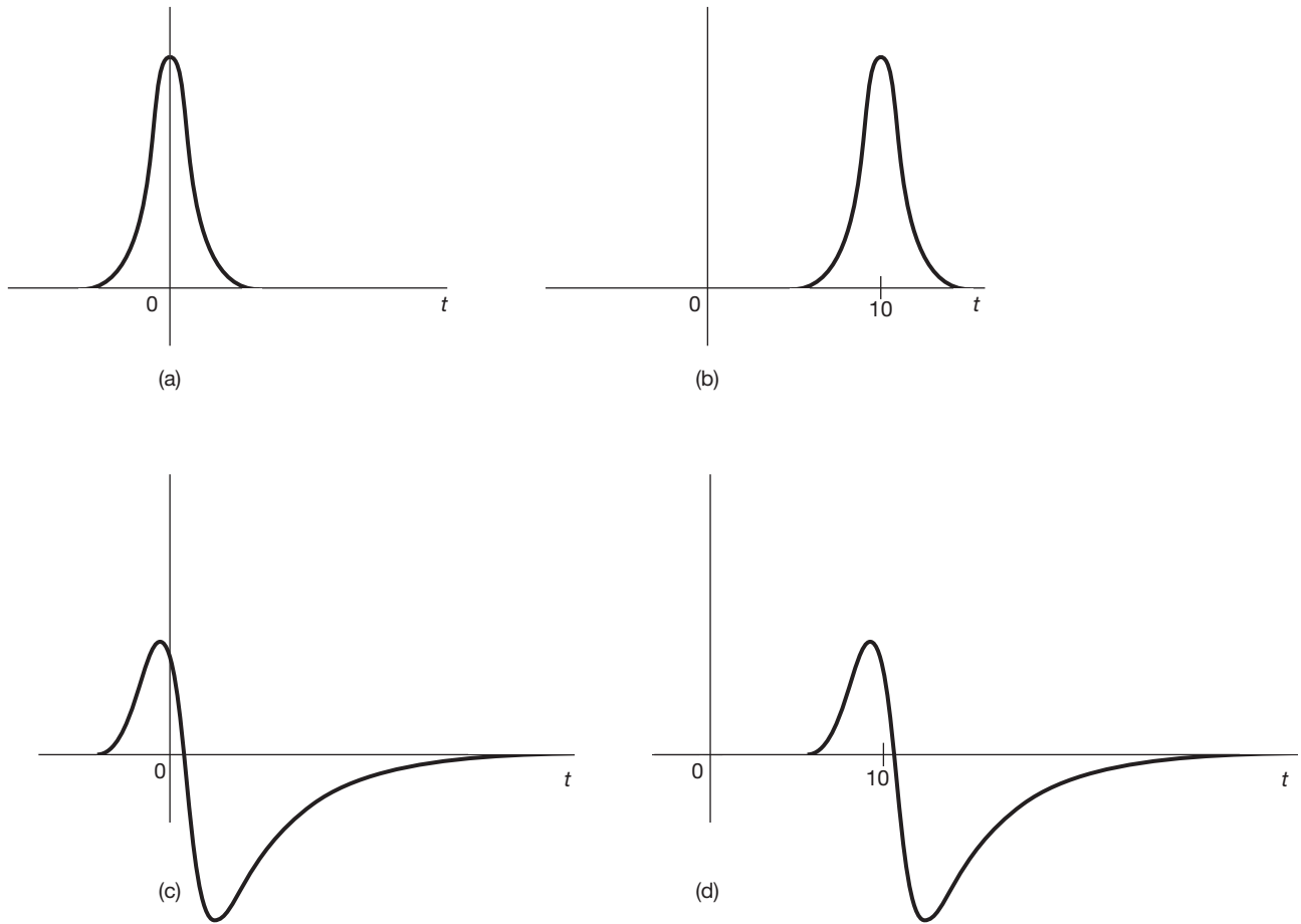
Figura 6.3 (a) Sinal de tempo contínuo, que é aplicado como entrada para diversos sistemas para os quais a resposta em frequência tem magnitude unitária; (b) resposta para um sistema com fase linear; (c) resposta para um sistema com fase não linear; (d) resposta para um sistema com fase igual à fase não linear do sistema no item (c) mais um termo de fase linear.
