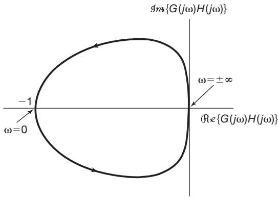
Figura 11.22 Diagrama de Nyquist para o Exemplo 11.6. A seta na curva indica a direção de \omega crescente.
