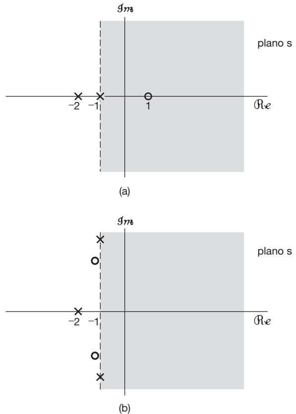
Figura 9.2 Representação no plano s das transformadas de Laplace para o (a) Exemplo 9.3 e para o (b) Exemplo 9.4. Cada 'x' nessas figuras indica a localização de um polo da transformada de Laplace correspondente, ou seja, uma raiz do denominador. De modo semelhante, cada 'o' nessas figuras indica um zero, ou seja, uma raiz do numerador. As regiões sombreadas indicam as RDCs.
