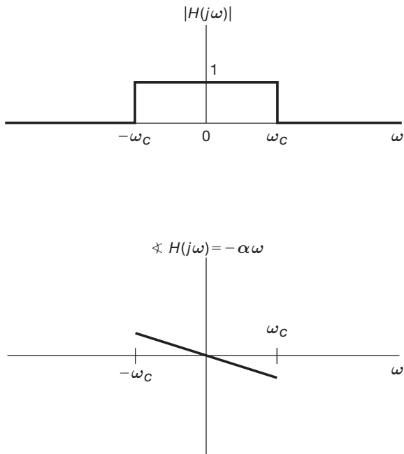
Figura 6.11 Filtro passa-baixas ideal de tempo contínuo com característica de fase linear.
