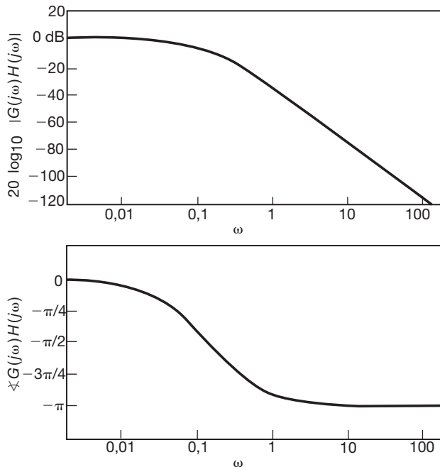
Figura 11.20 Diagrama de Bode para G(j\omega)H(j\omega) no Exemplo 11.5.
