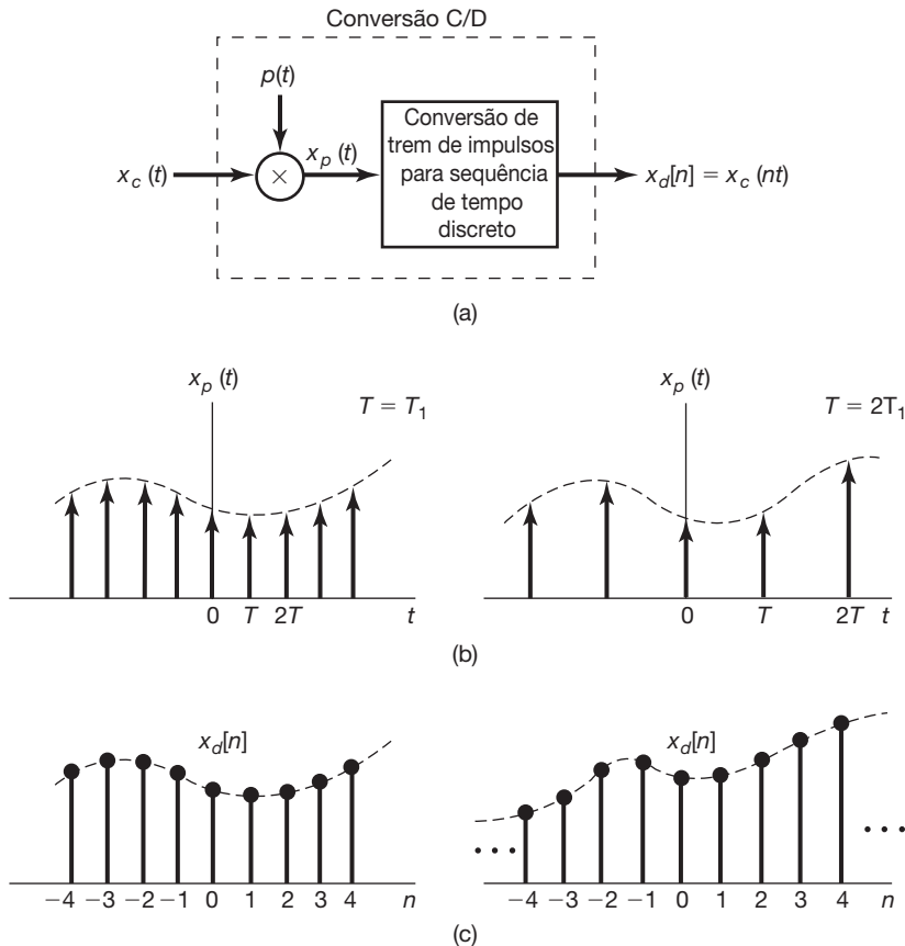
Figura 7.21 Amostragem com um trem de impulsos periódico, seguida pela conversão para uma sequência de tempo discreto: (a) sistema total; (b) x_p(t) para duas taxas de amostragem. A envoltória tracejada representa x_c(t) ; (c) a sequência de saída para duas taxas de amostragem diferentes.
