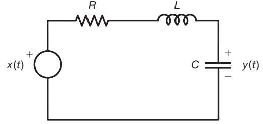
Figura 9.27 Um circuito RLC série.
