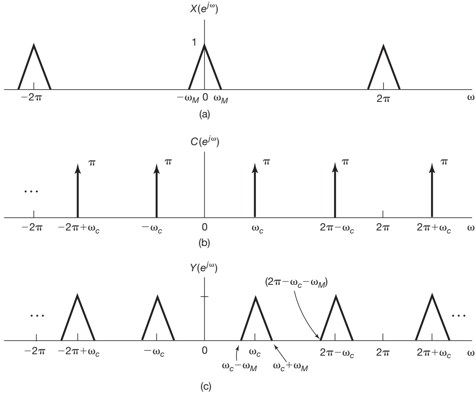
Figura 8.42 Espectros associados à modulação de tempo discreto usando uma portadora senoidal: (a) espectro de um sinal de banda limitada x[n] ; (b) espectro de um sinal de portadora senoidal c[n] = \cos \omega_c n ; (c) espectro do sinal modulado y[n] = x[n]c[n] .
