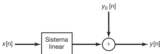
Figura 1.48 Estrutura de um sistema linear incremental. Aqui, y_0[n] é a resposta à entrada nula do sistema.
