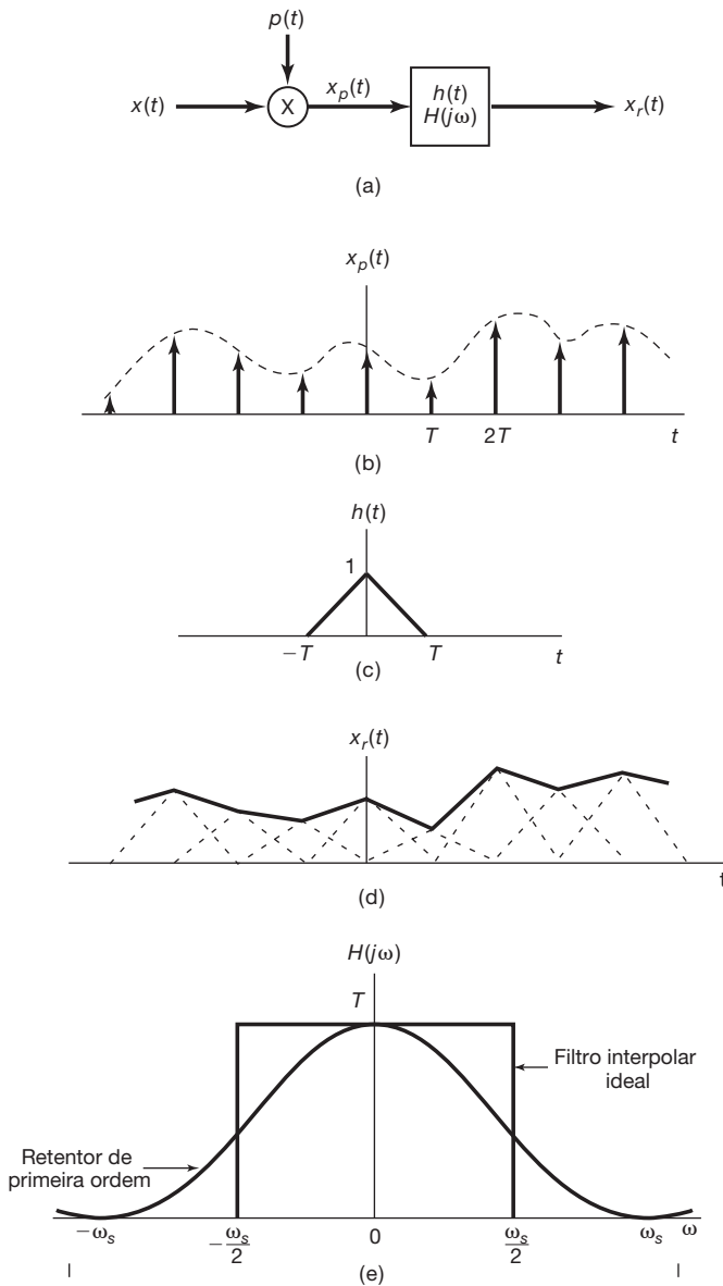
Figura 7.13 Interpolação linear (retentor de primeira ordem) como amostragem por trem de impulsos seguida pela convolução com uma resposta ao impulso triangular. (a) Sistema para amostragem e reconstrução. (b) Trem de impulsos ponderados pelas amostras. (c) Resposta ao impulso representando um retentor de primeira ordem. (d) Retentor de primeira ordem aplicado ao sinal amostrado. (e) Comparação da função de transferência do filtro interpolador ideal e retentor de primeira ordem.
