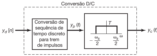
Figura 7.23 Conversão de uma sequência de tempo discreto para um sinal de tempo contínuo.
