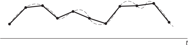
Figura 7.9 Interpolação linear entre os pontos das amostras. A curva tracejada representa o sinal original, e a curva sólida, a interpolação linear.
