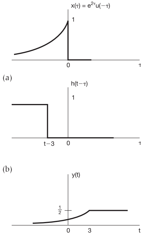
Figura 2.22 Problema de convolução considerado no Exemplo 2.8.
