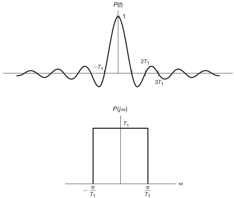
Figura 8.29 O pulso sinc e seu espectro correspondente.
