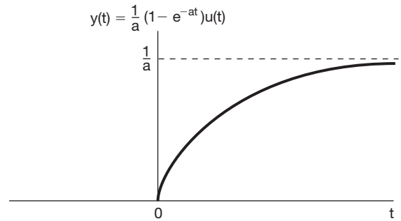
Figura 2.18 Resposta do sistema no Exemplo 2.6 com resposta ao impulso h(t) = u(t) para a entrada x(t) = e^{-at}u(t) .
