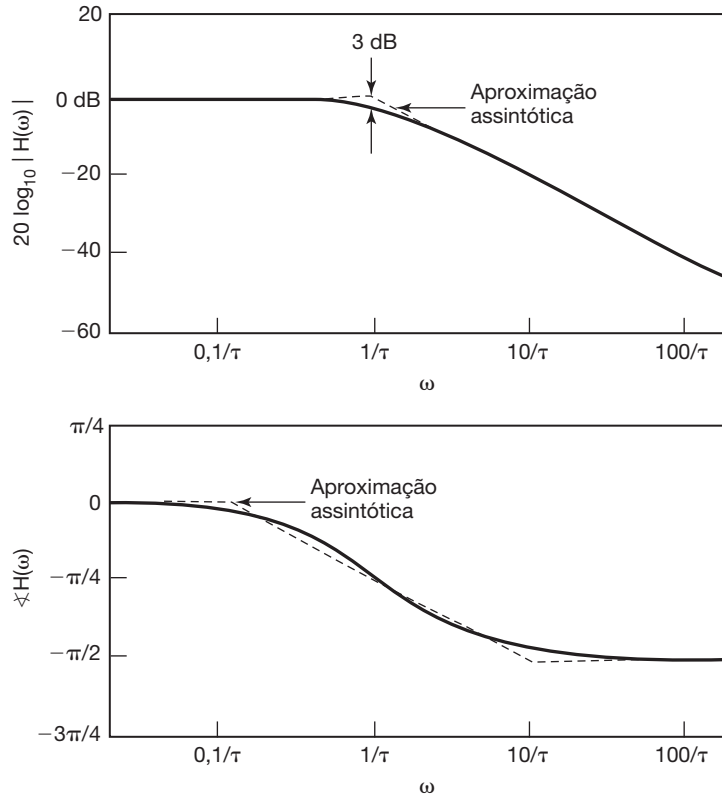
Figura 9.18 Resposta em frequência para um sistema de primeira ordem.
