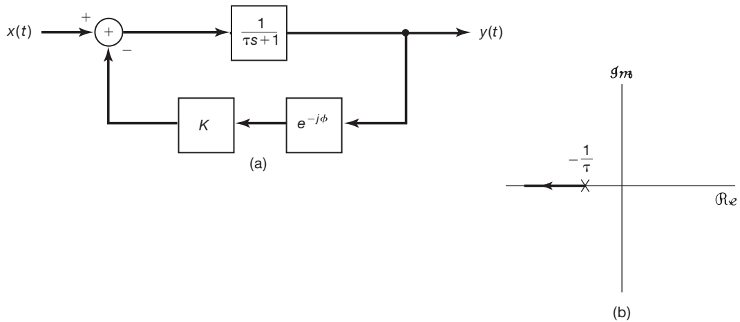
Figura 11.30 (a) Sistema com realimentação de primeira ordem com variações possíveis de ganho e fase no caminho de realimentação. (b) Lugar das raízes para este sistema com \phi = 0 , K > 0 .
