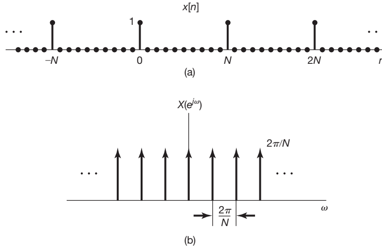
Figura 5.11 (a) Trem de impulsos periódico de tempo discreto; (b) sua transformada de Fourier.
