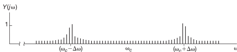
Figura 8.39 Magnitude do espectro para \omega > 0 correspondente à modulação em frequência com um sinal modulante onda quadrada periódica. Cada uma das linhas verticais na figura representa um impulso de área proporcional à altura da linha.
