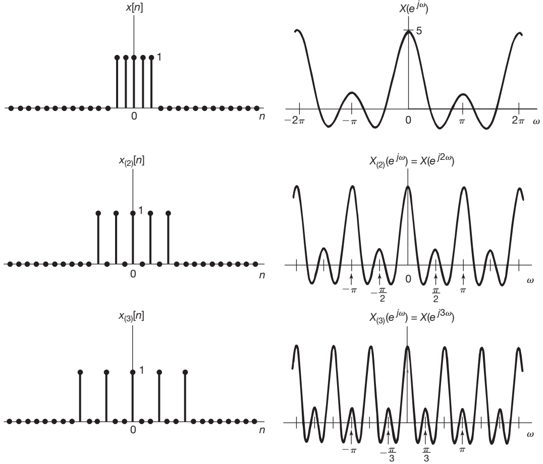
Figura 5.14 Relação inversa entre os domínios de tempo e frequência: conforme k aumenta, x_{(k)}[n] espalha-se enquanto sua transformada é comprimida.
