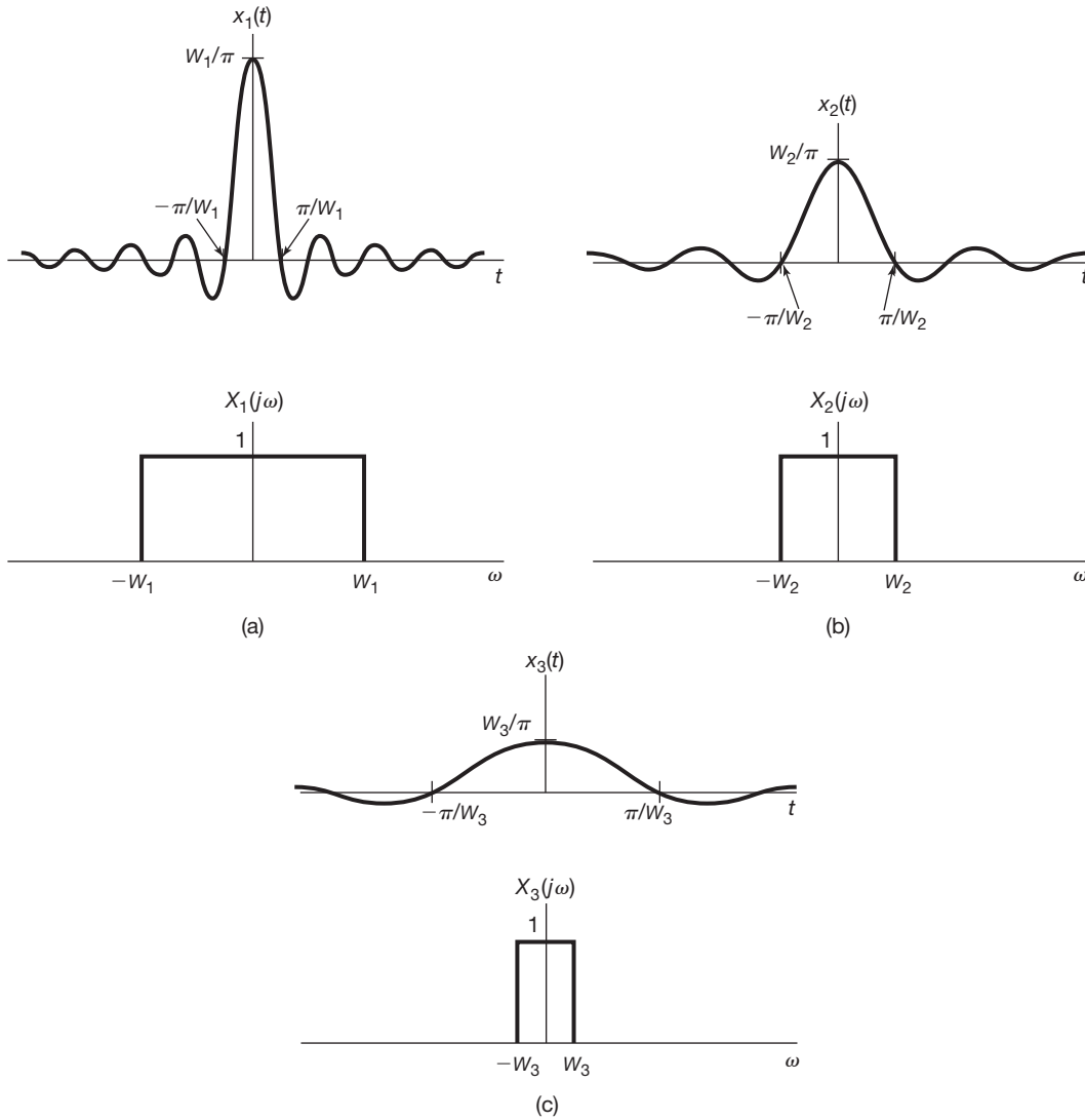
Figura 4.11 Par transformado de Fourier da Figura 4.9 para diferentes valores de W .
