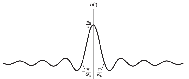
Figura 4.21 Resposta ao impulso de um filtro passa-baixas ideal do Exemplo 4.18.
