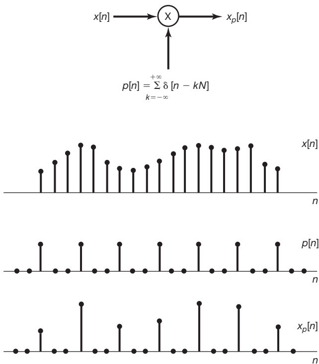
Figura 7.31 Amostragem de tempo discreto.
