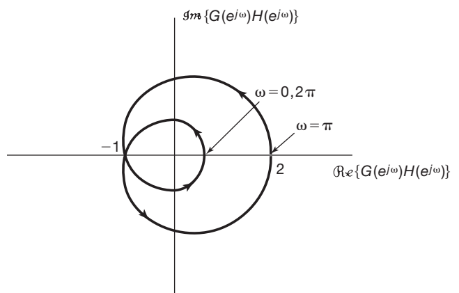
Figura 11.24 Diagrama de Nyquist para o Exemplo 11.8. A seta na curva indica a direção em que a curva é percorrida à medida que \omega aumenta de 0 a 2\pi .
