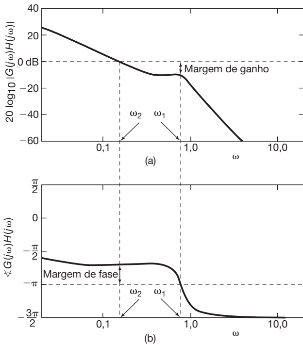
Figura 11.27 Uso de diagramas de Bode para calcular margens de ganho e de fase para o sistema do Exemplo 11.9.
