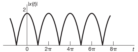
Figura 1.22 Sinal senoidal retificado em onda completa do Exemplo 1.5.
