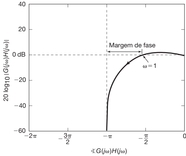
Figura 11.31 Gráfico logarítmico de magnitude-fase para o sistema de segunda ordem do Exemplo 11.11.
