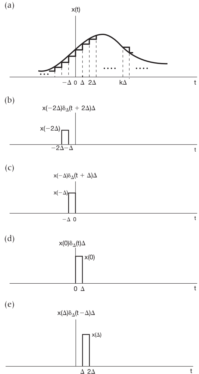
Figura 2.12 Aproximação em degraus para um sinal de tempo contínuo.
