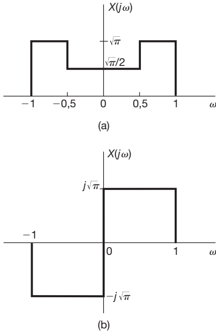
Figura 4.18 As transformadas de Fourier consideradas no Exemplo 4.14.
