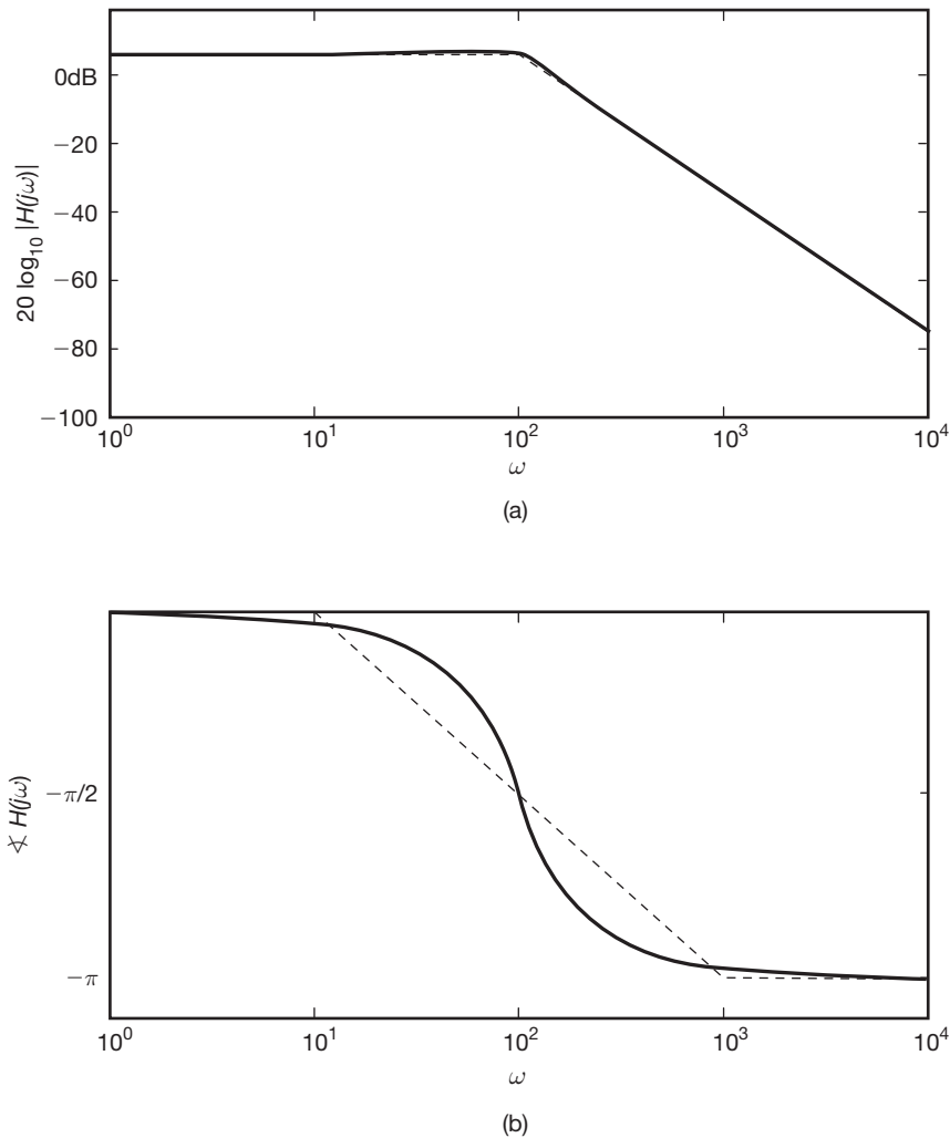
Figura 6.24 Diagrama de Bode para a função de sistema no Exemplo 6.4: (a) magnitude; (b) fase.
