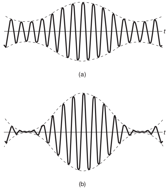
Figura 8.13 Saída do sistema de modulação de amplitude da Figura 8.12: (a) índice de modulação m = 0,5 ; (b) índice de modulação m = 1,0 .
