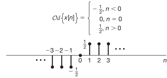
Figura 1.18 Exemplo de decomposição par-ímpar de um sinal de tempo discreto.
