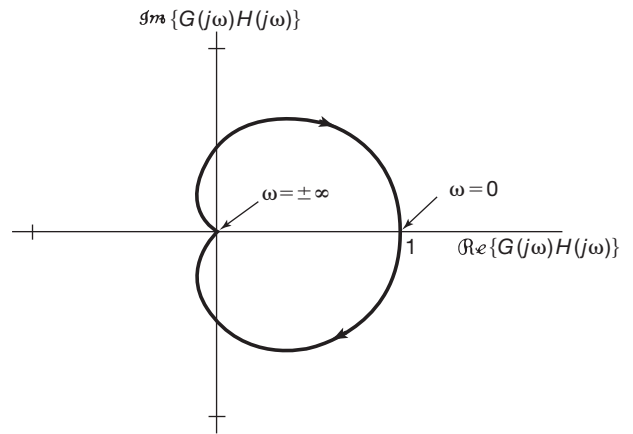
Figura 11.21 Diagrama de Nyquist de G(j\omega)H(j\omega) para o Exemplo 11.5. A seta na curva indica a direção de \omega crescente.
