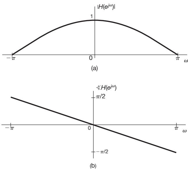
Figura 3.25 (a) Magnitude e (b) fase da resposta em frequência do sistema LIT de tempo discreto y[n] = 1/2(x[n] + x[n-1]) .
