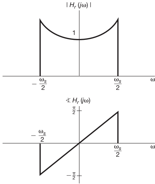
Figura 7.8 Magnitude e fase do filtro de reconstrução para um retentor de ordem zero.
