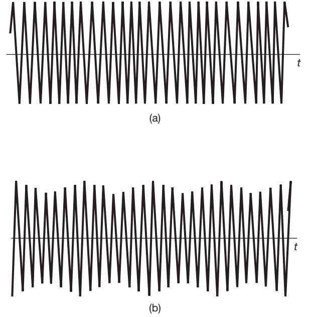
Figura 8.34 Comparação de FM de banda estreita e AM-DSB/WC: (a) FM de banda estreita; (b) AM-DSB/WC.
