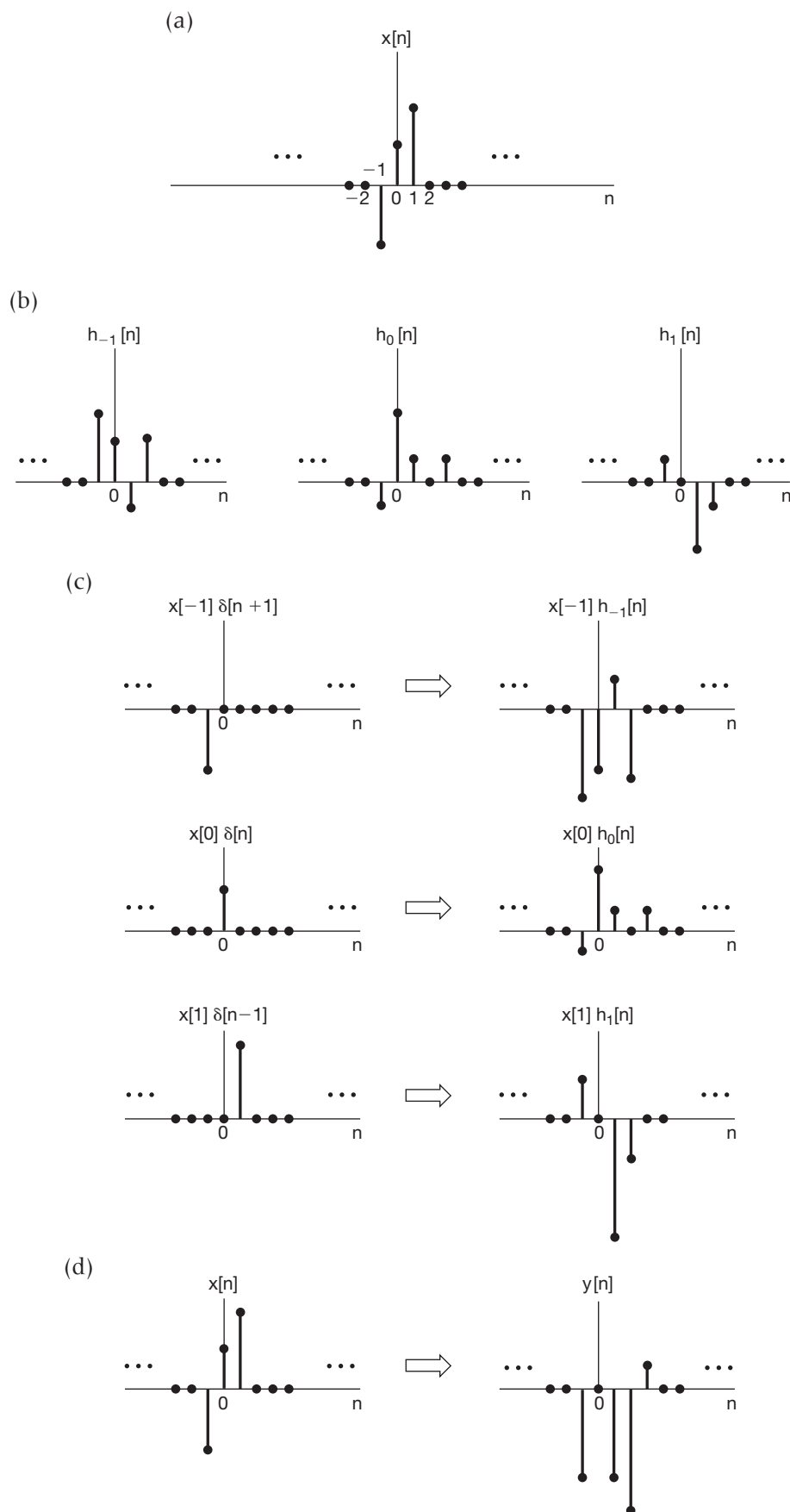
Figura 2.2 Interpretação gráfica da resposta de um sistema linear de tempo discreto conforme representado na Equação 2.3.
