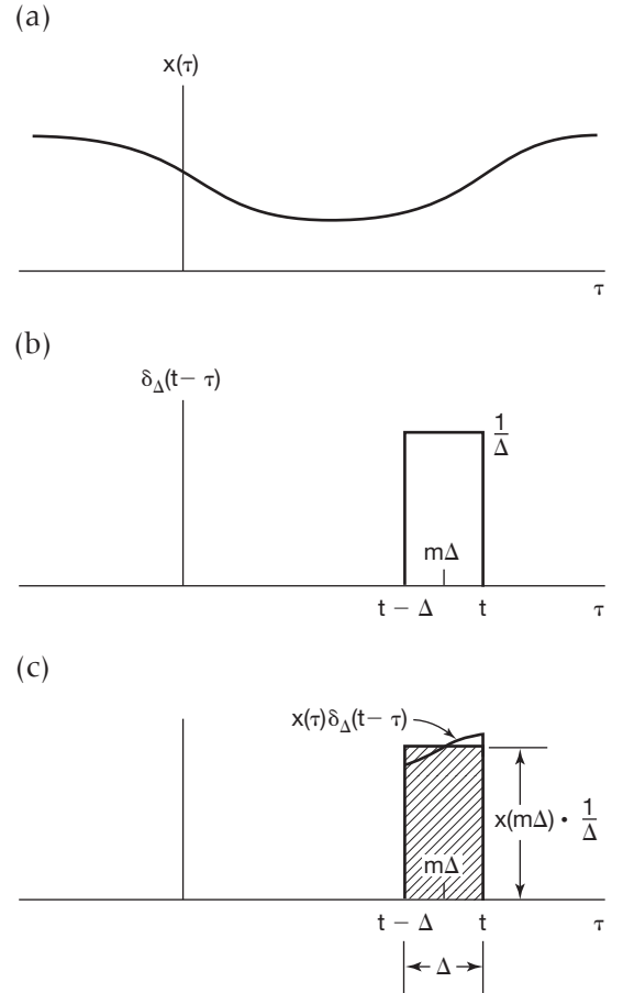
Figura 2.13 Interpretação gráfica da Equação 2.26.
