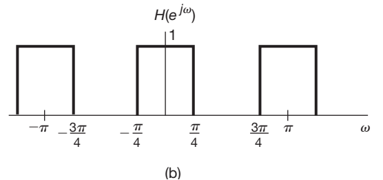
Figura 5.18 (a) Interconexão de sistemas do Exemplo 5.14; (b) a resposta em frequência geral para esse sistema.
