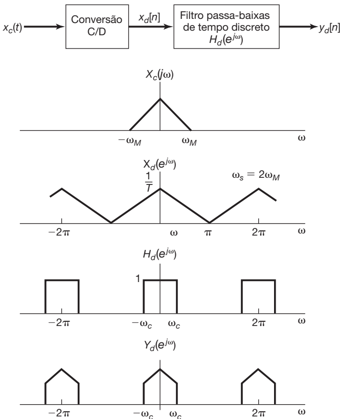
Figura 7.36 Sinal de tempo contínuo que foi amostrado originalmente na taxa de Nyquist. Após a filtragem de tempo discreto, a sequência resultante pode ser ainda subamostrada. Aqui, X_c(j\omega) é a transformada de Fourier de tempo contínuo de x_c(t) , X_d(e^{j\omega}) e Y_d(e^{j\omega}) são transformadas de Fourier de tempo discreto de x_d[n] e y_d[n] , respectivamente, e H_d(e^{j\omega}) é a resposta em frequência do filtro passa-baixas de tempo discreto representado no diagrama de blocos.
