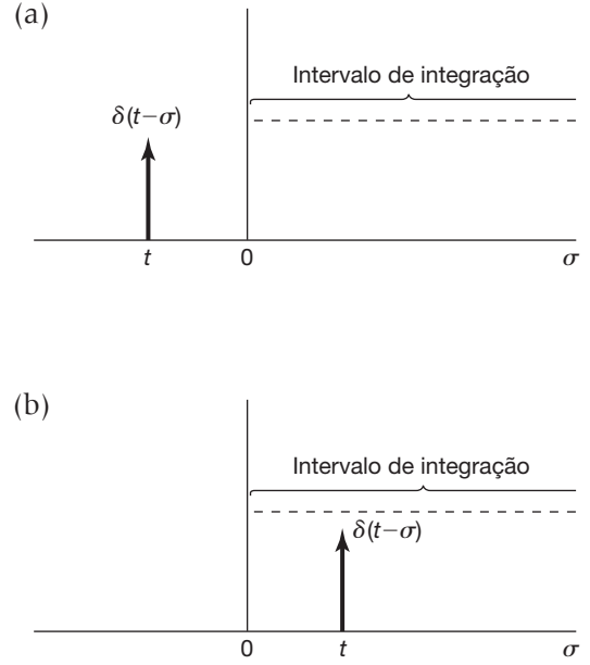
Figura 1.38 Relação dada na Equação 1.75; (a) t < 0 ; (b) t > 0 .
