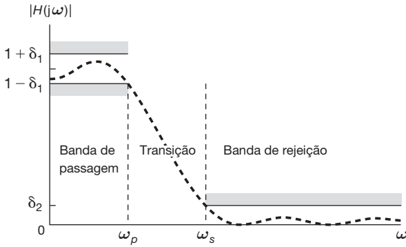
Figura 6.16 Tolerâncias para a característica de magnitude de um filtro passa-baixas. A ondulação permitida na banda de passagem é \delta_1 , e a ondulação permitida na banda de rejeição é \delta_2 . A curva tracejada ilustra uma resposta em frequência possível que permanece dentro dos limites toleráveis.
