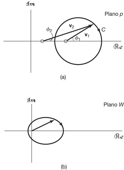
Figura 11.17 Propriedade de mapeamento básica. A curva fechada em (b) representa um gráfico dos valores de W(p) para valores de p ao longo da curva C em (a). Aqui, a seta na curva C em (a) indica a direção em que C é percorrida, e a seta em (b) indica a direção correspondente ao longo do contorno de valores de W(p) .
