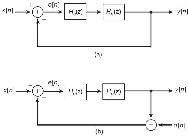
Figura 11.7 (a) Sistema de rastreamento de tempo discreto. (b) Sistema de rastreamento de (a) com distúrbio d[n] no caminho de realimentação considerando a presença de erros de medida.
