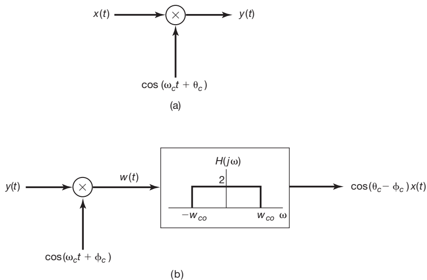
Figura 8.9 Sistema de modulação e demodulação em amplitude senoidal para a qual os sinais da portadora no modulador e no demodulador não estão sincronizados: (a) modulador; (b) demodulador.
