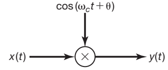
Figura 8.3 Modulação de amplitude com uma portadora senoidal.
