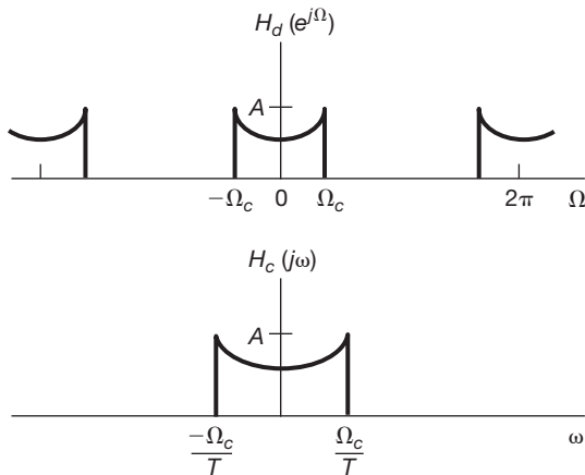
Figura 7.26 Resposta em frequência de tempo discreto e a resposta em frequência de tempo contínuo equivalente para o sistema da Figura 7.24.
