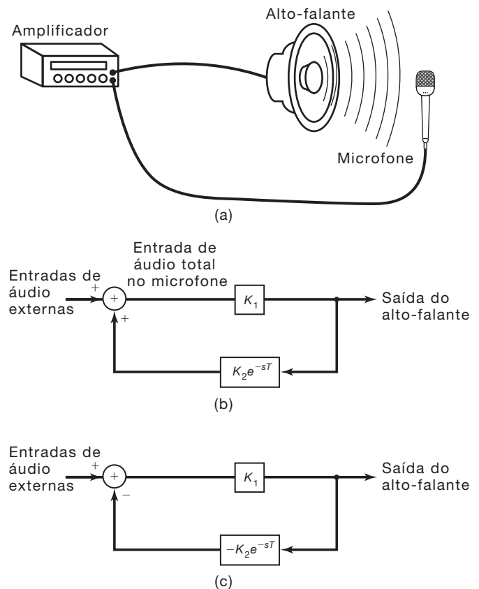
Figura 11.8 (a) Esquema do fenômeno da realimentação de áudio. (b) Representação em diagrama de blocos de (a). (c) Diagrama de blocos em (b) redesenhado como um sistema com realimentação negativa.
