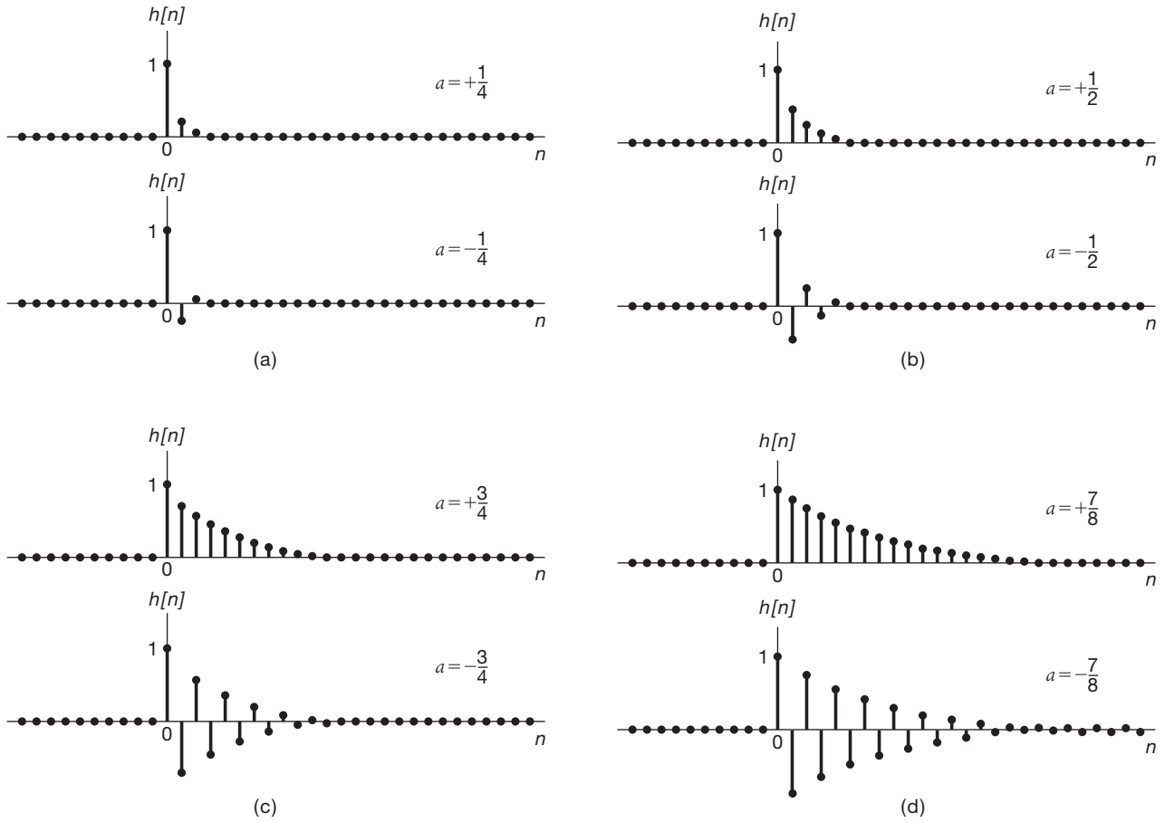
Figura 6.26 Resposta ao impulso h[n] = a^n u[n] de um sistema de primeira ordem: (a) a = \pm 1/4 ; (b) a = \pm 1/2 ; (c) a = \pm 3/4 ; (d) a = \pm 7/8 .
