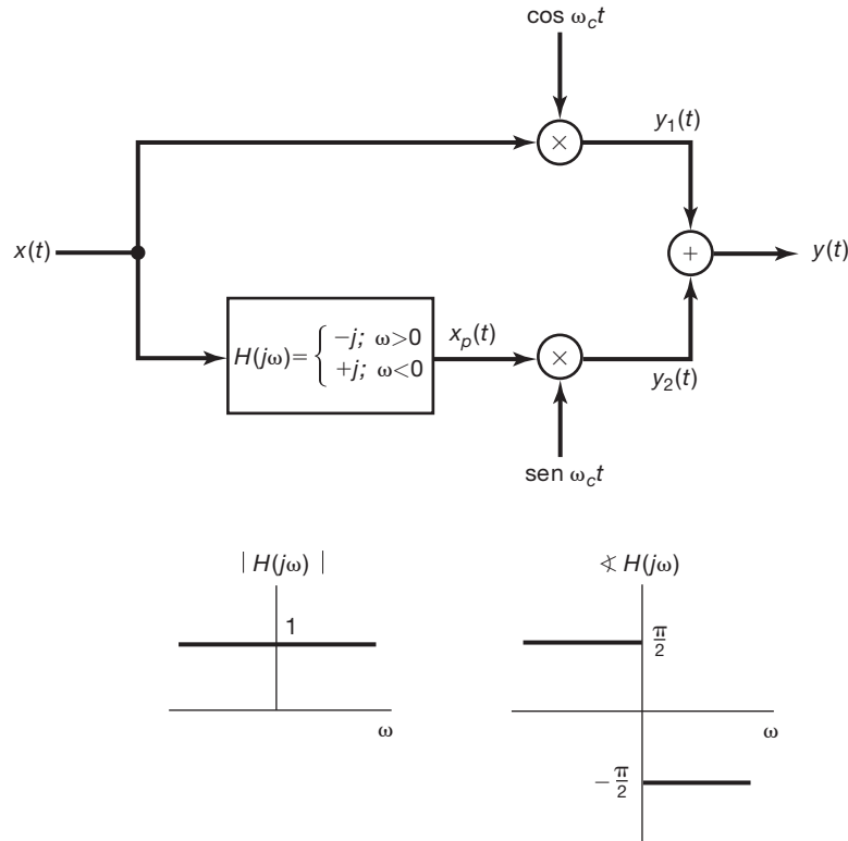
Figura 8.21 Sistema para modulação em amplitude de banda lateral única, usando rede de deslocamento de fase em 90^\circ , em que somente as bandas laterais inferiores são mantidas.
