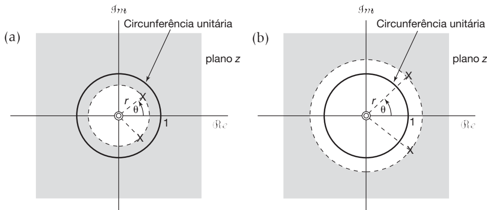
Figura 10.16 Diagrama de polos e zeros para um sistema de segunda ordem com polos complexos: (a) r < 1 ; (b) r > 1 , para o exemplo 10.24.
