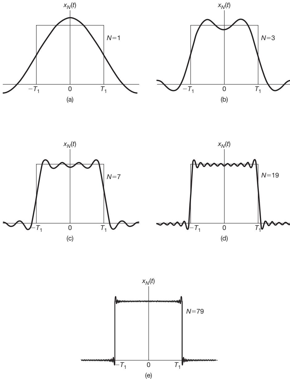
Figura 3.9 Convergência da representação em série de Fourier para uma onda quadrada: ilustração do fenômeno de Gibbs. Aqui, representamos uma aproximação de série finita x_N(t) = \sum_{k=-N}^N a_k e^{jk\omega_0 t} para diferentes valores de N .
