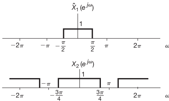
Figura 5.19 \hat{X}_1(e^{j\omega}) representando um período de X_1(e^{j\omega}) e X_2(e^{j\omega}) . A convolução linear de \hat{X}_1(e^{j\omega}) e X_2(e^{j\omega}) corresponde à convolução periódica de X_1(e^{j\omega}) e X_2(e^{j\omega}) .
