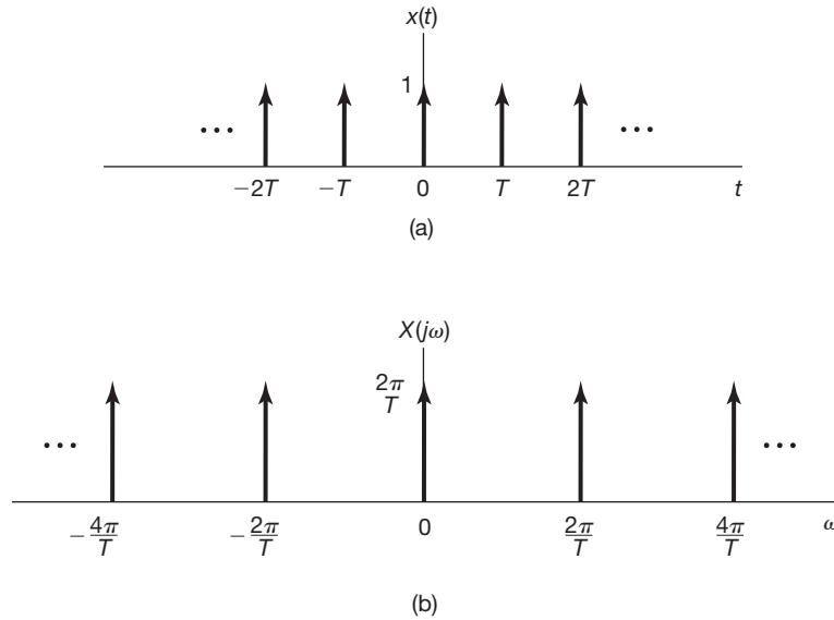
Figura 4.14 (a) Trem de impulsos periódico; (b) sua transformada de Fourier.
