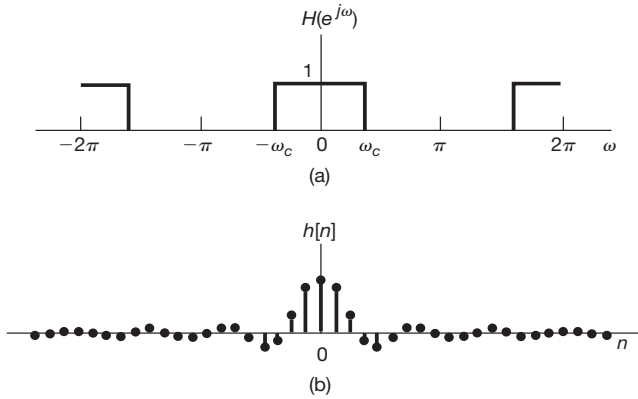
Figura 5.17 (a) Resposta em frequência de um filtro passa-baixas ideal de tempo discreto; (b) resposta ao impulso do filtro passa-baixas ideal.
