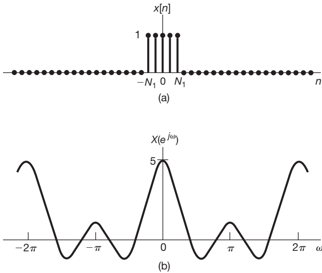
Figura 5.6 (a) Sinal de pulso retangular do Exemplo 5.3 para N_1 = 2 e (b) sua transformada de Fourier.
