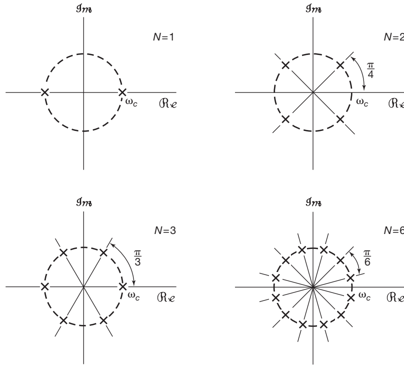
Figura 9.28 Localização dos polos de B(s)B(-s) para N=1, 2, 3 e 6 .
