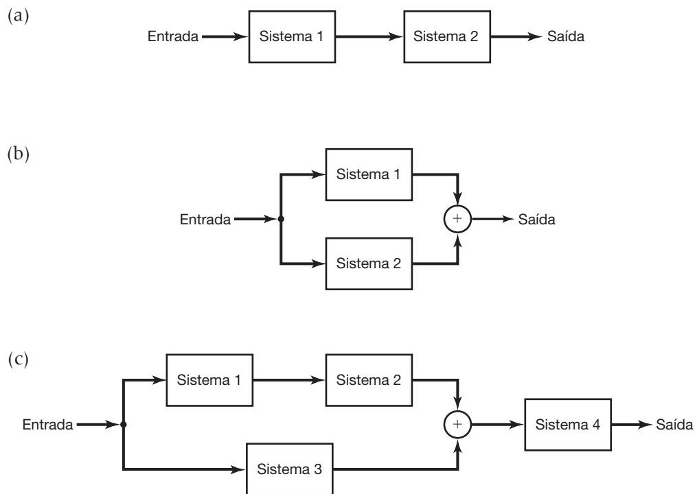
Figura 1.42 Interconexão de dois sistemas: (a) interconexão em série (cascata); (b) interconexão paralela; (c) interconexão série-paralela.
