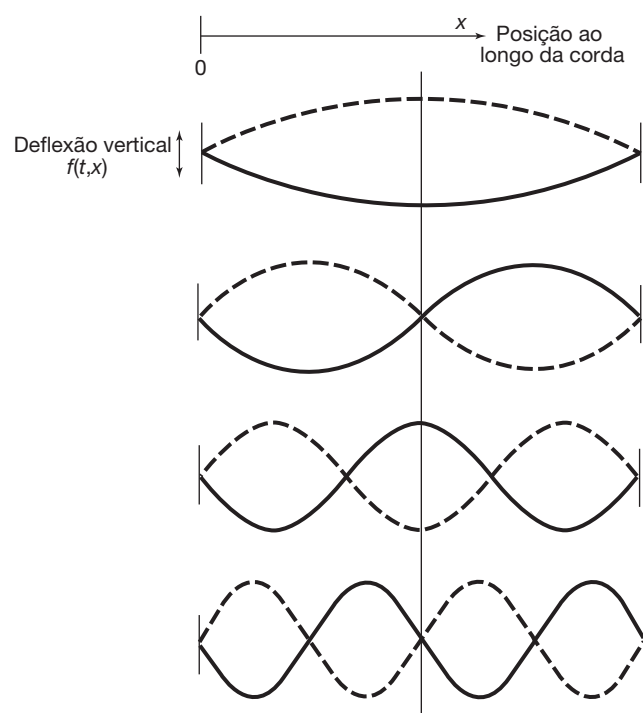
Figura 3.1 Modos normais de uma corda vibrante. (Linhas sólidas indicam a configuração de cada um desses modos em algum instante fixo no tempo, t .)
