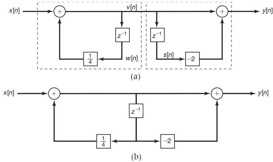
Figura 10.19 (a) Representações por diagrama de blocos para o sistema do Exemplo 10.29; (b) representação por diagrama de blocos usando apenas um elemento de atraso unitário.
