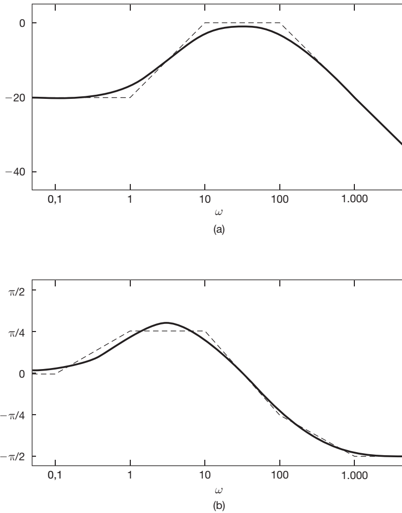
Figura 6.25 Diagrama de Bode para a função de sistema do Exemplo 6.5: (a) magnitude; (b) fase.
