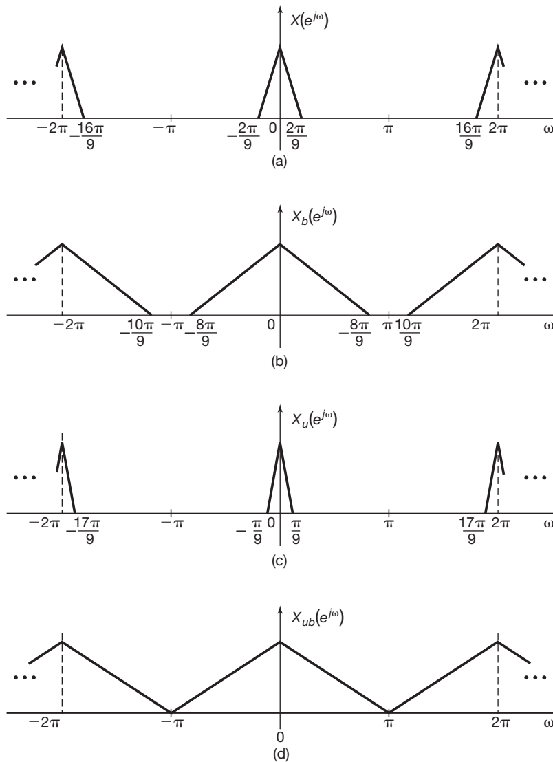
Figura 7.38 Espectros associados ao Exemplo 7.5. (a) Espectro de x[n] . (b) Espectro após subamostragem por 4. (c) Espectro após sobreamostragem de x[n] por um fator de 2. (d) Espectro após sobreamostragem de x[n] por 2 e depois, subamostragem por 9.
