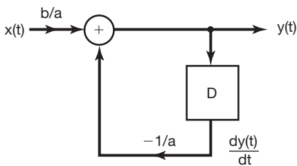
Figura 2.30 Representação em diagrama de blocos para o sistema nas equações 2.128 e 2.129 usando somadores, multiplicações por coeficientes e diferenciadores.
