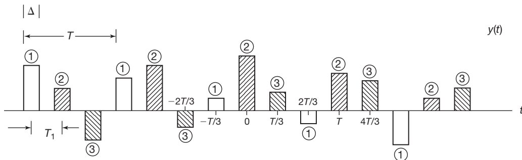
Figura 8.27 Forma de onda transmitida com três canais PAM multiplexados no tempo. Os pulsos associados a cada canal são distinguidos pelo sombreamento, além do número do canal acima de cada pulso. Aqui, o espaçamento entre símbolos é T_1 = T/3 .
