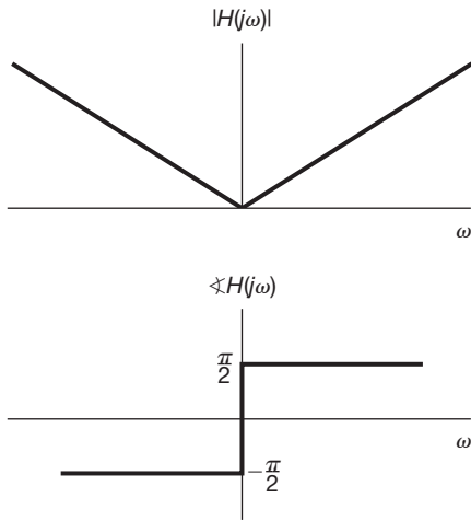
Figura 3.23 Características da resposta em frequência de um filtro para o qual a saída é a derivativa da entrada.
