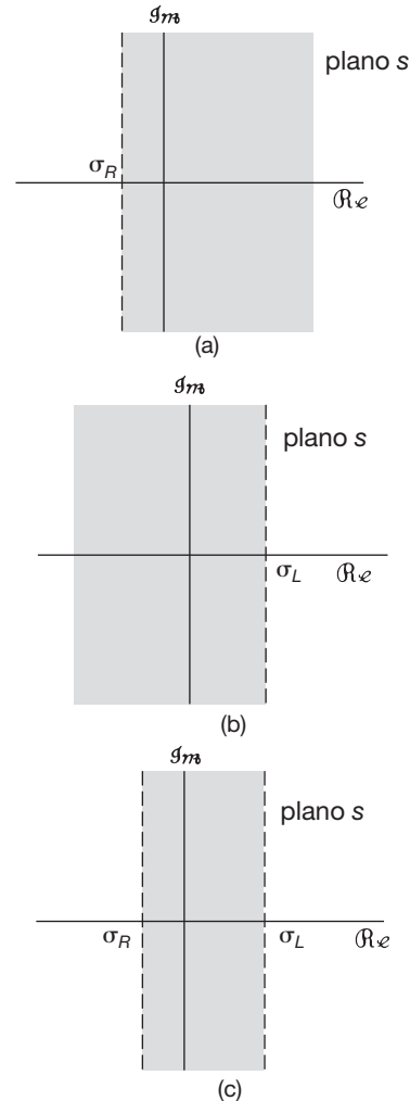
Figura 9.10 (a) RDC para x_R(t) da Figura 9.9. (b) RDC para x_L(t) da Figura 9.9. (c) A RDC para x(t) = x_R(t) + x_L(t) , supondo que as RDCs em (a) e (b) se sobrepõem.
