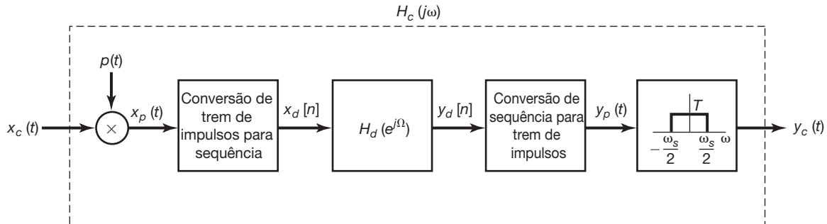
Figura 7.24 Sistema total para filtragem de um sinal de tempo contínuo usando um filtro de tempo discreto.
