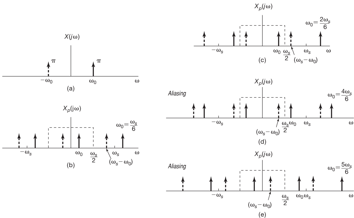
Figura 7.15 Efeito no domínio de frequência da sobreamostragem e subamostragem: (a) espectro do sinal senoidal original; (b), (c) espectro do sinal amostrado com \omega_s > 2\omega_0 ; (d), (e) espectro do sinal amostrado com \omega_s < 2\omega_0 . À medida que aumentamos \omega_0 passando de (b) para (d), os impulsos desenhados com linhas sólidas movem-se para a direita, enquanto os impulsos desenhados com linhas tracejadas se movem para a esquerda. Em (d) e (e), esses impulsos moveram-se de modo suficiente para que haja uma mudança naqueles que se encontram dentro da banda de passagem do filtro passa-baixas ideal.
