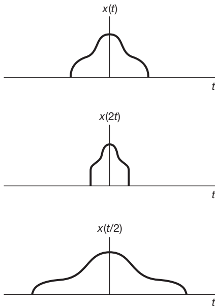
Figura 1.12 Sinais de tempo contínuo relacionados por mudança de escala no tempo.
