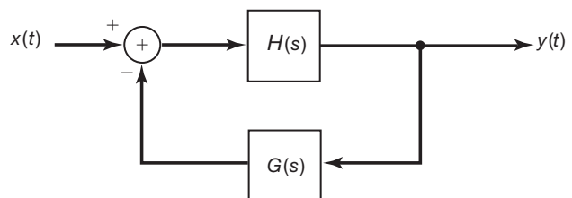
Figura 11.25 Sistema com realimentação típico projetado para ser estável considerando as descrições nominais para H(s) e G(s) .
