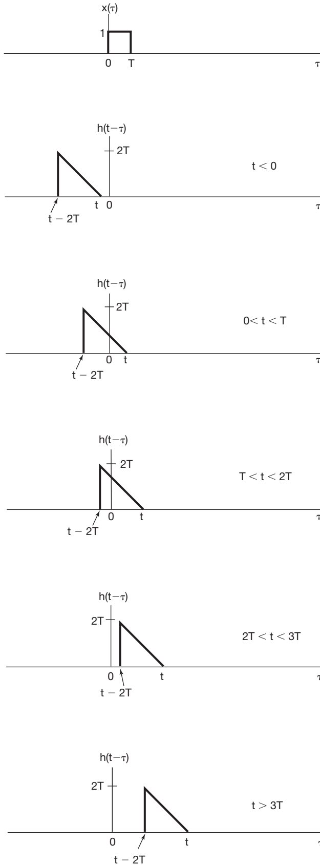
Figura 2.19 Sinais x(\tau) e h(t-\tau) para diferentes valores de t para o Exemplo 2.7.
