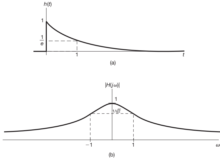
Figura 4.22 (a) Resposta ao impulso do sistema LIT da Equação 4.65; (b) magnitude da resposta em frequência do sistema.
