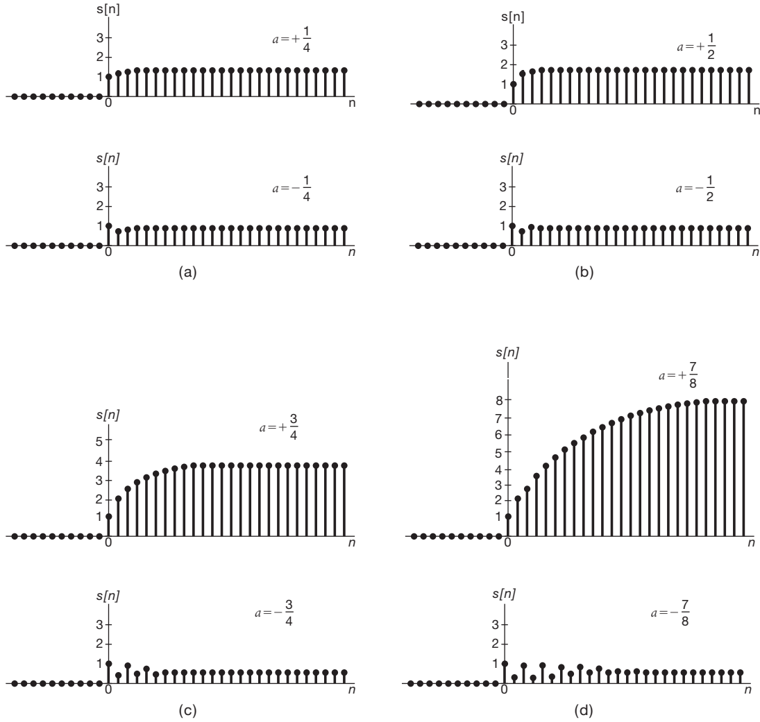
Figura 6.27 Resposta ao degrau s[n] de um sistema de primeira ordem: (a) a = \pm 1/4 ; (b) a = \pm 1/2 ; (c) a = \pm 3/4 ; (d) a = \pm 7/8 .
