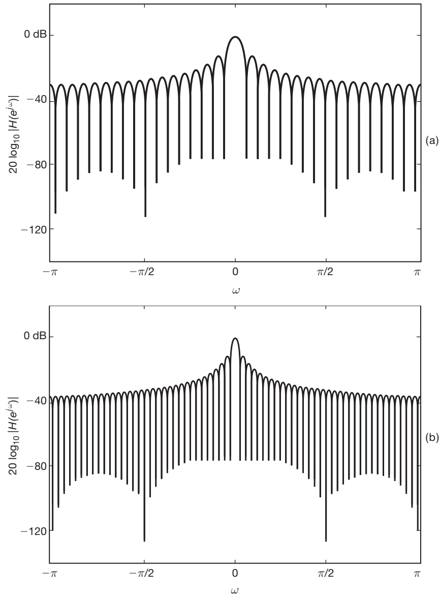
Figura 6.35 Gráficos do logaritmo da magnitude do filtro de média móvel das equações 6.78 e 6.79 para (a) M + N + 1 = 33 e (b) M + N + 1 = 65 .
