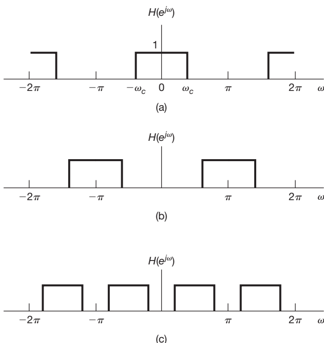
Figura 3.28 Filtros seletivos em frequência ideais de tempo discreto: (a) passa-baixas; (b) passa-altas; (c) passa-faixa.
