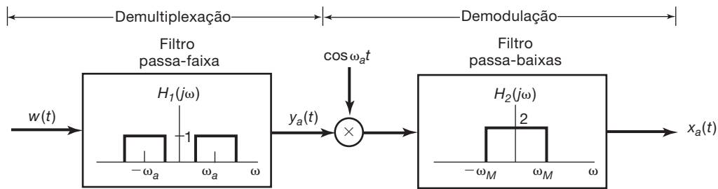
Figura 8.17 Demultiplexação e demodulação para um sinal multiplexado por divisão de frequência.
