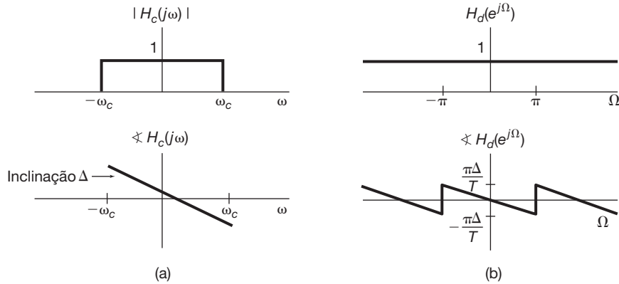
Figura 7.29 (a) Magnitude e fase da resposta em frequência para um atraso de tempo contínuo. (b) Magnitude e fase da resposta em frequência para o atraso de tempo discreto correspondente.
