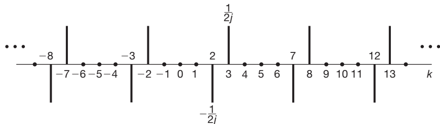
Figura 3.14 Coeficientes de Fourier para x[n] = \text{sen } 3(2\pi/5)n .
