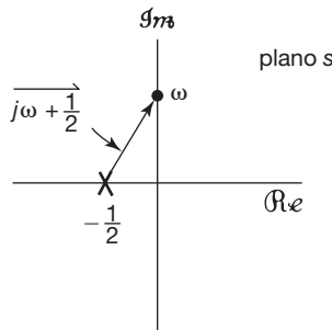
Figura 9.16 Diagrama de polos e zeros do Exemplo 9.12. |X(j\omega)| é o inverso do comprimento do vetor mostrado e \angle X(j\omega) é o negativo do ângulo do vetor.
