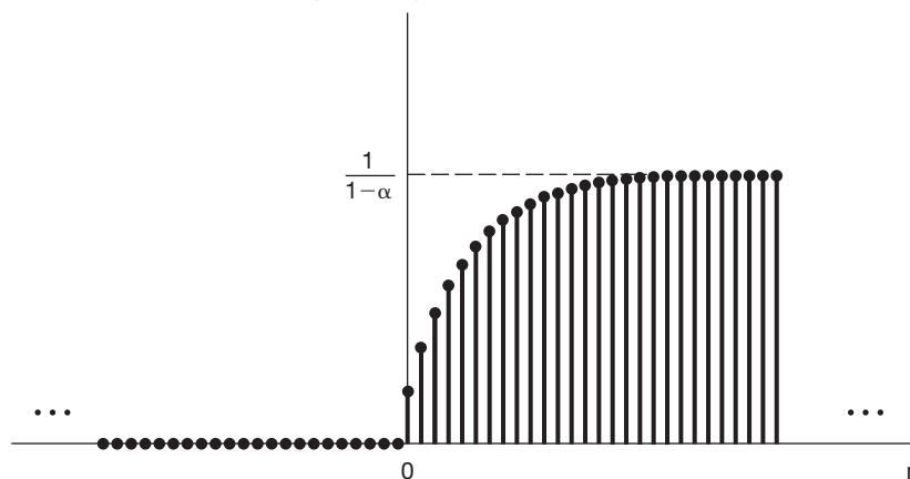
Figura 2.7 Saída para o Exemplo 2.3.
