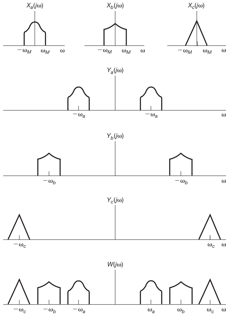
Figura 8.16 Espectros associados com o sistema de multiplexação por divisão de frequência da Figura 8.15.
