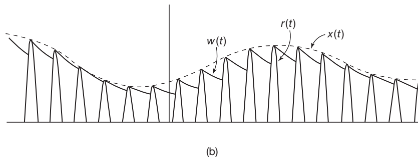
Figura 8.11 Demodulação por detecção de envoltória: (a) circuito para detecção de envoltória usando retificação de meia onda; (b) formas de onda associadas ao detector de envoltória em (a): r(t) é o sinal retificado em meia onda, x(t) é a envoltória verdadeira e w(t) é a envoltória obtida a partir do circuito em (a). A relação entre x(t) e w(t) foi exagerada em (b) para fins de ilustração. Em um sistema de demodulação assíncrona prático, w(t) tipicamente seria uma aproximação muito melhor para x(t) do que é representado aqui.
