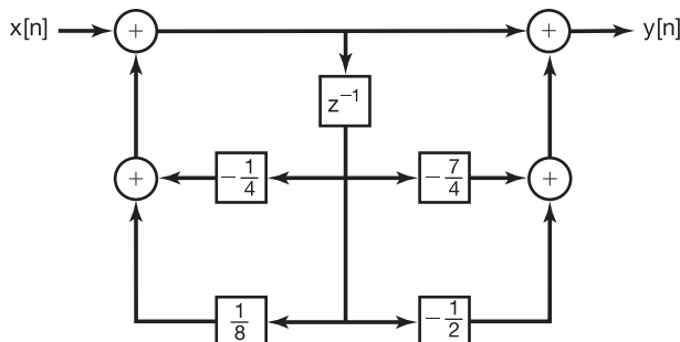
Figura 10.21 Representação na forma direta para o sistema do Exemplo 10.31.
