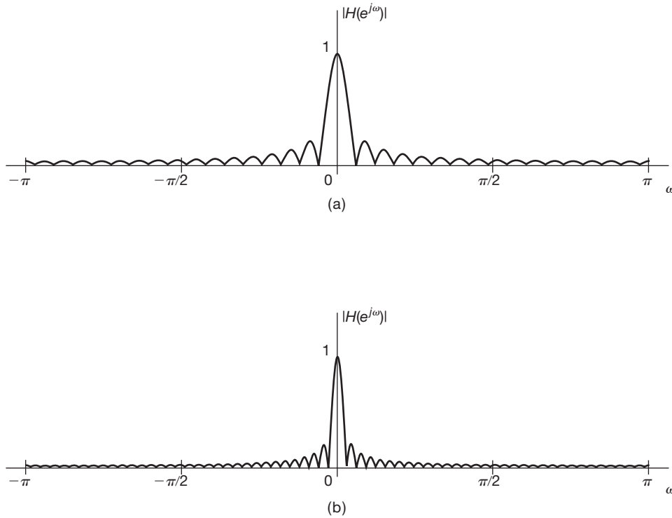
Figura 3.36 Magnitude da resposta em frequência para o filtro de média móvel passa-baixas da Equação 3.162: (a) M = N = 16 ; (b) M = N = 32 .
