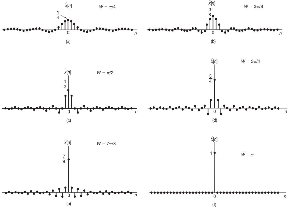
Figura 5.7 Aproximação para a amostra unitária obtida como na Equação 5.16 usando exponenciais complexas com frequências |\omega| \leq W : (a) W = \pi/4 ; (b) W = 3\pi/8 ; (c) W = \pi/2 ; (d) W = 3\pi/4 ; (e) W = 7\pi/8 ; (f) W = \pi . Observe que, para W = \pi , \hat{x}[n] = \delta[n] .
