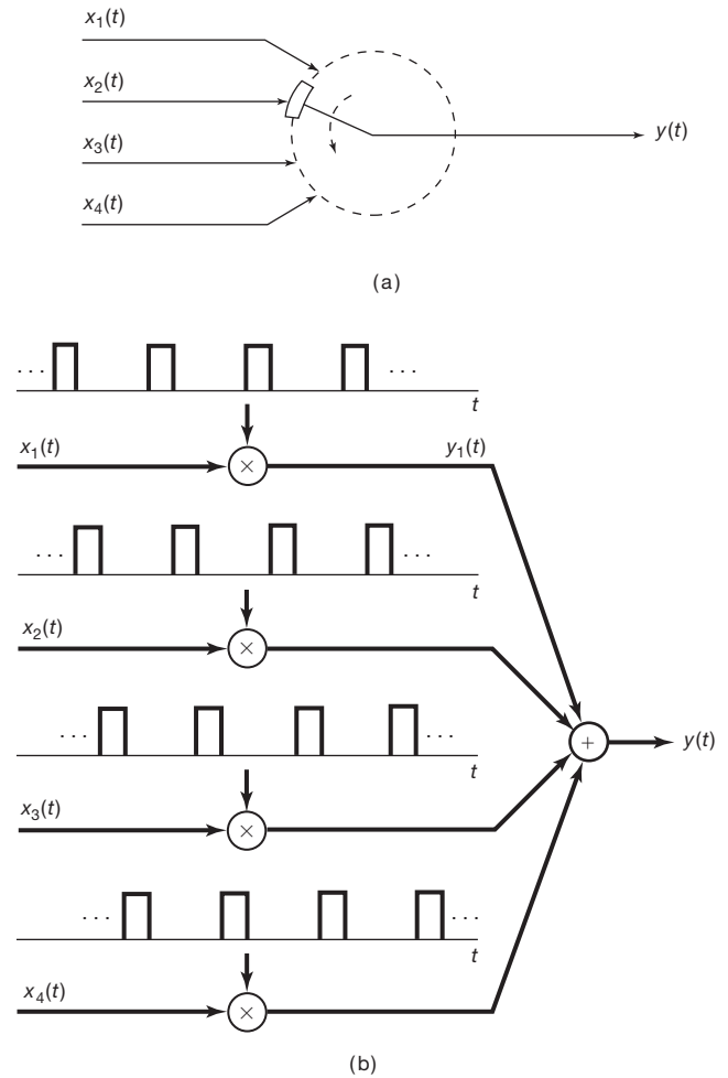
Figura 8.25 Multiplexação por divisão de tempo.
