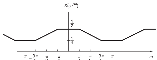
Figura 5.20 Resultado da convolução periódica do Exemplo 5.15.
