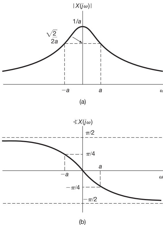
Figura 4.5 Transformada de Fourier do sinal x(t) = e^{-at}u(t) , a > 0 , considerado no Exemplo 4.1.
