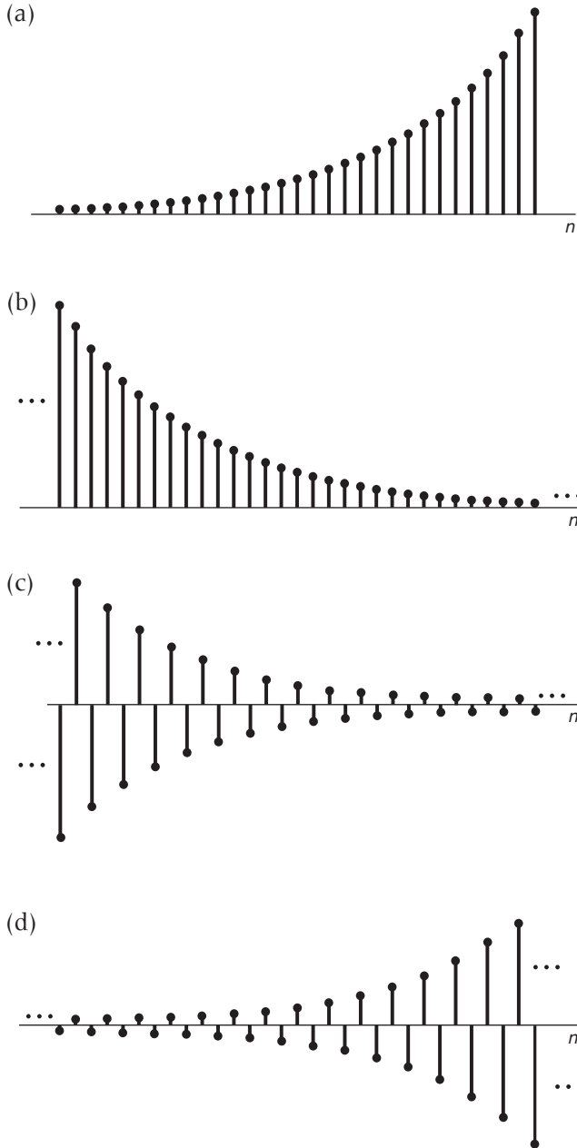
Figura 1.24 Sinal exponencial real x[n] = C\alpha^n : (a) \alpha > 1 ; (b) 0 < \alpha < 1 ; (c) -1 < \alpha < 0 ; (d) \alpha < -1 .
