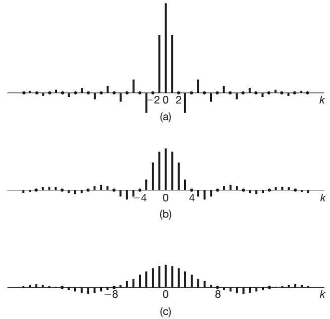
Figura 3.7 Gráficos dos coeficientes Ta_k da série de Fourier para a onda quadrada periódica com T_1 fixo e para diferentes valores de T : (a) T = 4T_1 ; (b) T = 8T_1 ; (c) T = 16T_1 . Os coeficientes são amostras regularmente espaçadas da 'envoltória' dada por (2 \text{sen } \omega T_1)/\omega , o qual o espaçamento entre as amostras, 2\pi/T , diminui quando T aumenta.
