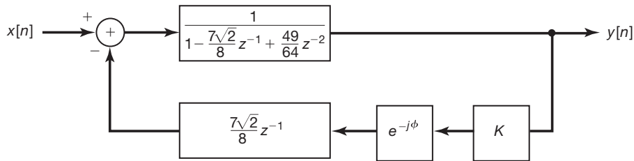
Figura 11.33 Sistema com realimentação de tempo discreto do Exemplo 11.13.
