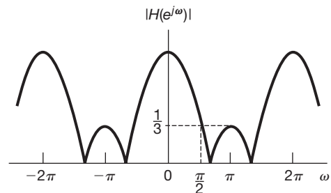
Figura 3.35 Magnitude da resposta em frequência de um filtro passa-baixas de média móvel de três amostras.
