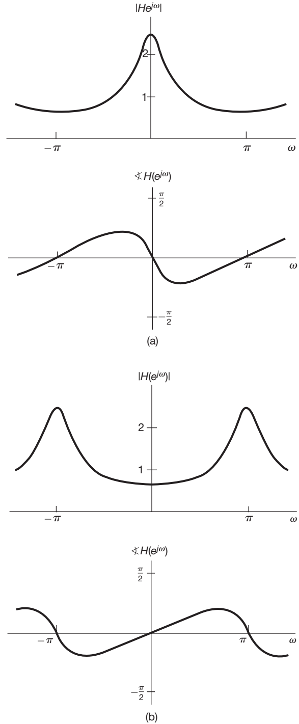
Figura 3.34 Resposta em frequência do filtro de tempo discreto recursivo de primeira ordem da Equação 3.151: (a) a = 0,6 ; (b) a = -0,6 .
