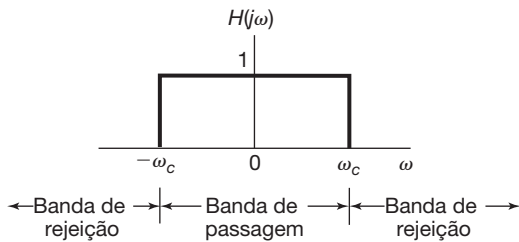
Figura 4.20 Resposta de frequência de um filtro passa-baixas ideal.
