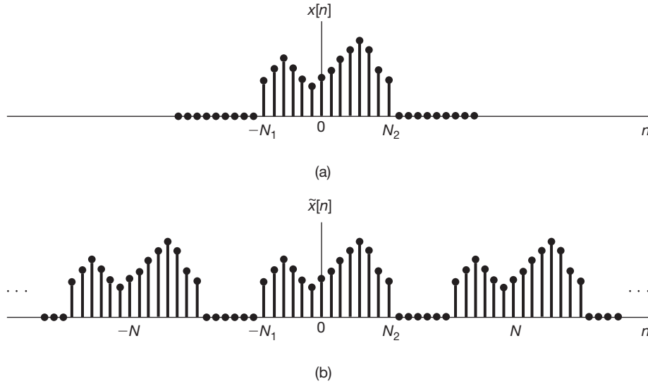
Figura 5.1 (a) Sinal x[n] de duração finita; (b) sinal periódico \tilde{x}[n] construído para ser igual a x[n] por um período.
