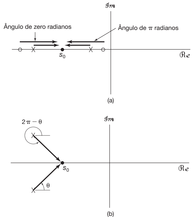
Figura 11.13 (a) Contribuição angular dos polos e zeros reais a um ponto no eixo real. (b) Contribuição angular total de um par de polos complexos conjugados a um ponto no eixo real.
