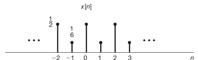
Figura 3.20 Sequência x[n] que é consistente com as propriedades especificadas no Exemplo 3.14.
