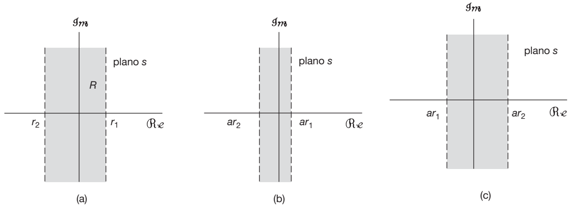
Figura 9.24 Efeito da mudança de escala de tempo sobre a RDC. (a) RDC de X(s) . (b) RDC de (1/|a|)X(s/a) para 0 < a < 1 . (c) RDC de (1/|a|)X(s/a) para 0 > a > -1 .
