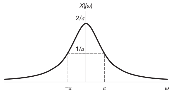
Figura 4.7 Transformada de Fourier do sinal considerado no Exemplo 4.2 e representado na Figura 4.6.
