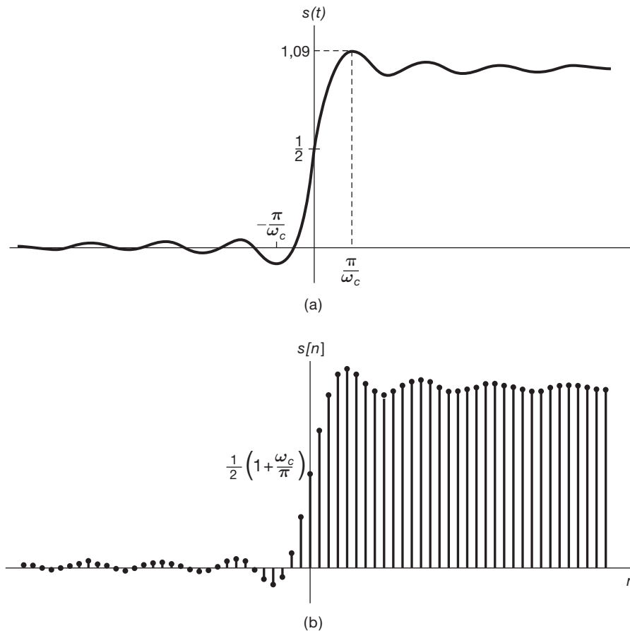
Figura 6.14 (a) Resposta ao degrau de um filtro passa-baixas ideal de tempo contínuo; (b) resposta ao degrau de um filtro passa-baixas ideal de tempo discreto.
