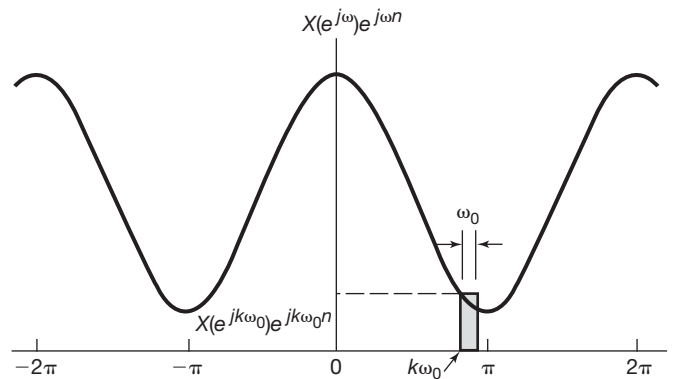
Figura 5.2 Interpretação gráfica da Equação 5.7.
