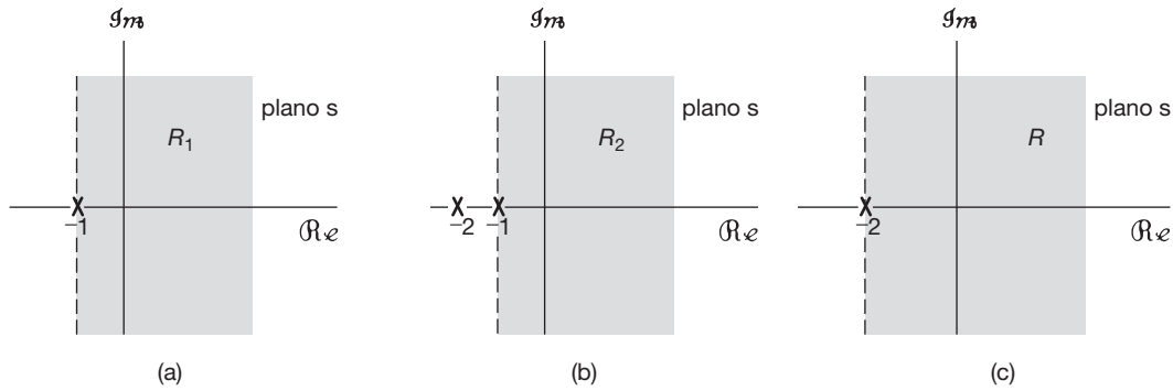
Figura 9.22 Diagramas de polos e zeros e RDCs para o Exemplo 9.13. (a) X_1(s) . (b) X_2(s) . (c) X_1(s) - X_2(s) . A RDC para X_1(s) - X_2(s) inclui a intersecção de R_1 e R_2 que pode então ser estendida para ser delimitada pelo polo em s = -2 .
