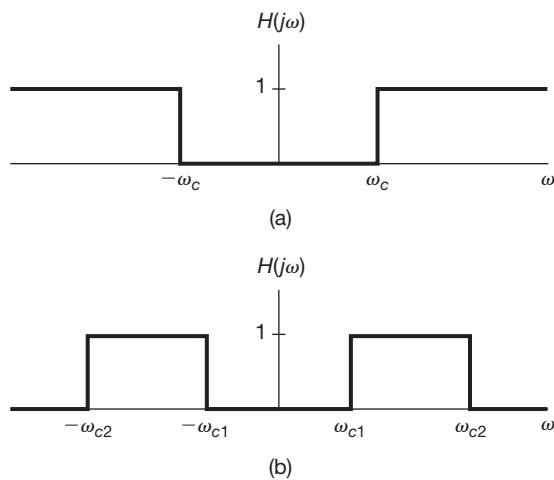
Figura 3.27 (a) Resposta em frequência de um filtro passa-altas ideal; (b) resposta em frequência de um filtro passa-faixa ideal.
