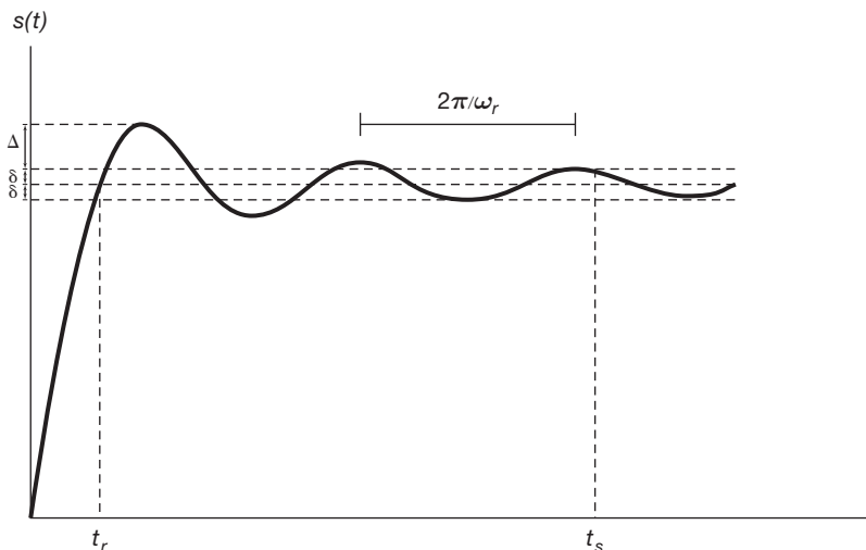
Figura 6.17 Resposta ao degrau de um filtro passa-baixas de tempo contínuo indicando seu tempo de subida t_r , sobressinal \Delta , frequência de oscilação \omega_r e tempo de acomodação t_s , ou seja, o tempo em que a resposta ao degrau permanece dentro de uma faixa \pm\delta de seu valor final.
