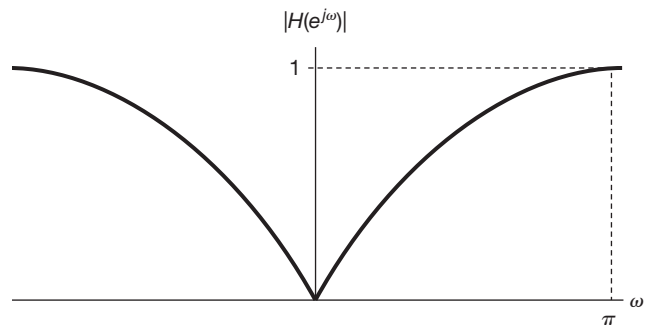
Figura 3.37 Resposta em frequência de um filtro passa-altas simples.
