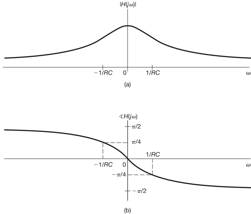
Figura 3.30 Gráficos de (a) magnitude e (b) fase para a resposta em frequência do circuito RC da Figura 3.29 com saída v_c(t) .
