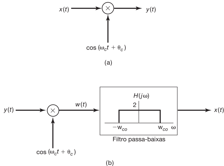
Figura 8.8 Modulação e demodulação em amplitude com uma portadora senoidal: (a) sistema de modulação; (b) sistema de demodulação. A frequência de corte do filtro passa-baixas \omega_{co} é maior que \omega_M e menor que (2\omega_c - \omega_M) .
