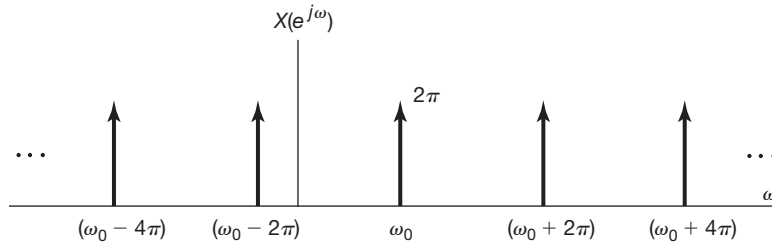
Figura 5.8 Transformada de Fourier de x[n] = e^{j\omega_0 n} .
