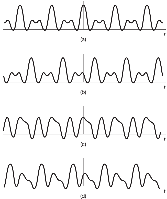
Figura 6.1 O sinal x(t) dado na Equação 6.3 para diversas escolhas diferentes dos ângulos de fase \phi_1 , \phi_2 e \phi_3 : (a) \phi_1 = \phi_2 = \phi_3 = 0 ; (b) \phi_1 = 4 rad, \phi_2 = 8 rad, \phi_3 = 12 rad; (c) \phi_1 = 6 rad, \phi_2 = -2,7 rad, \phi_3 = 0,93 rad; (d) \phi_1 = 1,2 rad, \phi_2 = 4,1 rad, \phi_3 = -7,02 rad.
