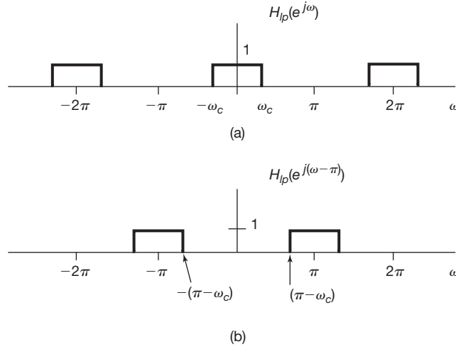
Figura 5.12 (a) Resposta em frequência de um filtro passa-baixas; (b) resposta em frequência de um filtro passa-altas obtido pelo deslocamento da resposta em frequência em (a) por \omega = \pi , correspondendo a meio período.
