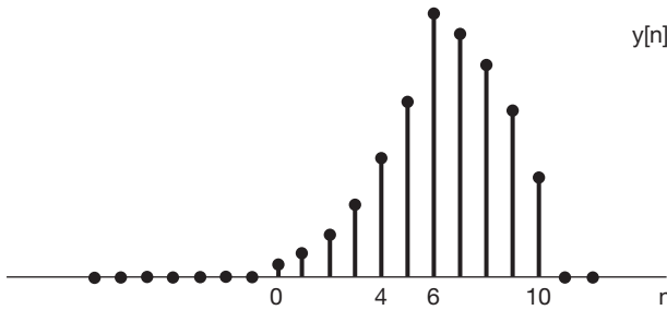
Figura 2.10 Resultado da convolução do Exemplo 2.4.
