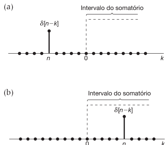
Figura 1.31 Relação dada na Equação 1.67: (a) n < 0 ; (b) n > 0 .
