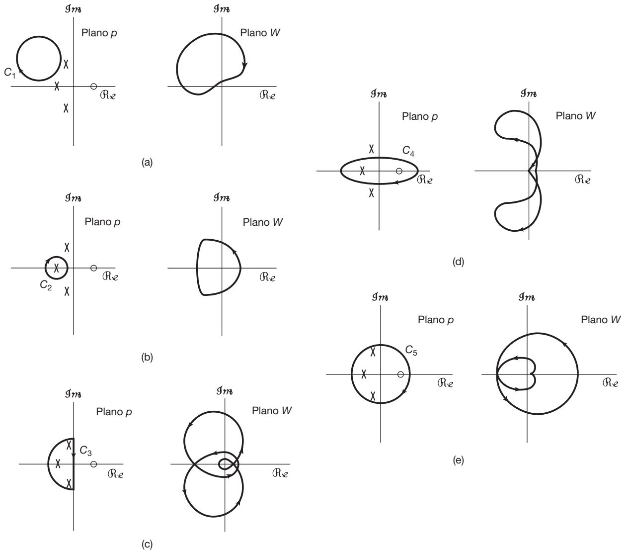
Figura 11.18 Propriedade de mapeamento básica para o Exemplo 11.4: (a) o contorno não circunda polos ou zeros e, conseqüentemente, W(p) não tem circundações da origem; (b) o contorno circunda um polo e, logo, W(p) possui uma circundação da origem; (c) o contorno circunda três polos e, portanto, W(p) tem três circundações da origem; (d) o contorno circunda um polo e um zero e, dessa forma, W(p) não apresenta circundações da origem; (e) o contorno circunda três polos e um zero. W(p) possui duas circundações da origem.
