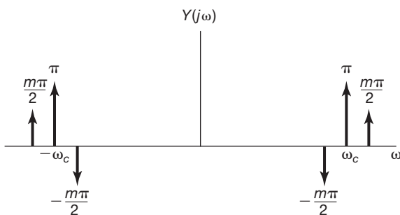
Figura 8.33 Espectro aproximado para FM de banda estreita.
