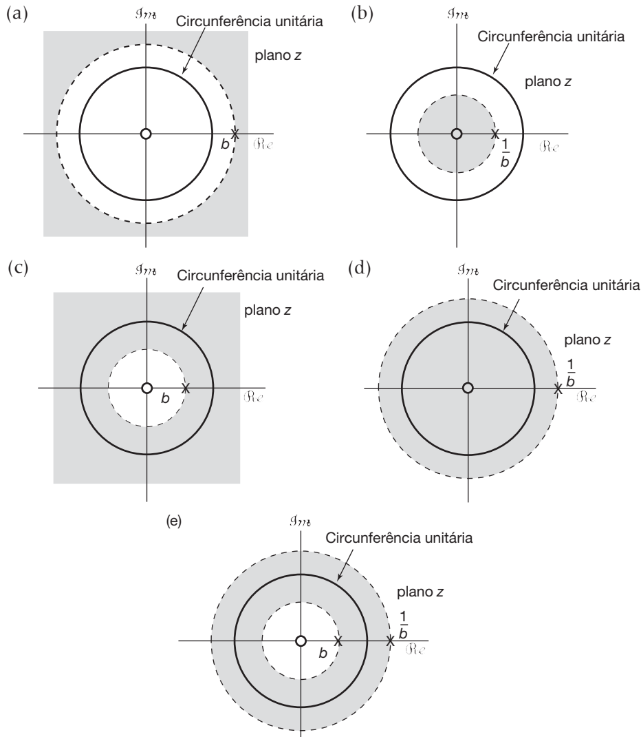
Figura 10.11 Diagramas de polos e zeros e RDCs para o Exemplo 10.7: (a) Equação 10.33, para b > 1 ; (b) Equação 10.34 para b > 1 ; (c) Equação 10.33 para 0 < b < 1 ; (d) Equação 10.34 para 0 < b < 1 ; (e) diagrama de polos e zeros e RDC para Equação 10.36 com 0 < b < 1 . Para b > 1 , a transformada z de x[n] na Equação 10.31 não converge para nenhum valor de z .
