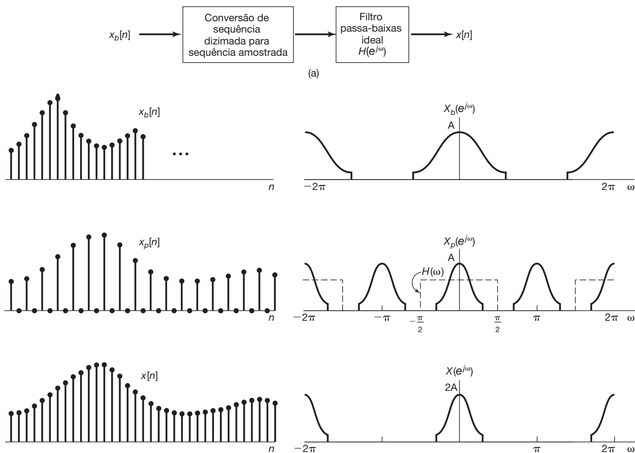
Figura 7.37 Sobreamostragem: (a) sistema total; (b) sequências associadas e espectros para sobreamostragem por um fator de 2.
