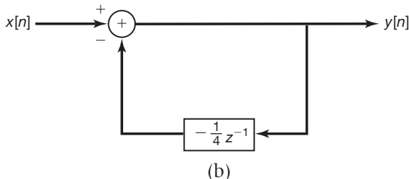
Figura 10.18 (a) Representações por diagrama de blocos do sistema LIT causal do Exemplo 10.28; (b) representação de diagrama em blocos equivalente.
