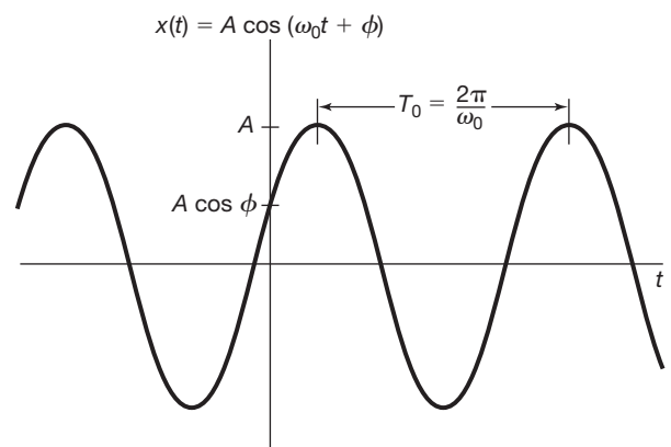
Figura 1.20 Sinal senoidal de tempo contínuo.
