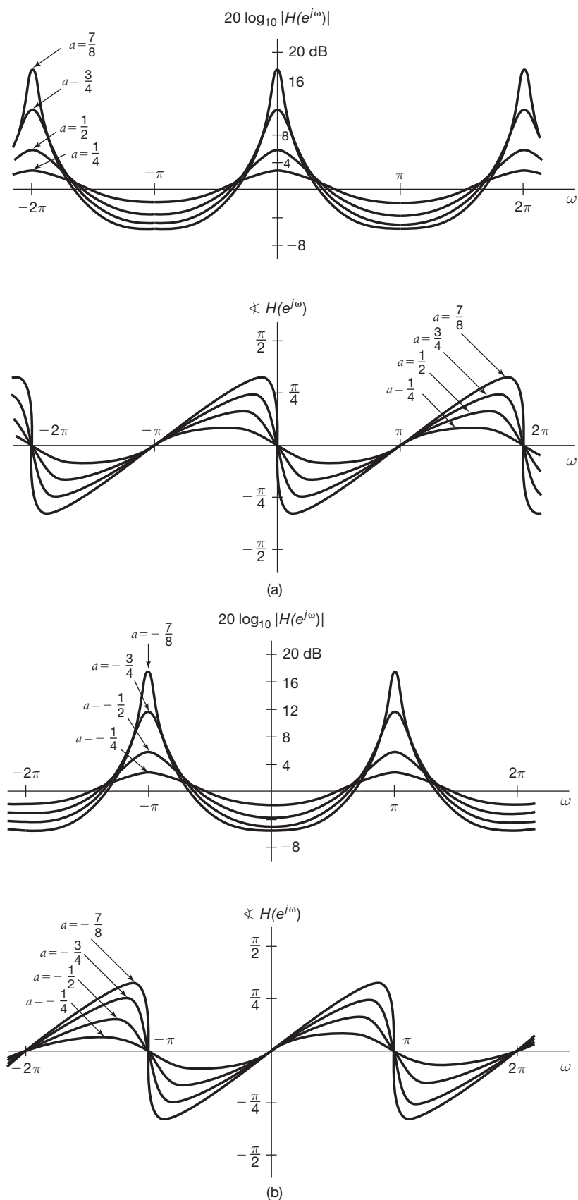
Figura 6.28 Magnitude e fase da resposta em frequência da Equação 6.52 para um sistema de primeira ordem: (a) gráficos para diferentes valores de a > 0 ; (b) gráficos para diferentes valores de a < 0 .
