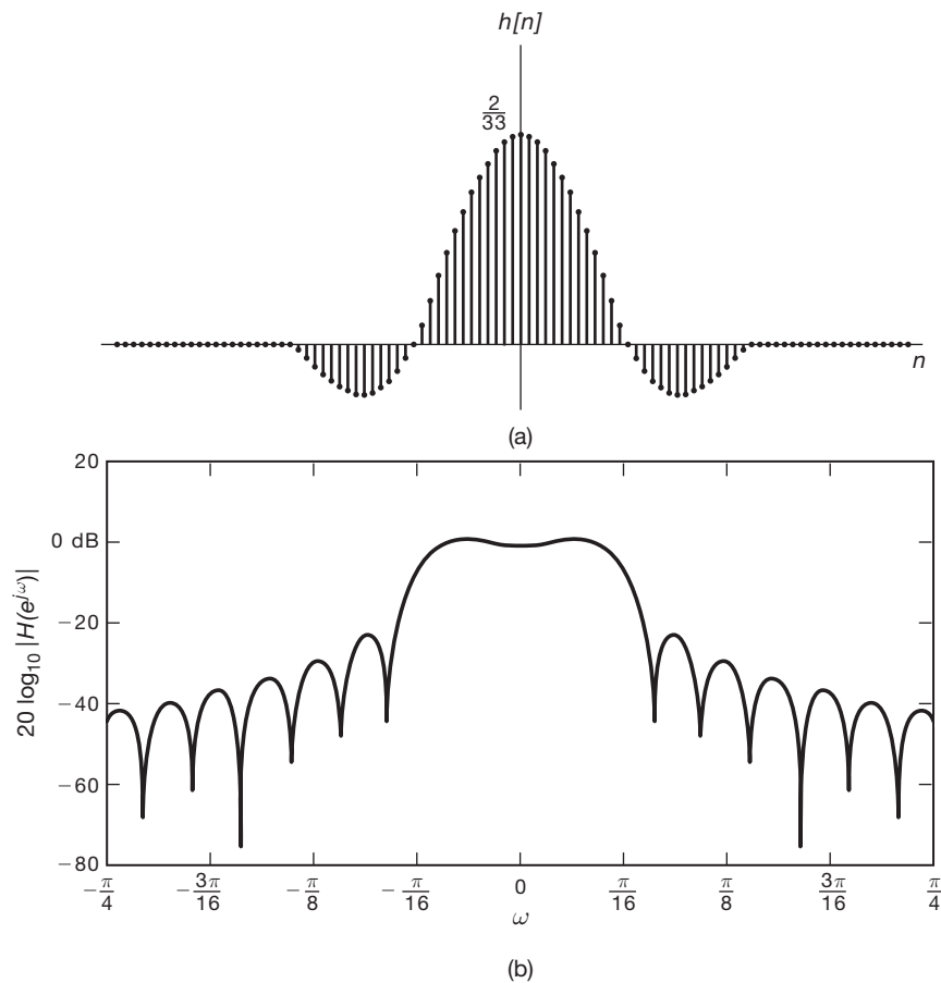
Figura 6.37 (a) Resposta ao impulso para o filtro não recursivo da Equação 6.82; (b) magnitude logarítmica de resposta em frequência do filtro.
