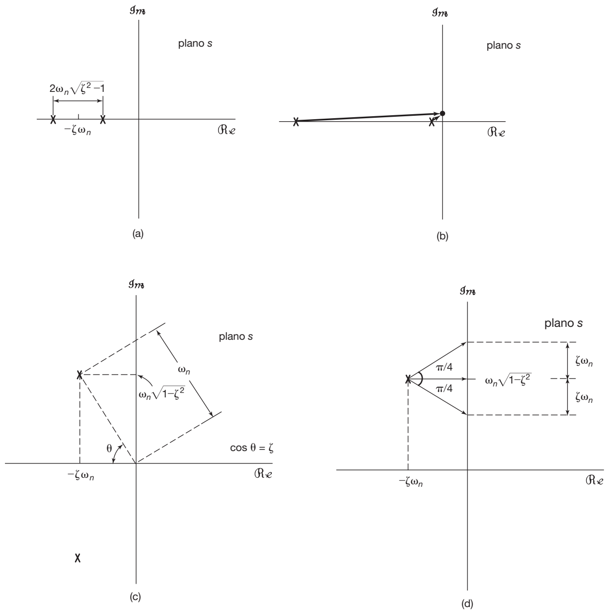
Figura 9.19 (a) Diagrama de polos e zeros para um sistema de segunda ordem com \zeta > 1 . (b) Vetores polos para \zeta \gg 1 . (c) Diagrama de polos e zeros para um sistema de segunda ordem com 0 < \zeta < 1 . (d) Vetores polos para 0 < \zeta < 1 e para \omega = \omega_n\sqrt{1-\zeta^2} e \omega = \omega_n\sqrt{1-\zeta^2} \pm j\zeta\omega_n .
