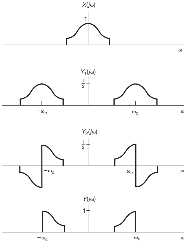
Figura 8.22 Espectros associados ao sistema de banda lateral única da Figura 8.21.
