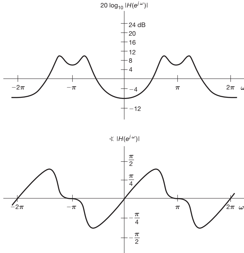
Figura 6.9 Representações gráficas típicas da magnitude e fase de uma resposta em frequência de tempo discreto H(e^{j\omega}) .
