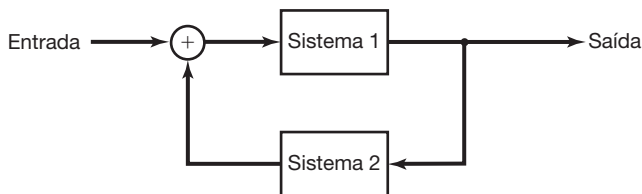
Figura 1.43 Interconexão com realimentação.
