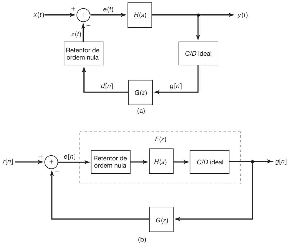
Figura 11.6 (a) Sistema com realimentação de dados amostrados usando um retentor de ordem nula. (b) Sistema em tempo discreto equivalente.
