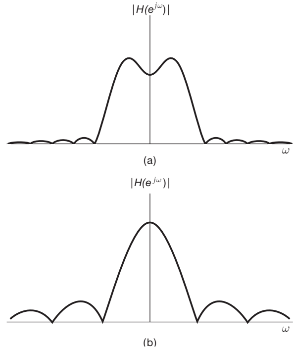
Figura 6.38 Comparação, em uma escala de amplitude linear, das respostas em frequência de (a) Figura 6.37 e (b) Figura 6.35.
