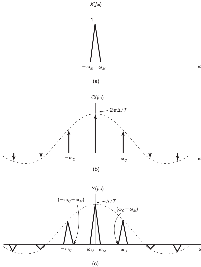
Figura 8.24 Espectros associados à modulação em amplitude de um trem de pulsos. (a) Espectro de um sinal de banda limitada x(t) . (b) Espectro do sinal da portadora de pulso c(t) na Figura 8.23. (c) Espectro do trem de pulsos modulado y(t) .
