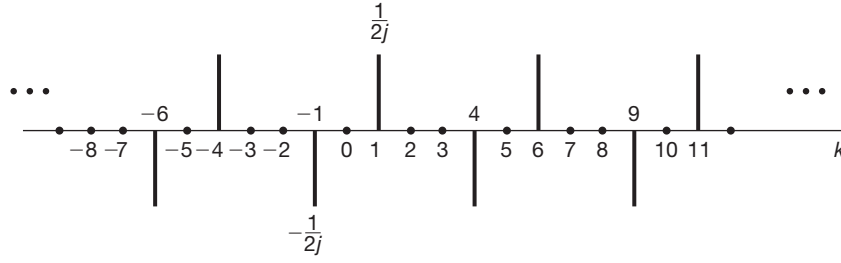
Figura 3.13 Coeficientes de Fourier para x[n] = \text{sen}(2\pi/5)n .
