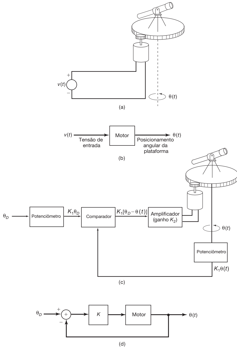
Figura 11.1 Uso de realimentação para controlar o posicionamento angular de um telescópio: (a) plataforma de telescópio controlada por motor dc; (b) diagrama de blocos do sistema em (a); (c) sistema de realimentação para o direcionamento do telescópio; (d) diagrama de blocos do sistema em (c) (aqui, K = K_1 K_2 ).
