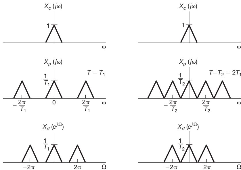
Figura 7.22 Relação entre X_c(j\omega) , X_p(j\omega) e X_d(e^{j\Omega}) para duas taxas de amostragem diferentes.
