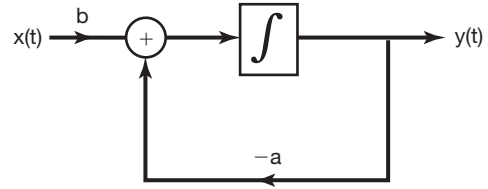
Figura 2.32 Representação em diagrama de blocos do sistema das equações 2.128 e 2.131 usando somadores, multiplicações por coeficientes e integradores.
