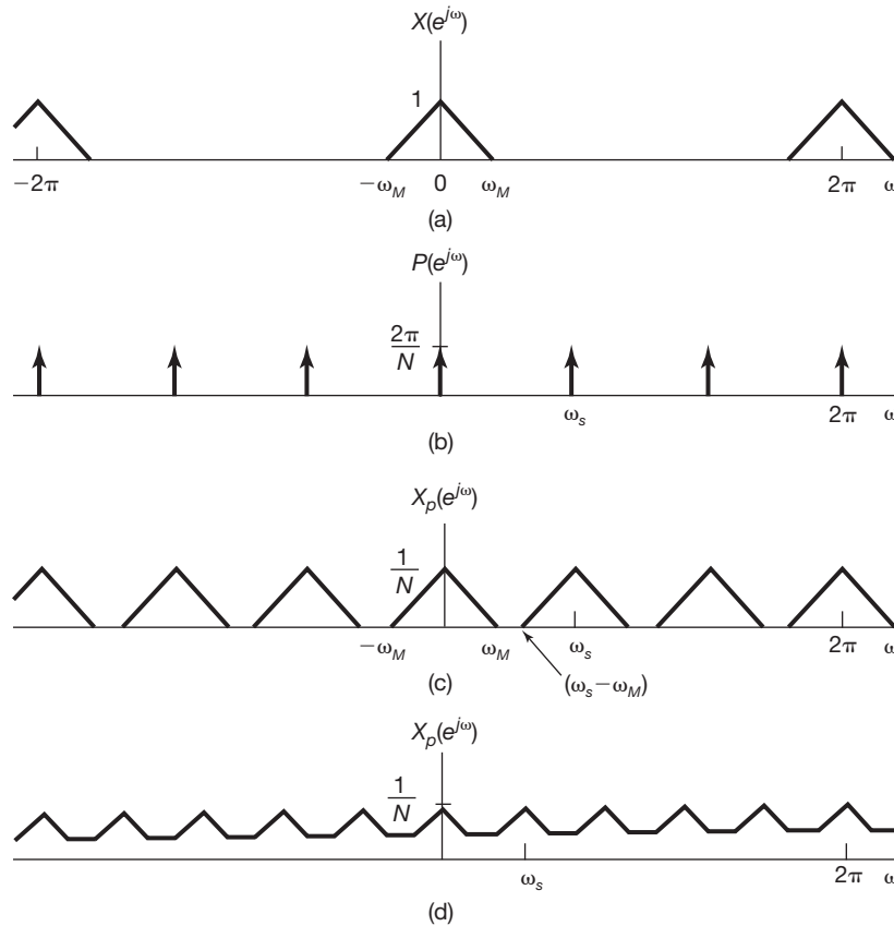
Figura 7.32 Efeito no domínio de frequência da amostragem por trem de impulsos de um sinal de tempo discreto: (a) espectro do sinal original; (b) espectro da sequência de amostragem; (c) espectro do sinal amostrado com \omega_s > 2\omega_M ; (d) espectro do sinal amostrado com \omega_s < 2\omega_M . Observe que ocorre aliasing .
