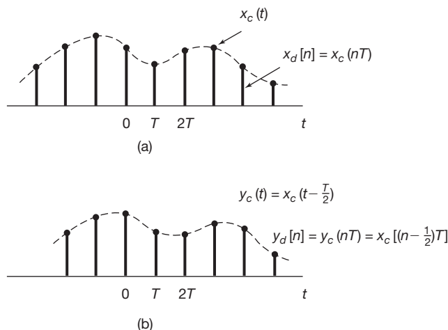
Figura 7.30 (a) Sequência de amostras de um sinal de tempo contínuo x_c(t) . (b) Sequência de (a) com um atraso de meia amostra.
