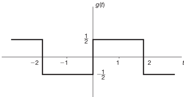
Figura 3.10 Sinal periódico do Exemplo 3.6.
