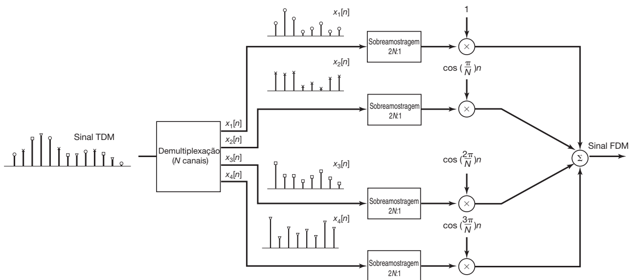
Figura 8.44 Diagrama em blocos para transmultiplexação TDM-para-FDM.
