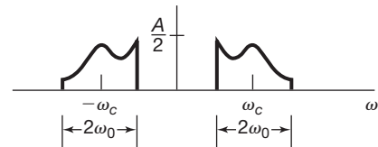
Figura 4.29 Espectro de \Re\{f(t)\} associado à Figura 4.26.
