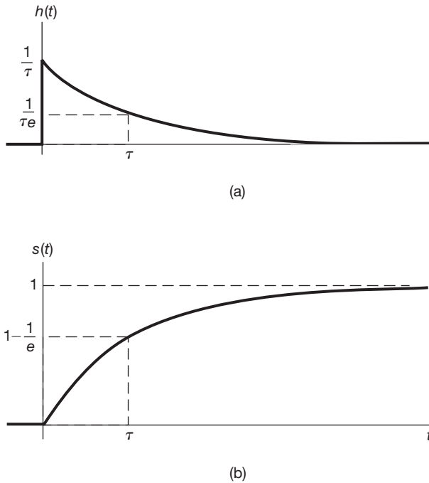
Figura 3.31 (a) Resposta ao impulso do filtro passa-baixas RC de primeira ordem com \tau = RC ; (b) resposta ao degrau do filtro passa-baixas RC com \tau = RC .
