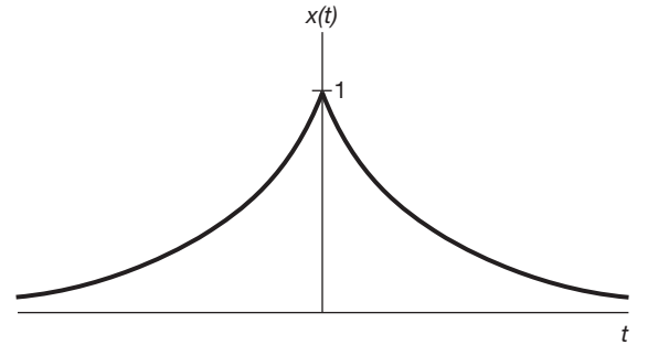
Figura 4.6 Sinal x(t) = e^{-a|t|} do Exemplo 4.2.
